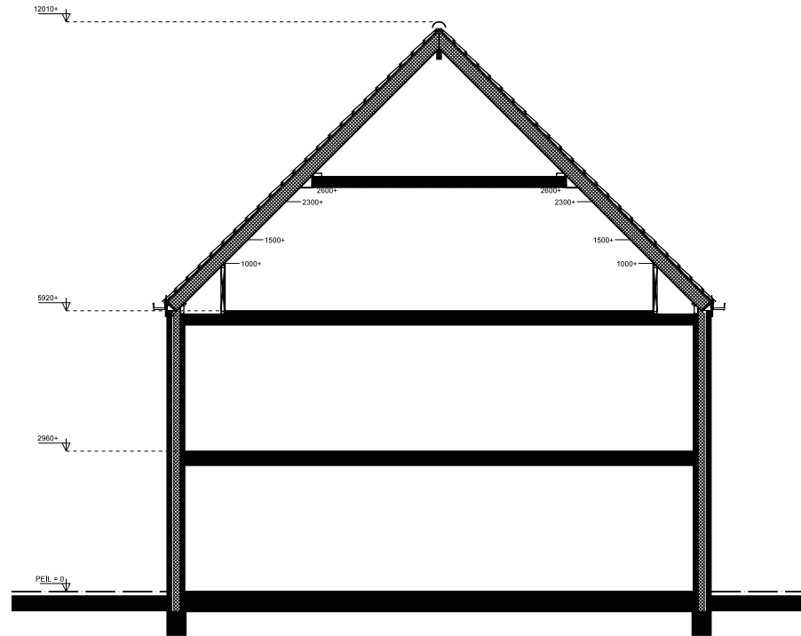
DOORSNEDE type D1
