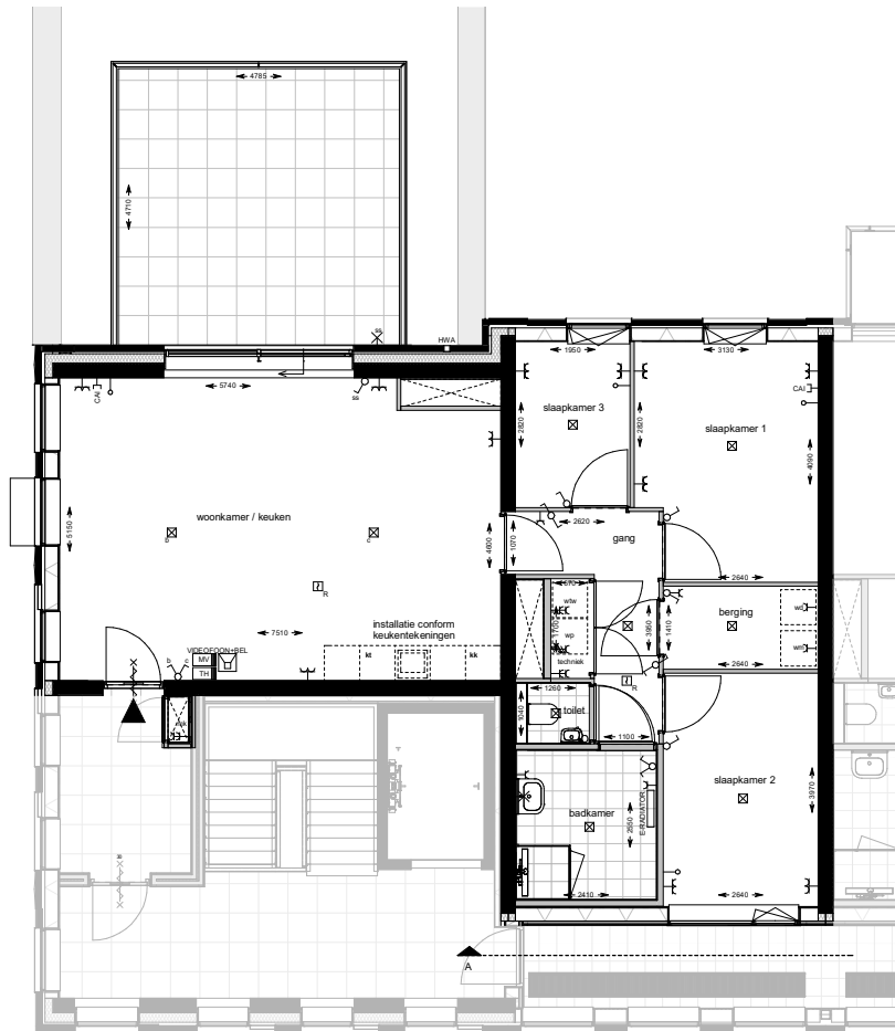
vijfde verdieping 1 : 50
