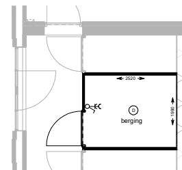
begane grond 1 : 50
