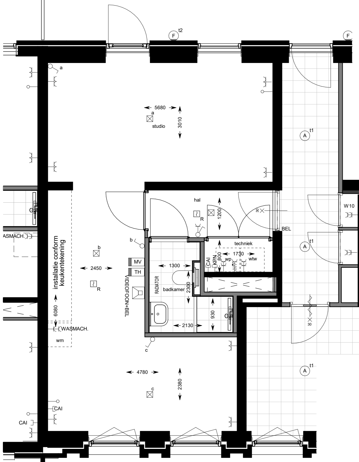
eerste verdieping
