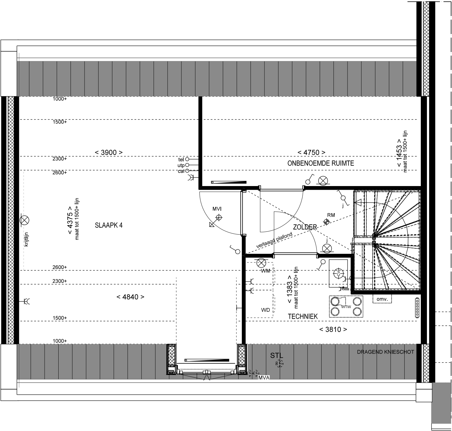
2e VERDIEPING
