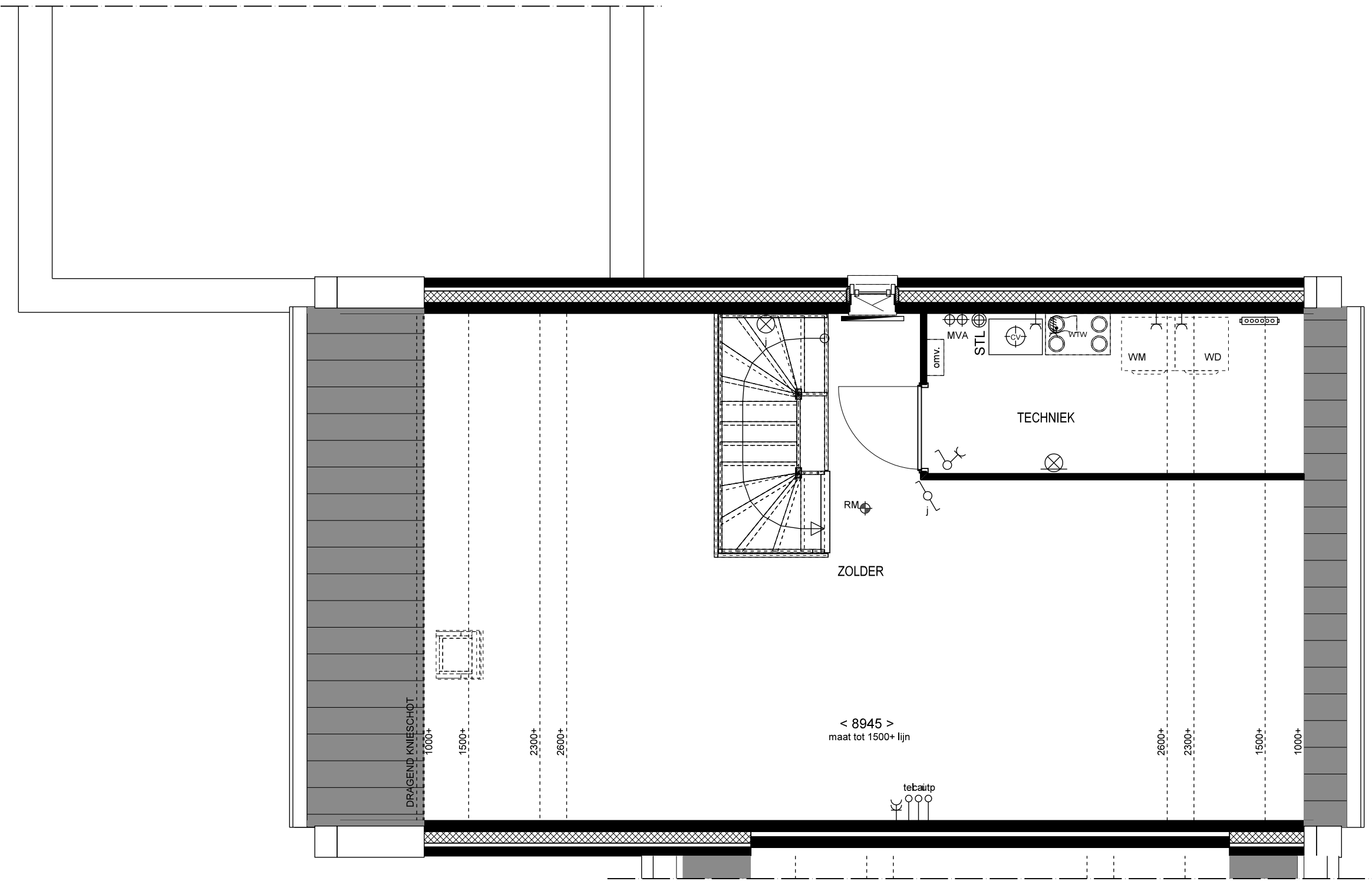
2e VERDIEPING
