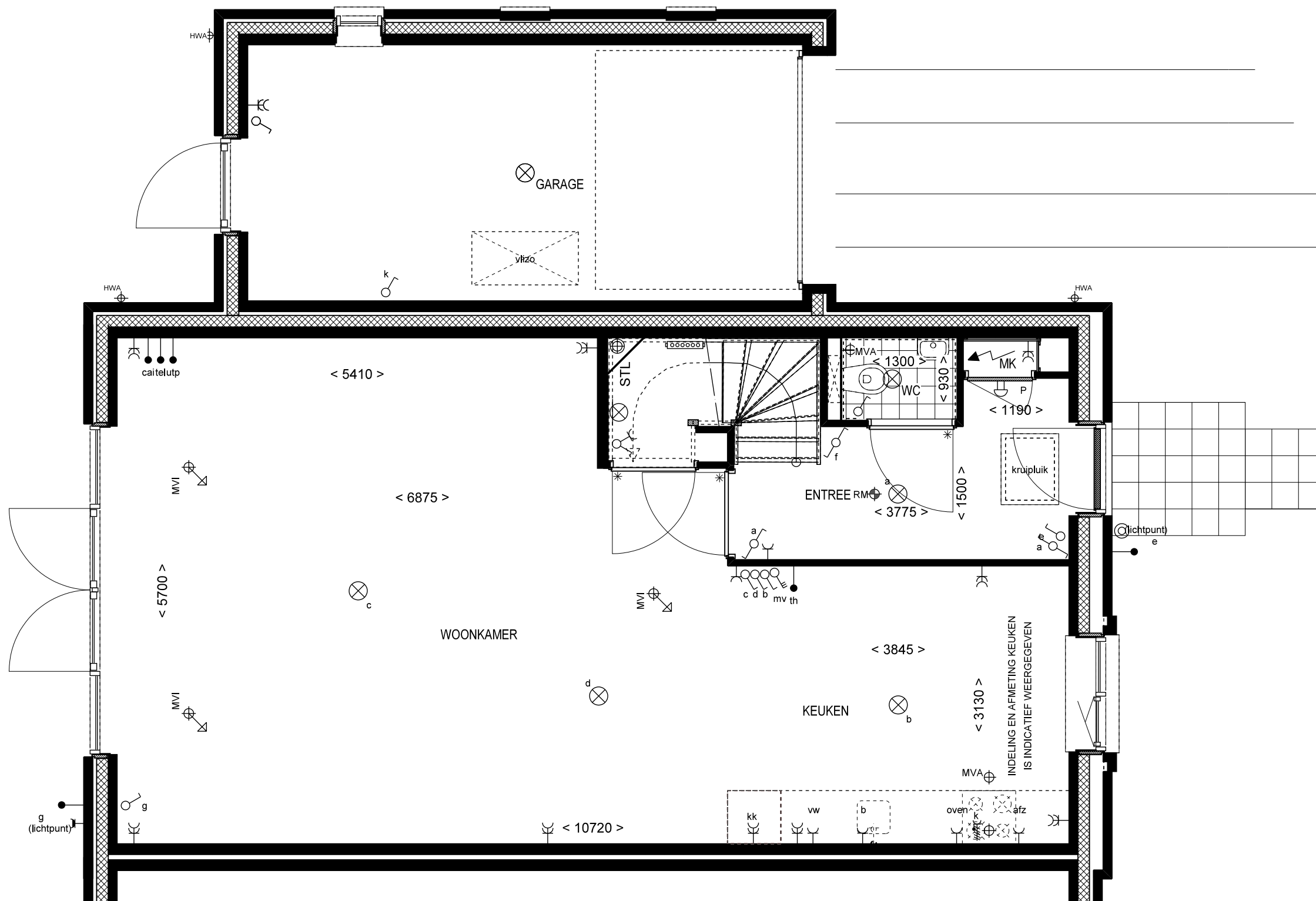
BEGANE GROND
