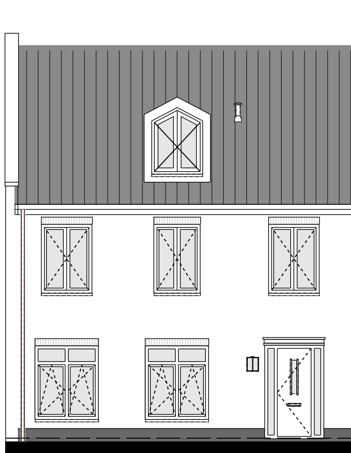
VOORGEVEL
