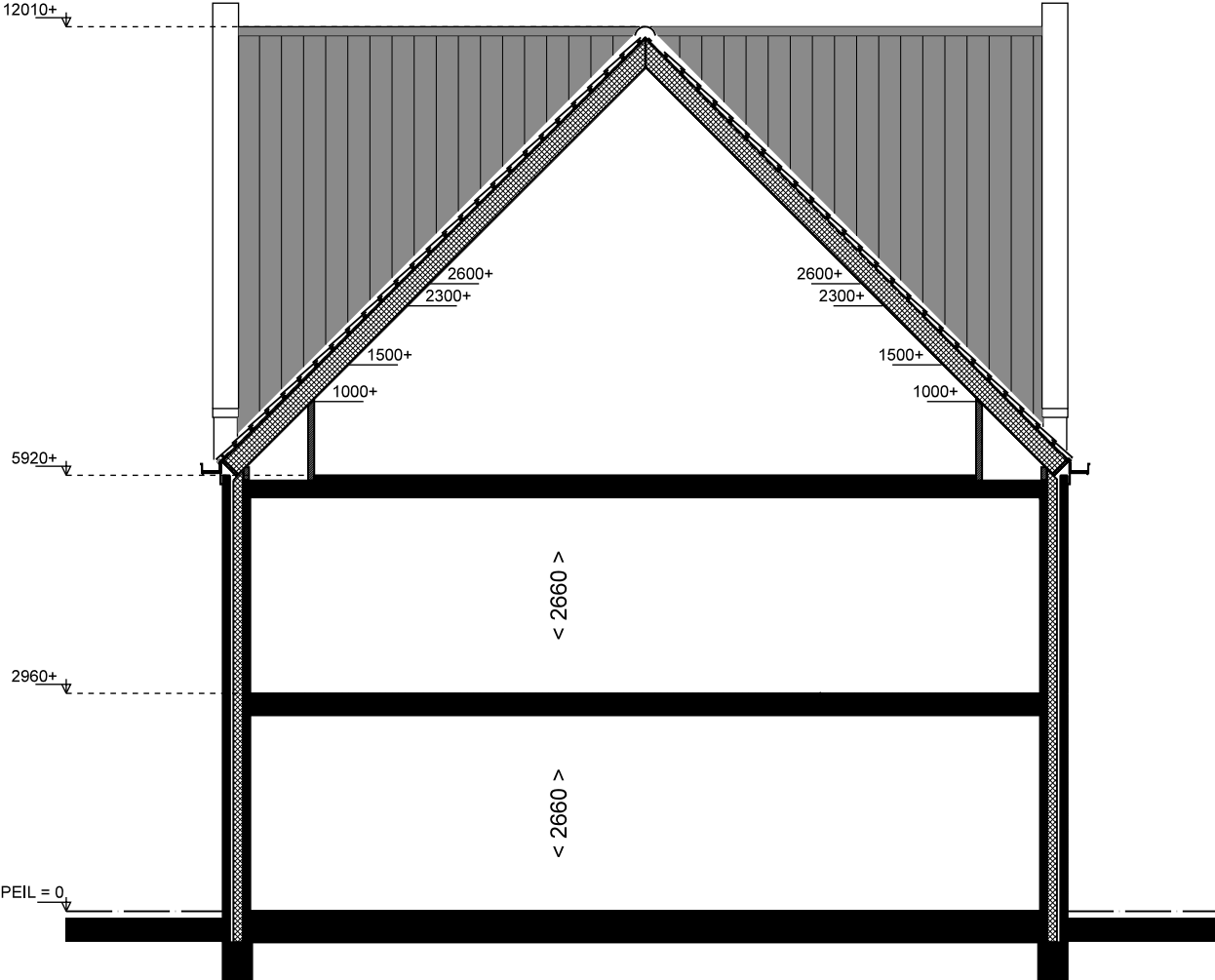
DOORSNEDE
