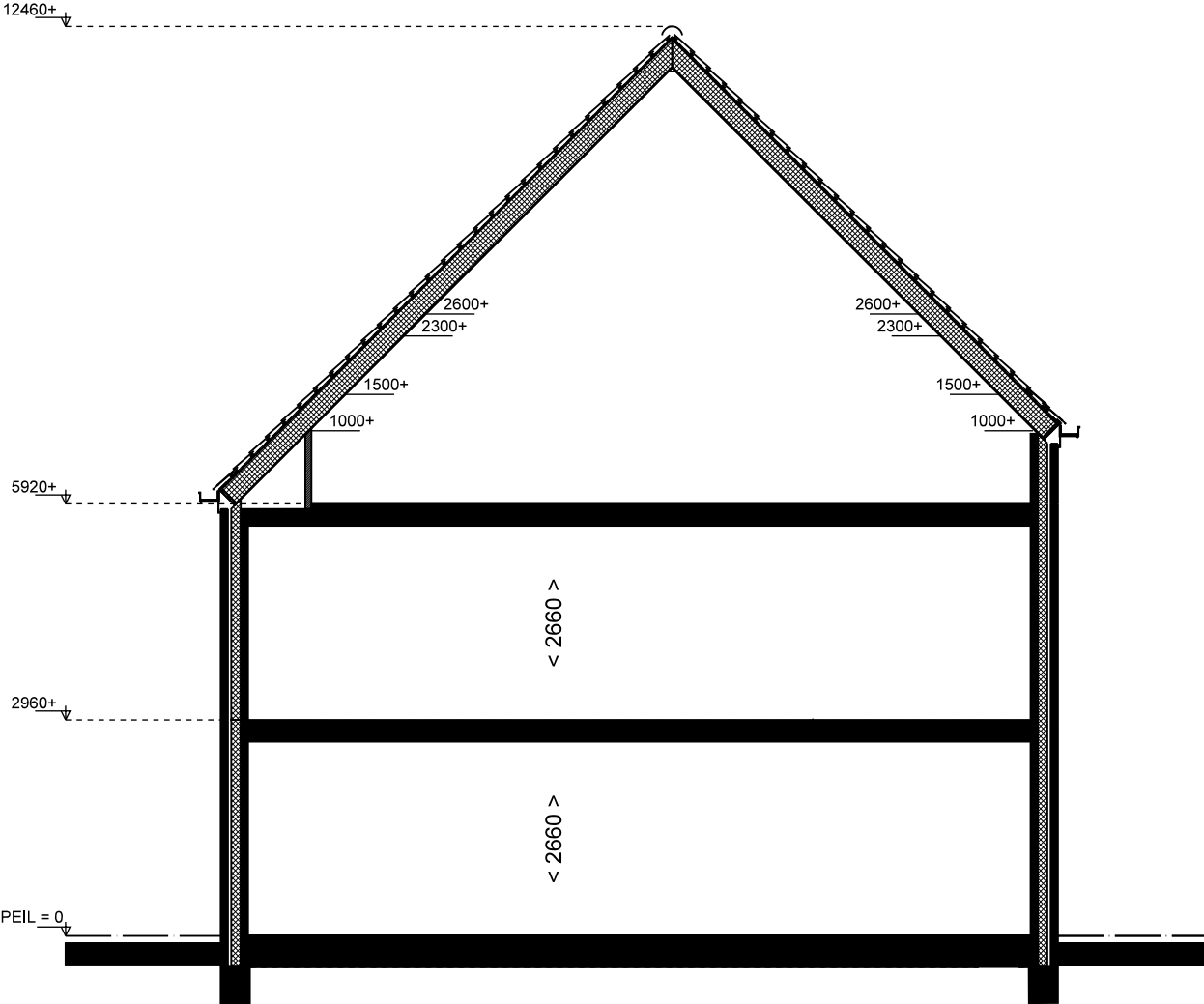
DOORSNEDE
