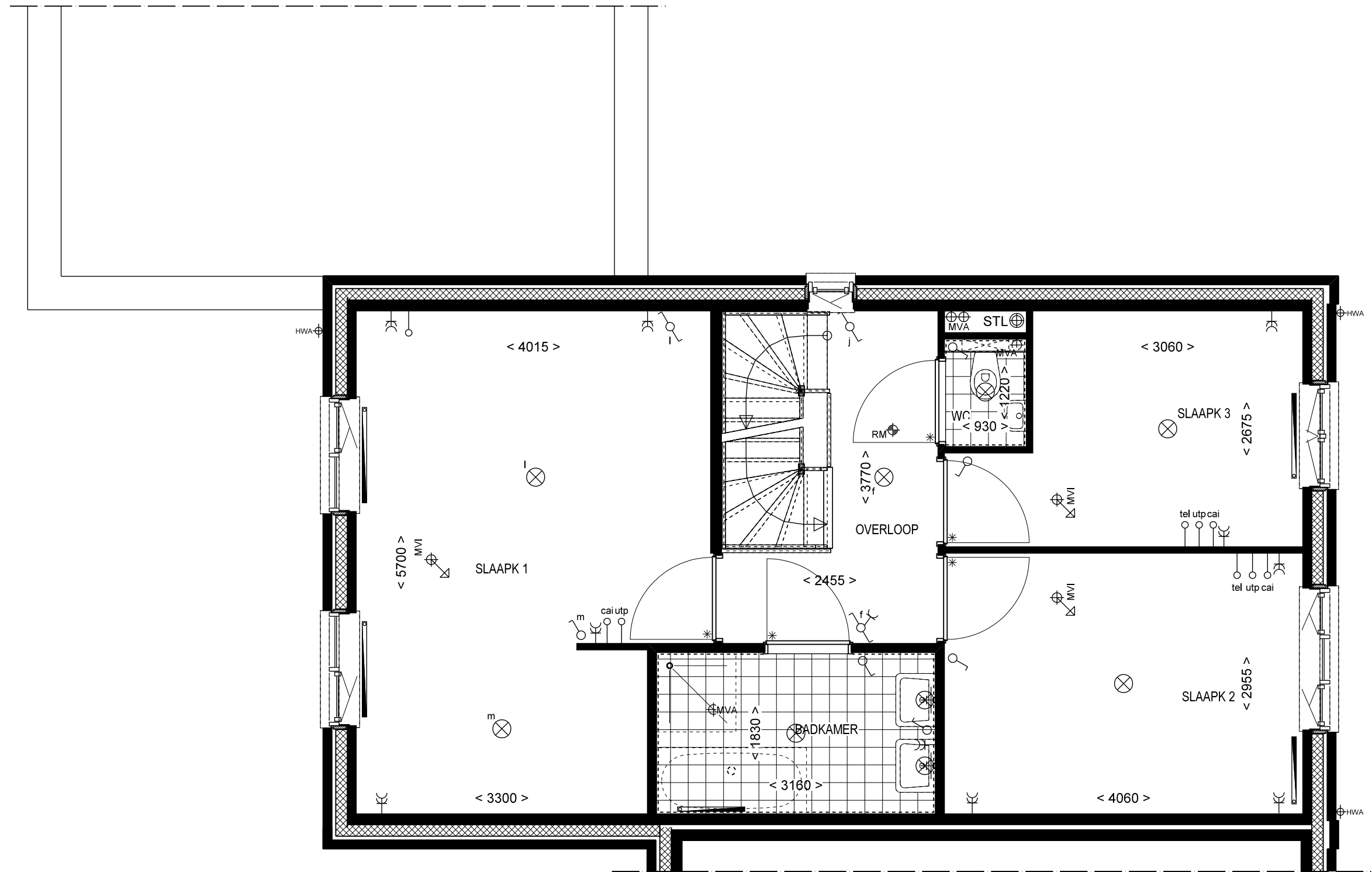
1e VERDIEPING
