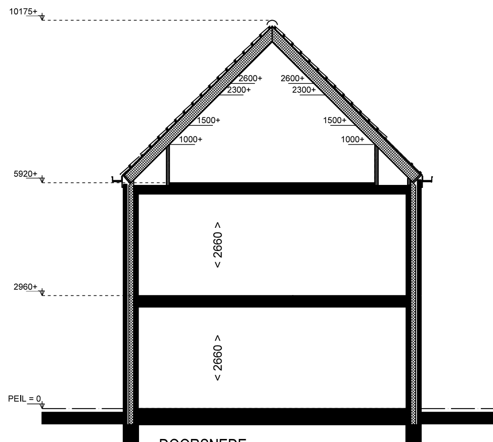
DOORSNEDE
