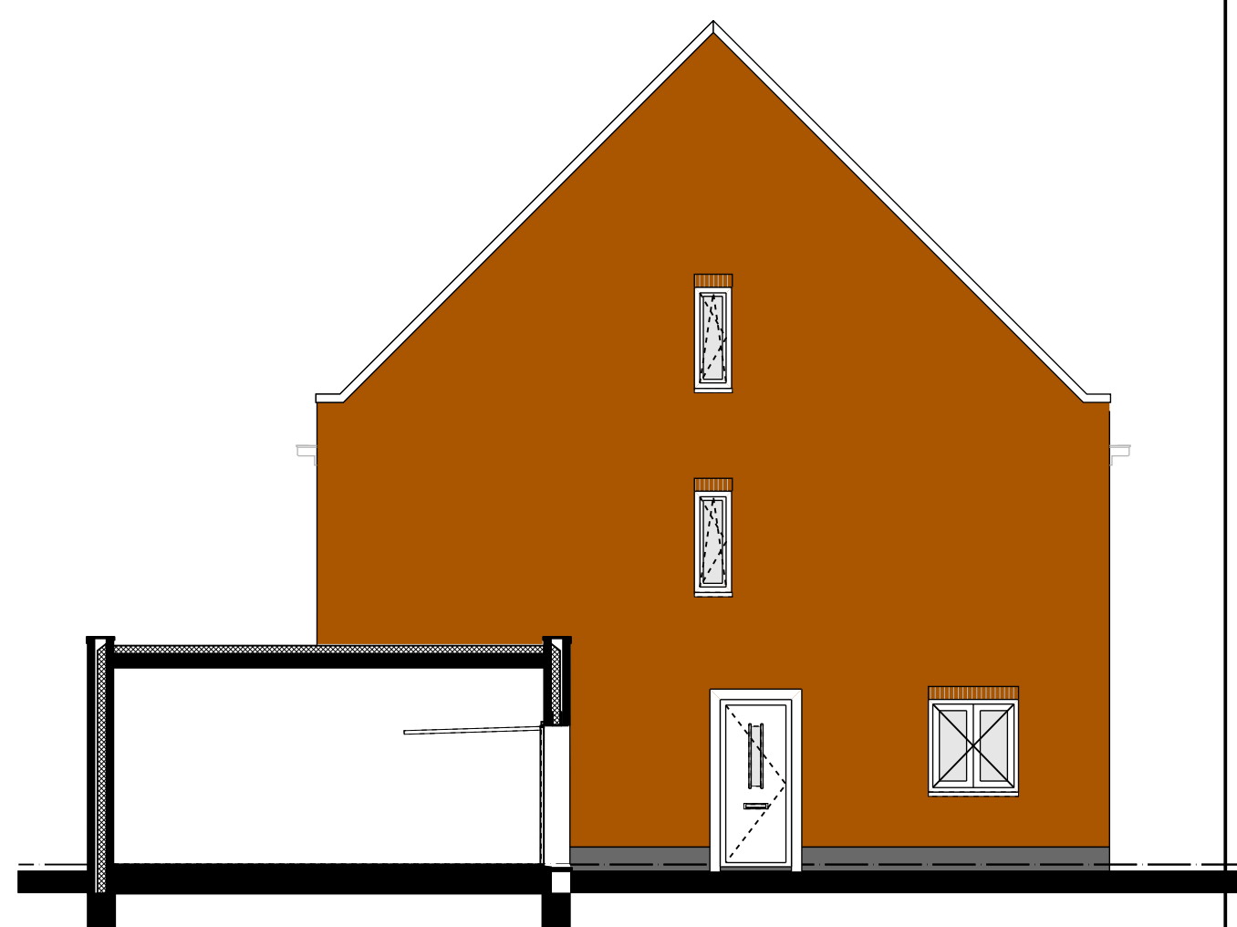
ZIJGEVEL
