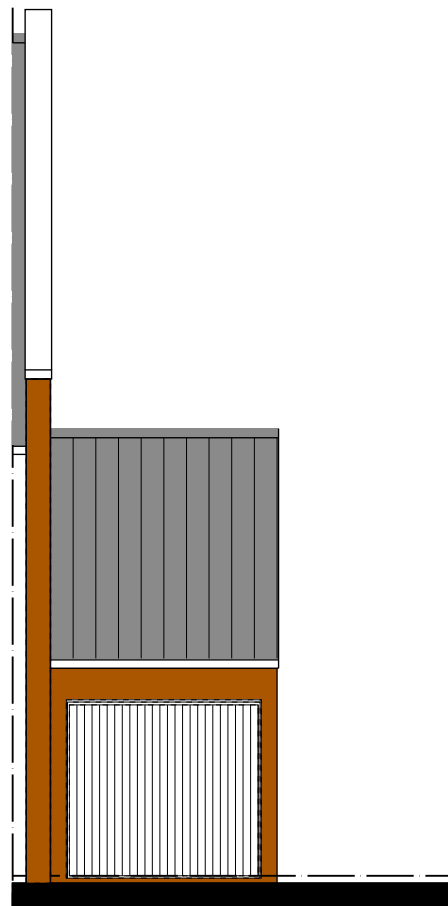
VOORGEVEL
