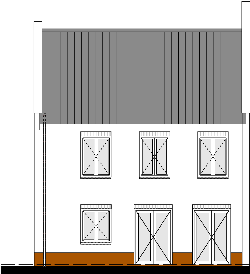
ACHTERGEVEL
