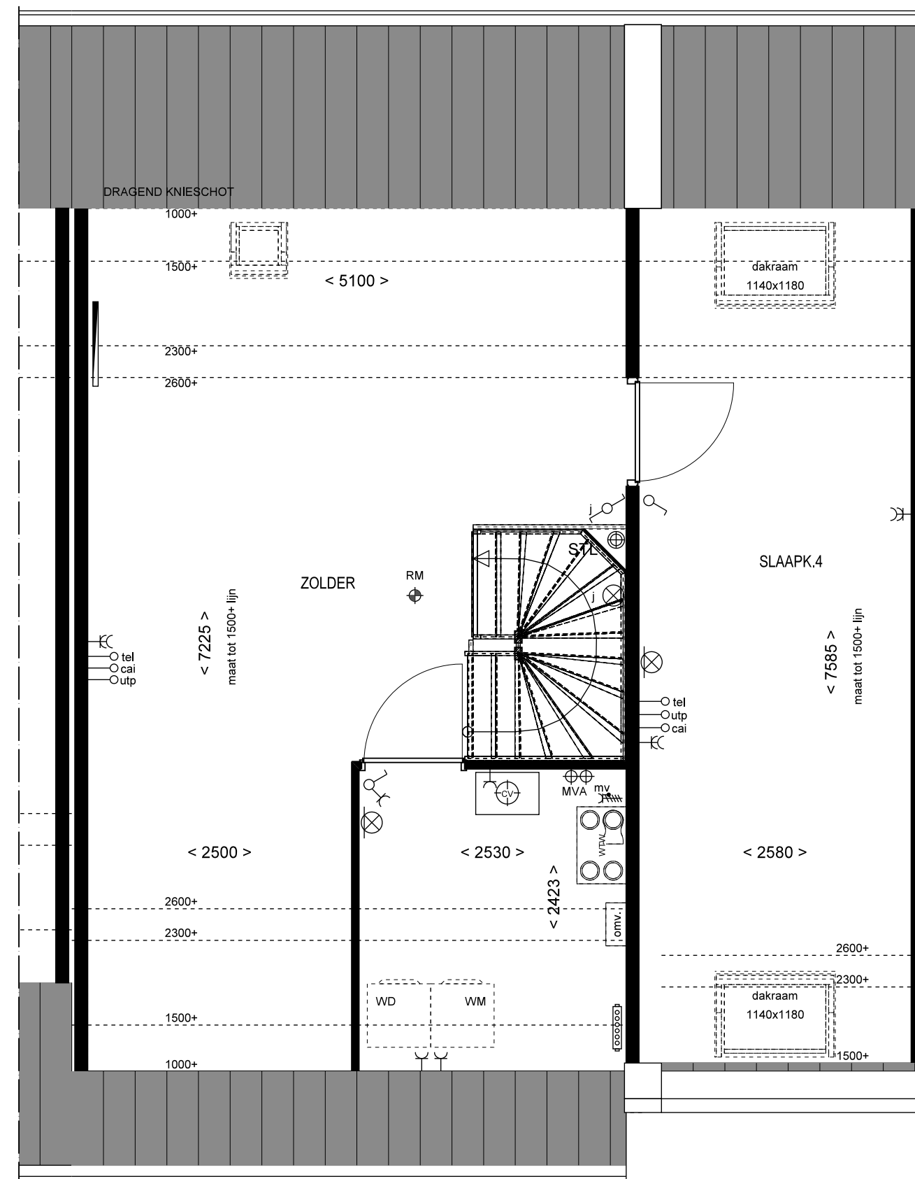
2e VERDIEPING
