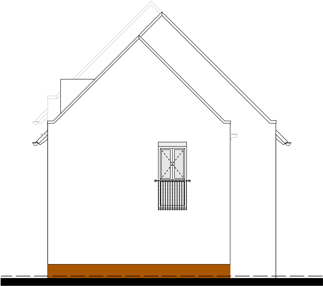
ZIJGEVEL
