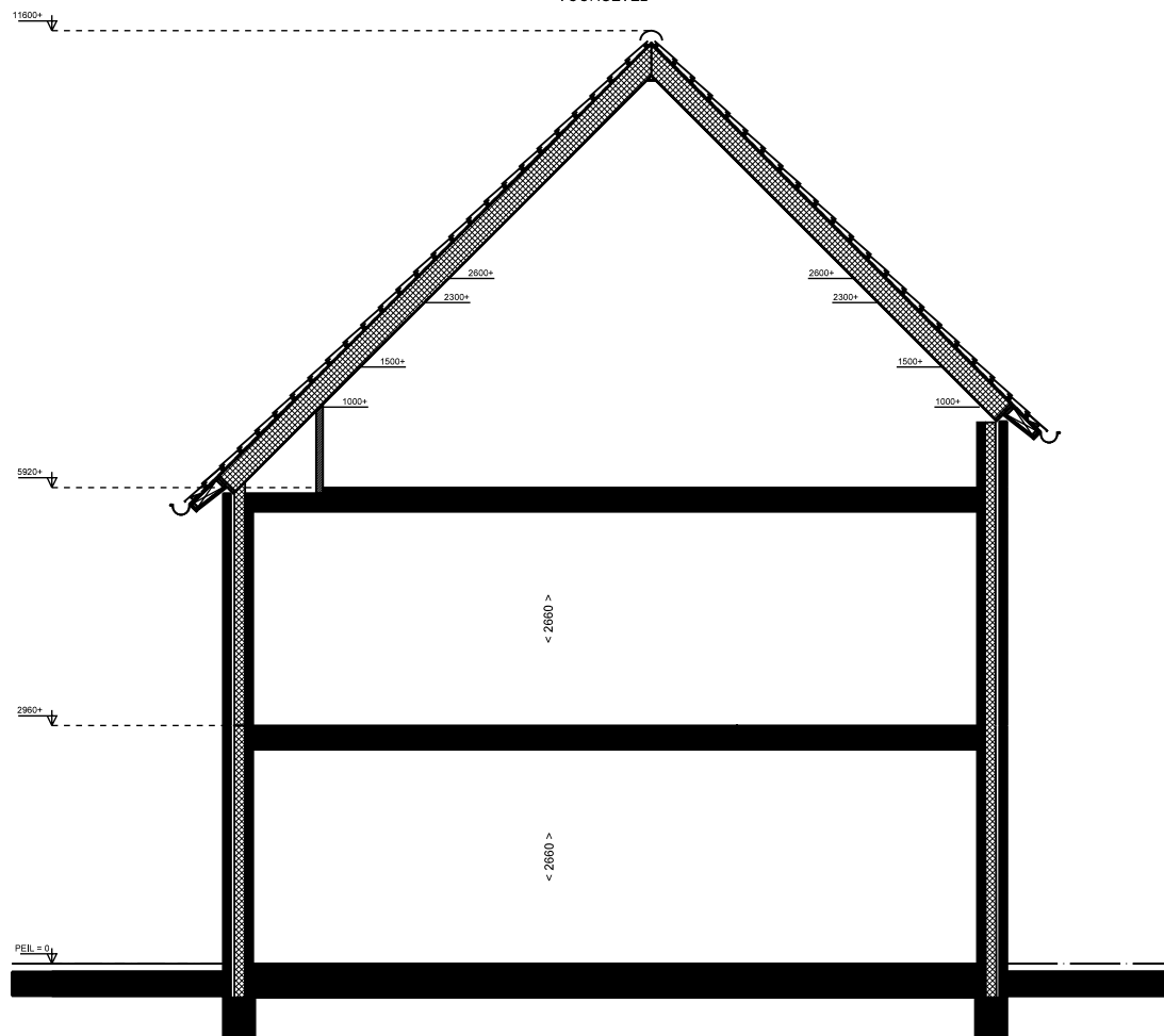
DOORSNEDE
