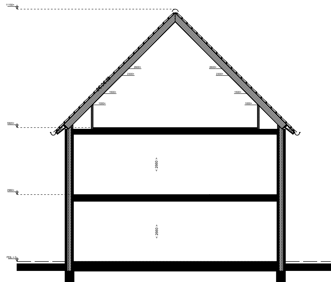
DOORSNEDE
