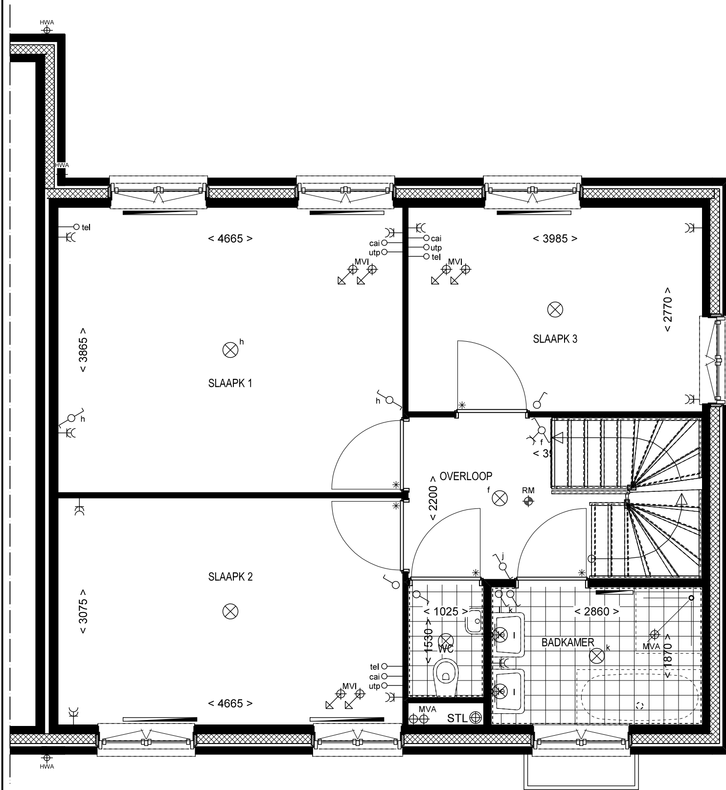
1e VERDIEPING
