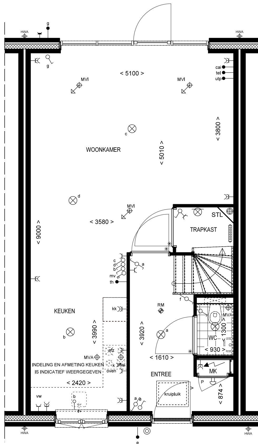
BEGANE GROND
