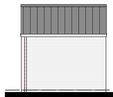
VOORGEVEL
