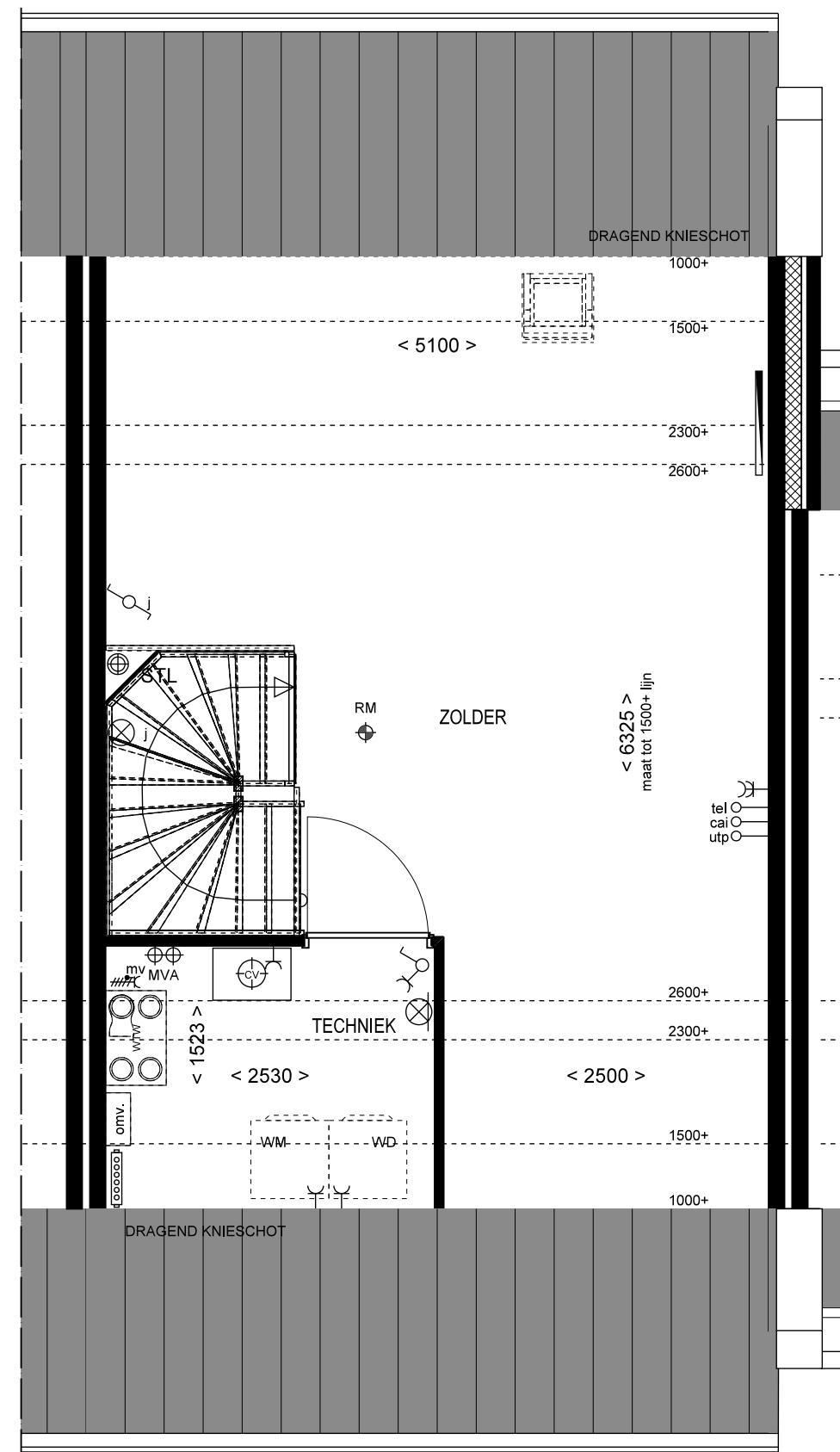
2e VERDIEPING
