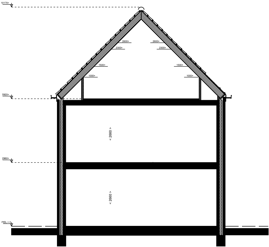
DOORSNEDE
