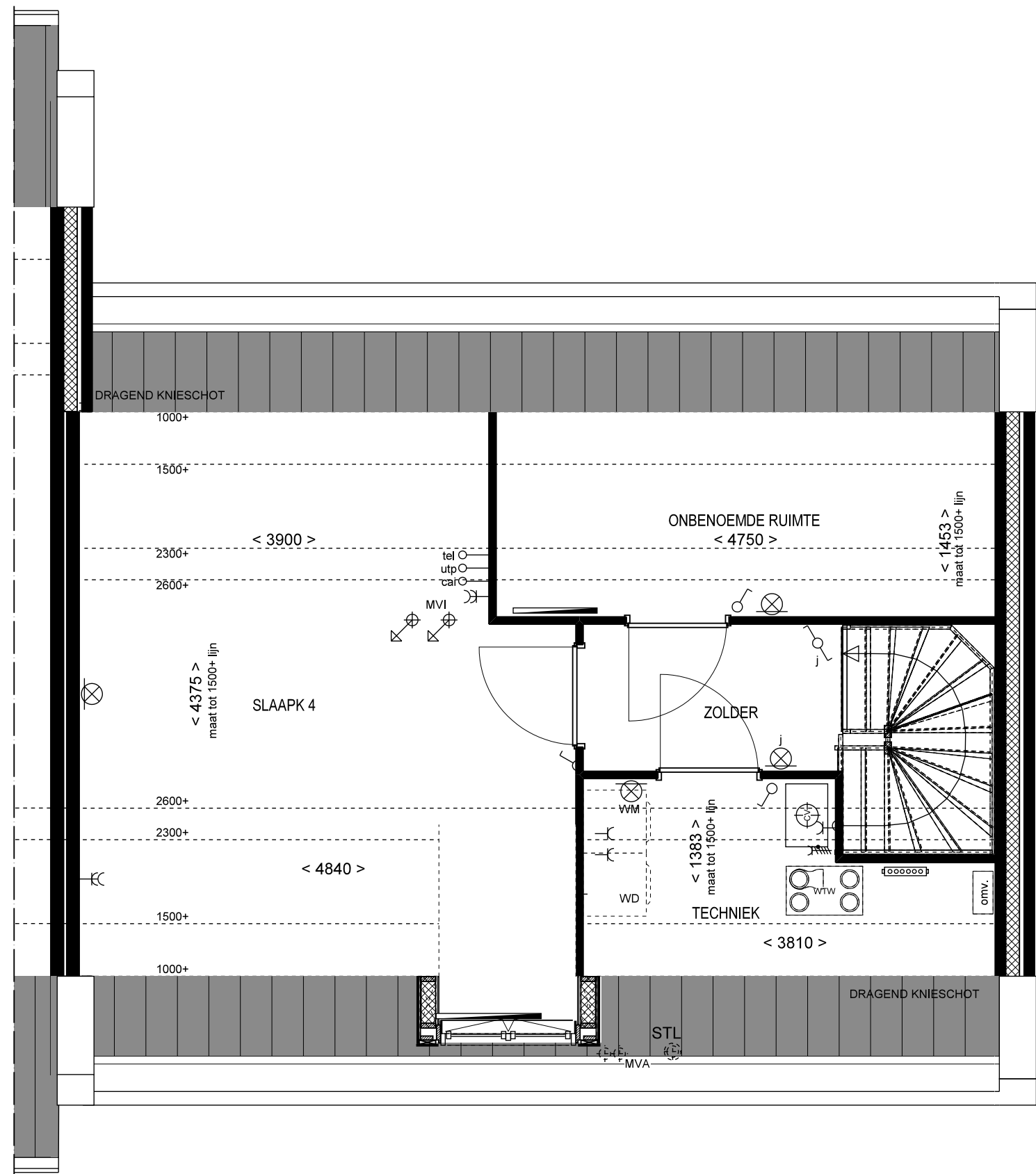
2e VERDIEPING
