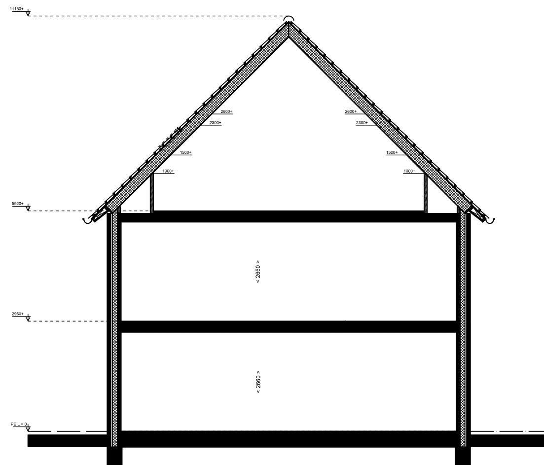
DOORSNEDE
