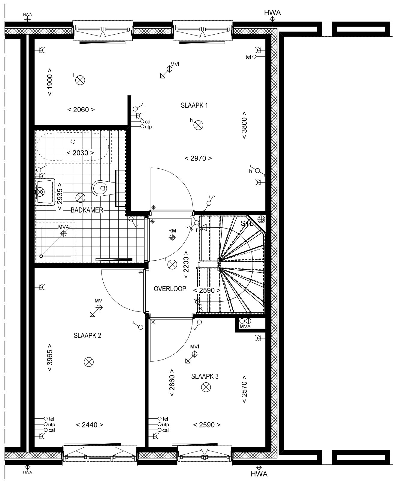
1e VERDIEPING
