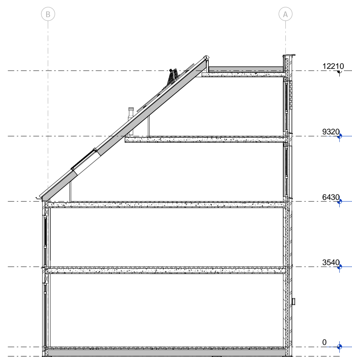
Doorsnede principe
