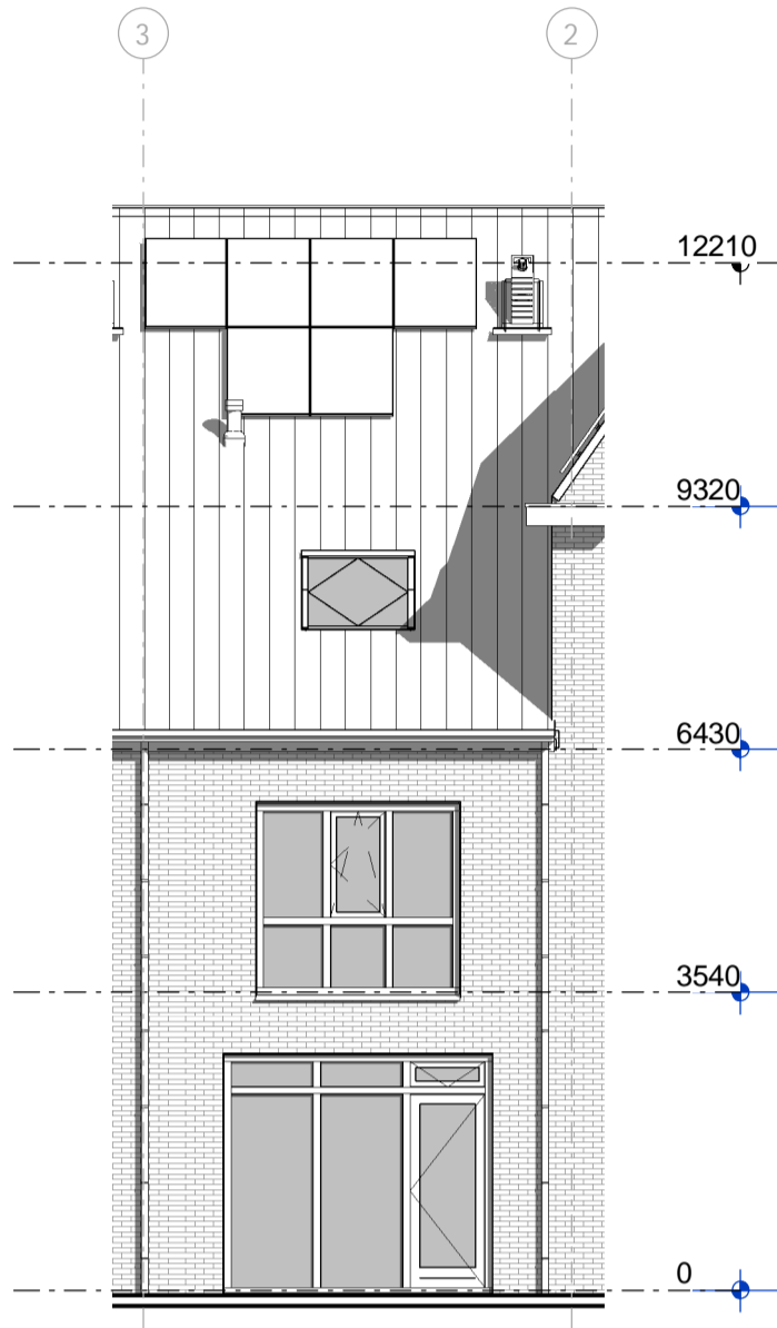
achtergevel
