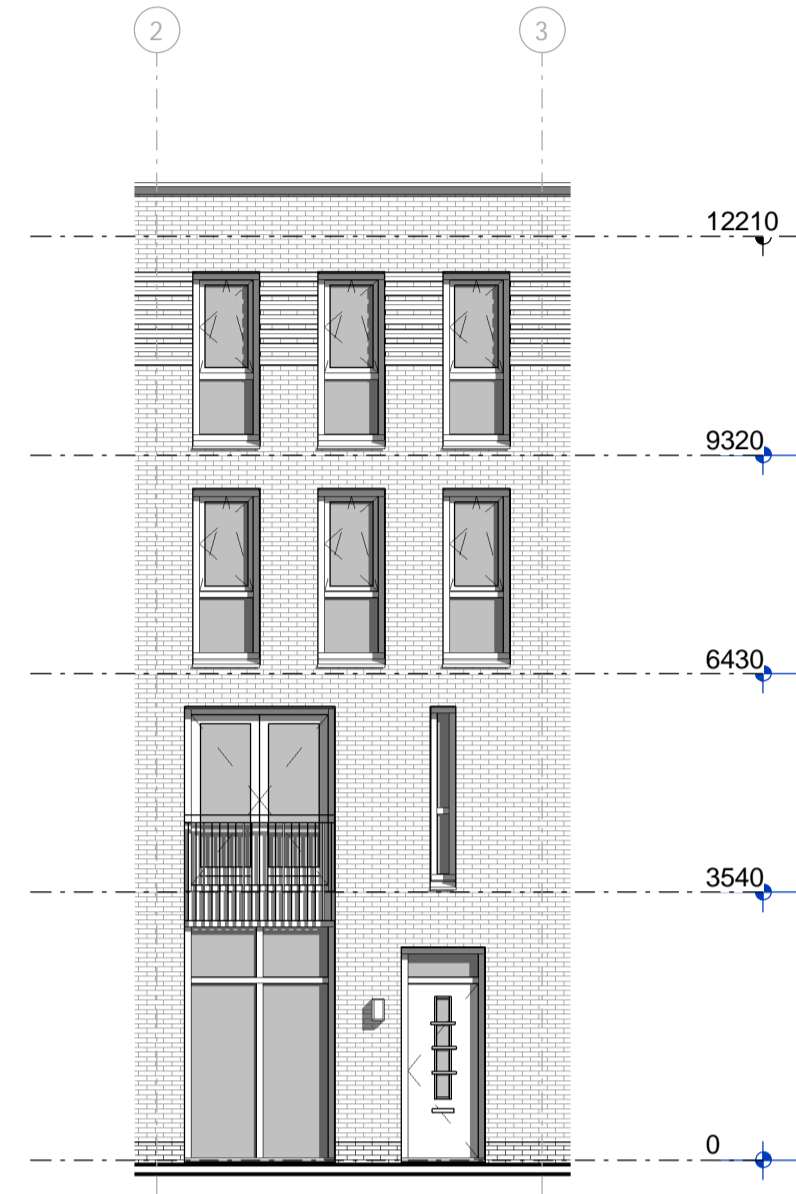
voorgevel
