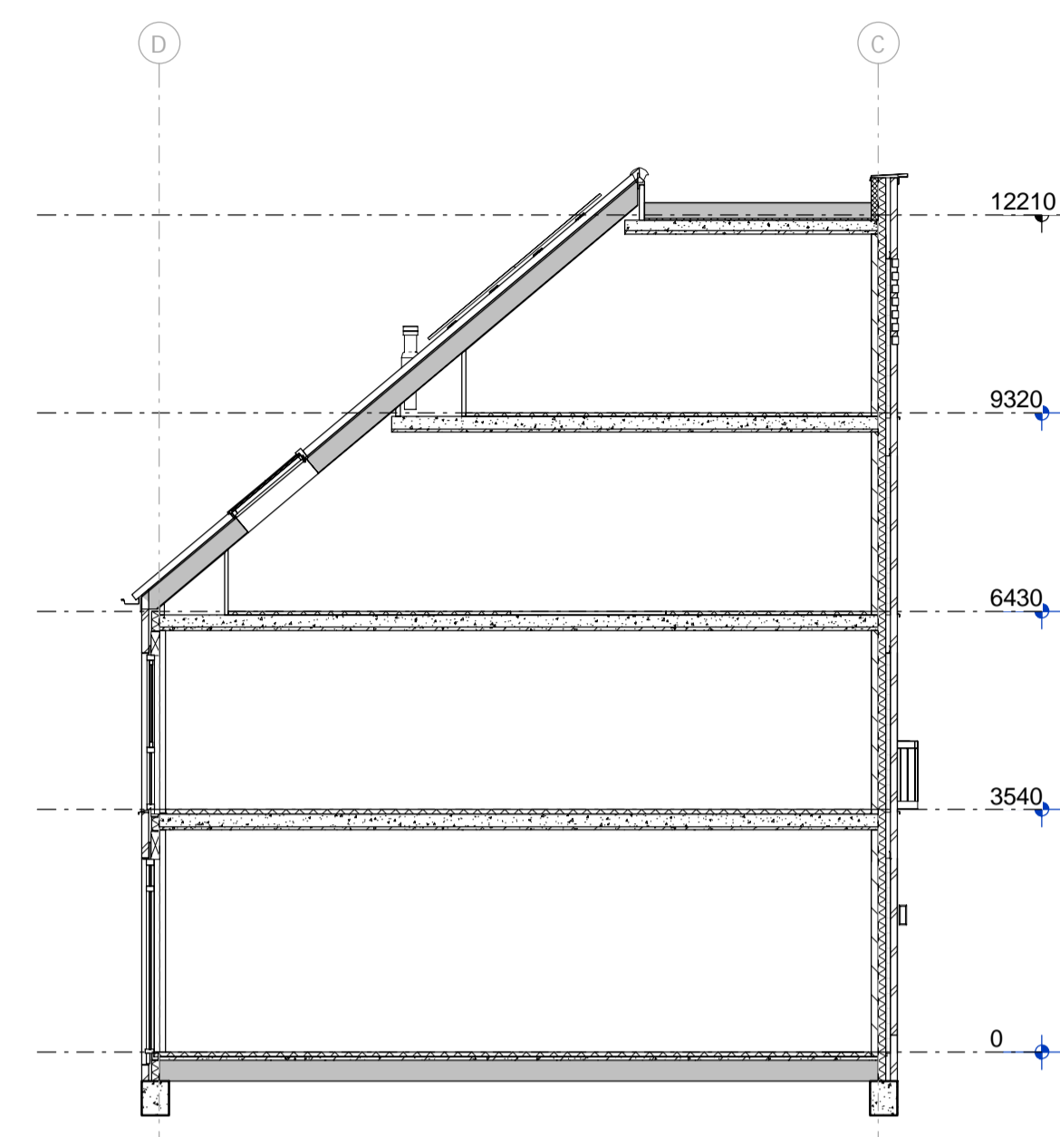
Doorsnede principe
