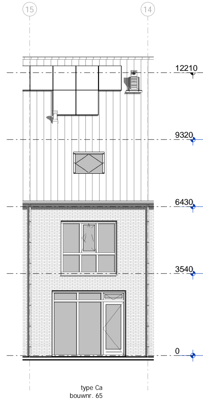
achtergevel
