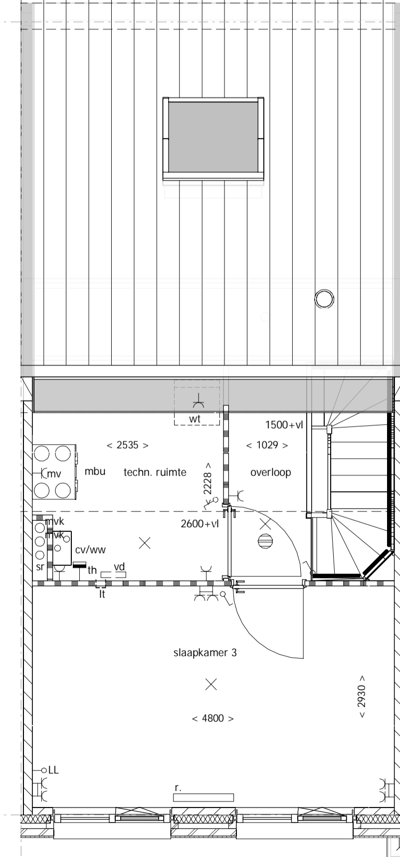
3e verdieping
