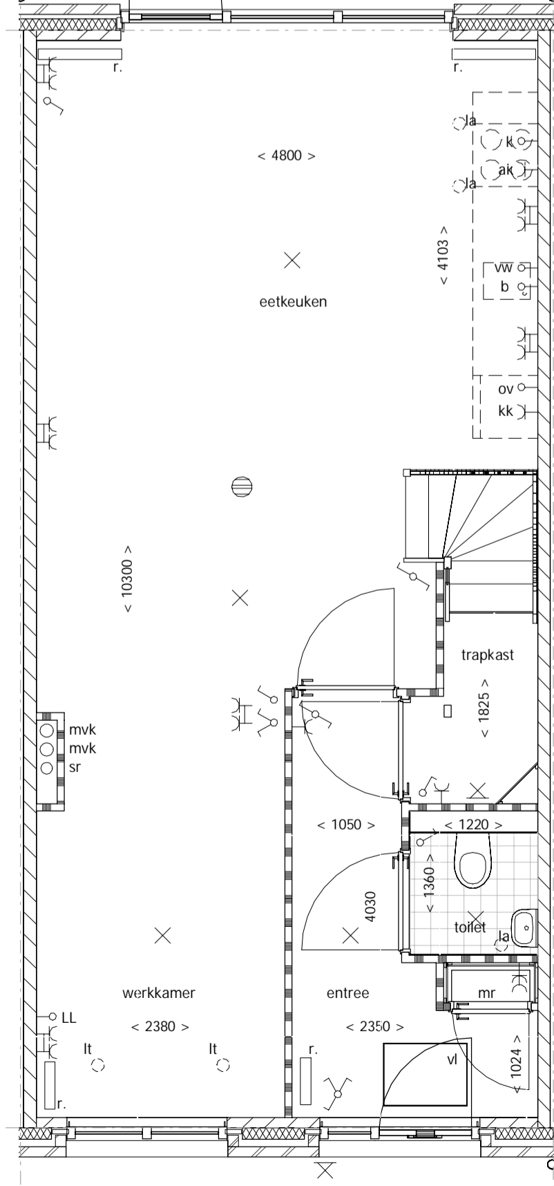
begane grond
