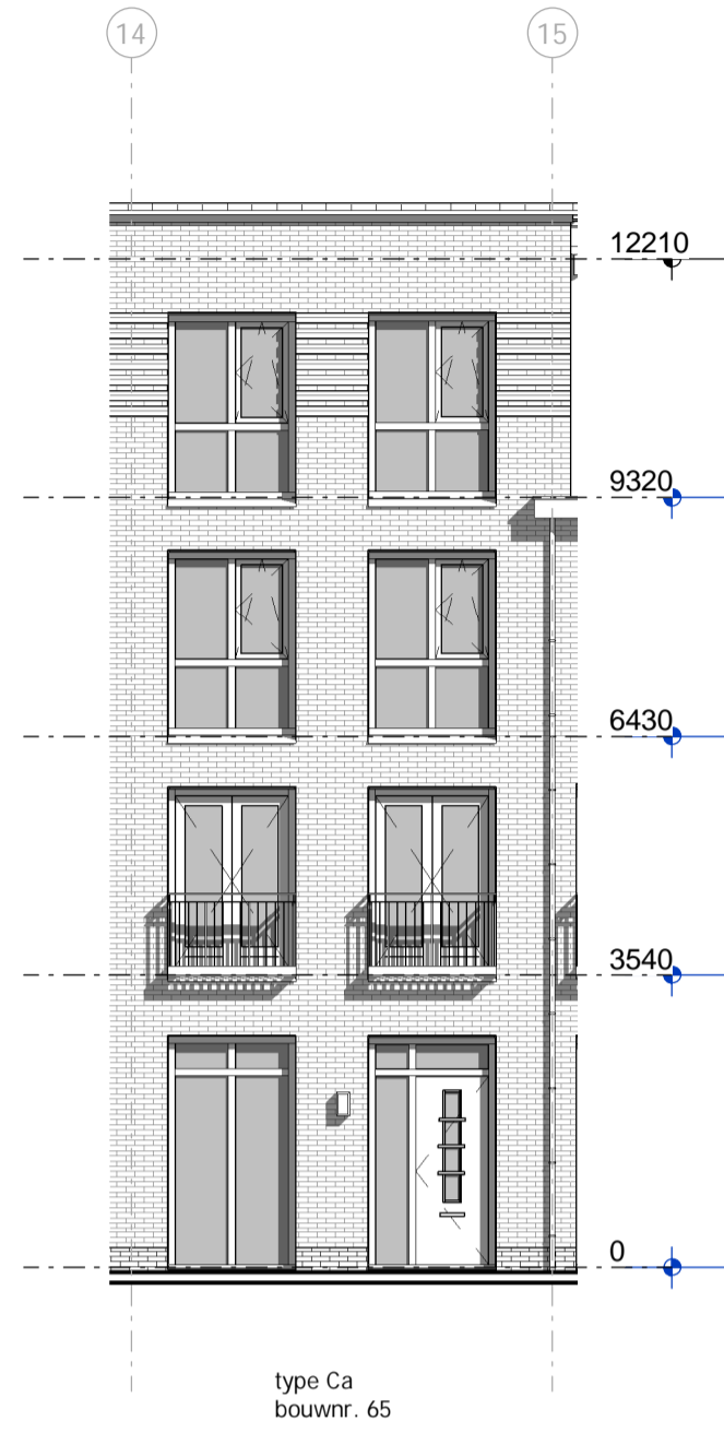
voorgevel
