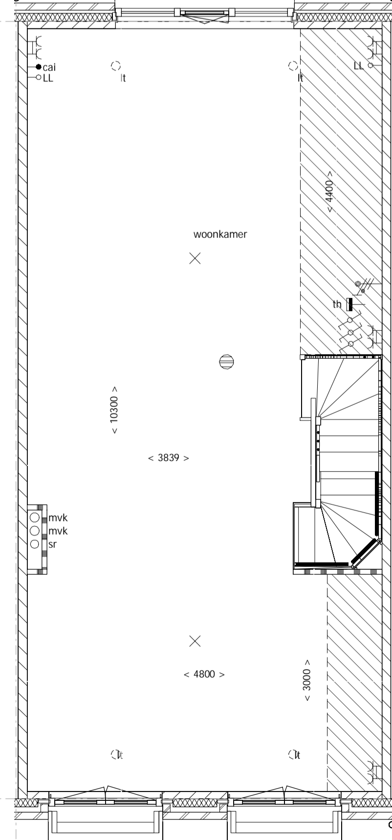
1e verdieping
