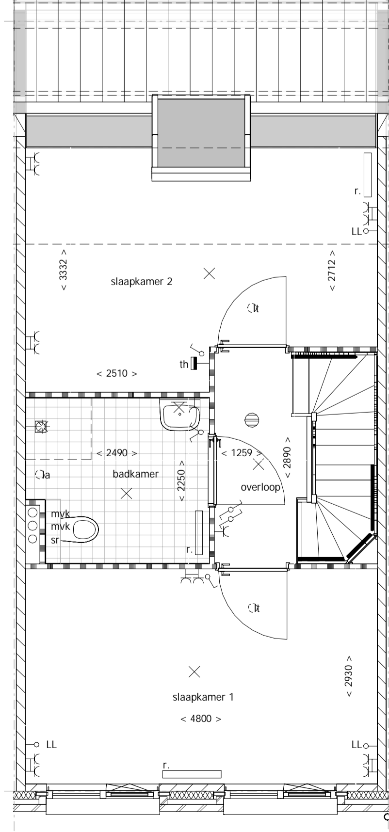
2e verdieping
