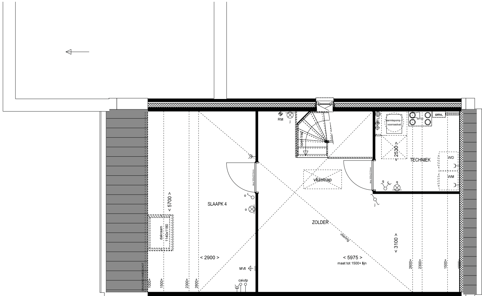
2e VERDIEPING BNR 14 TYPE C3
