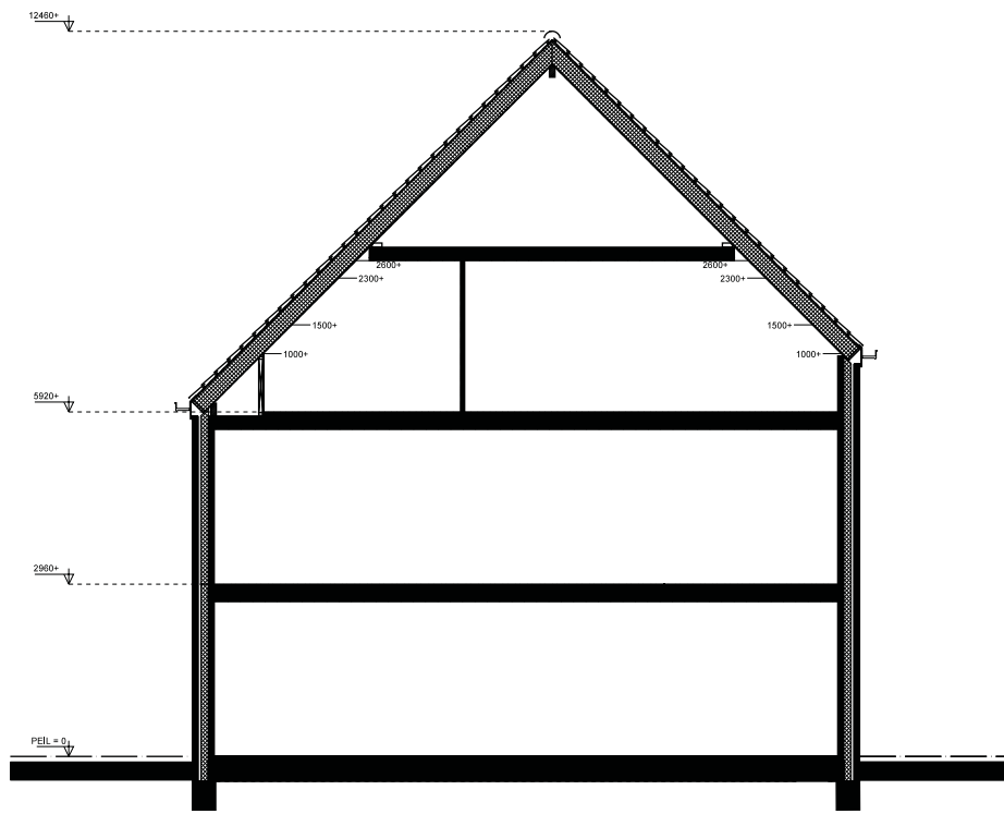
DOORSNEDE type C3
