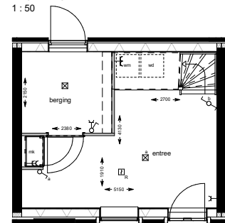
begane grond bnr. 05 1: 50
