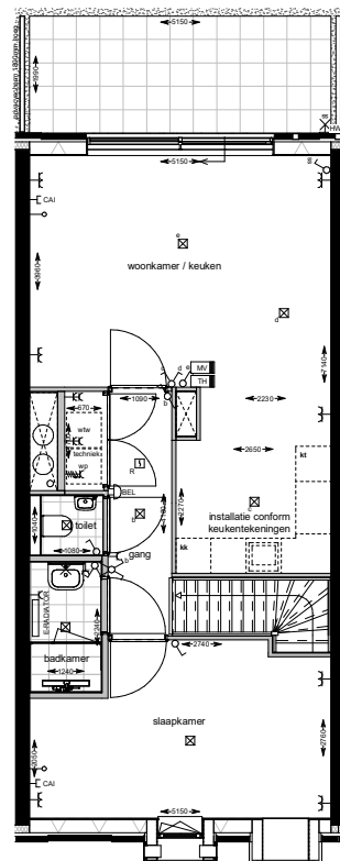
eerste verdieping bnr. 05 1: 50
