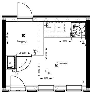
begane grond bnr. 03 en 04 1: 50
