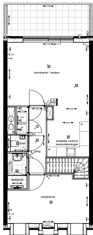
eerste verdieping bnr. 03 en 04 1: 50
