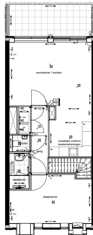
eerste verdieping bnr. 06 en 07 1: 50
