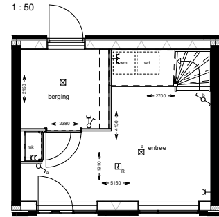
begane grond bnr. 06 en 07 1: 50
