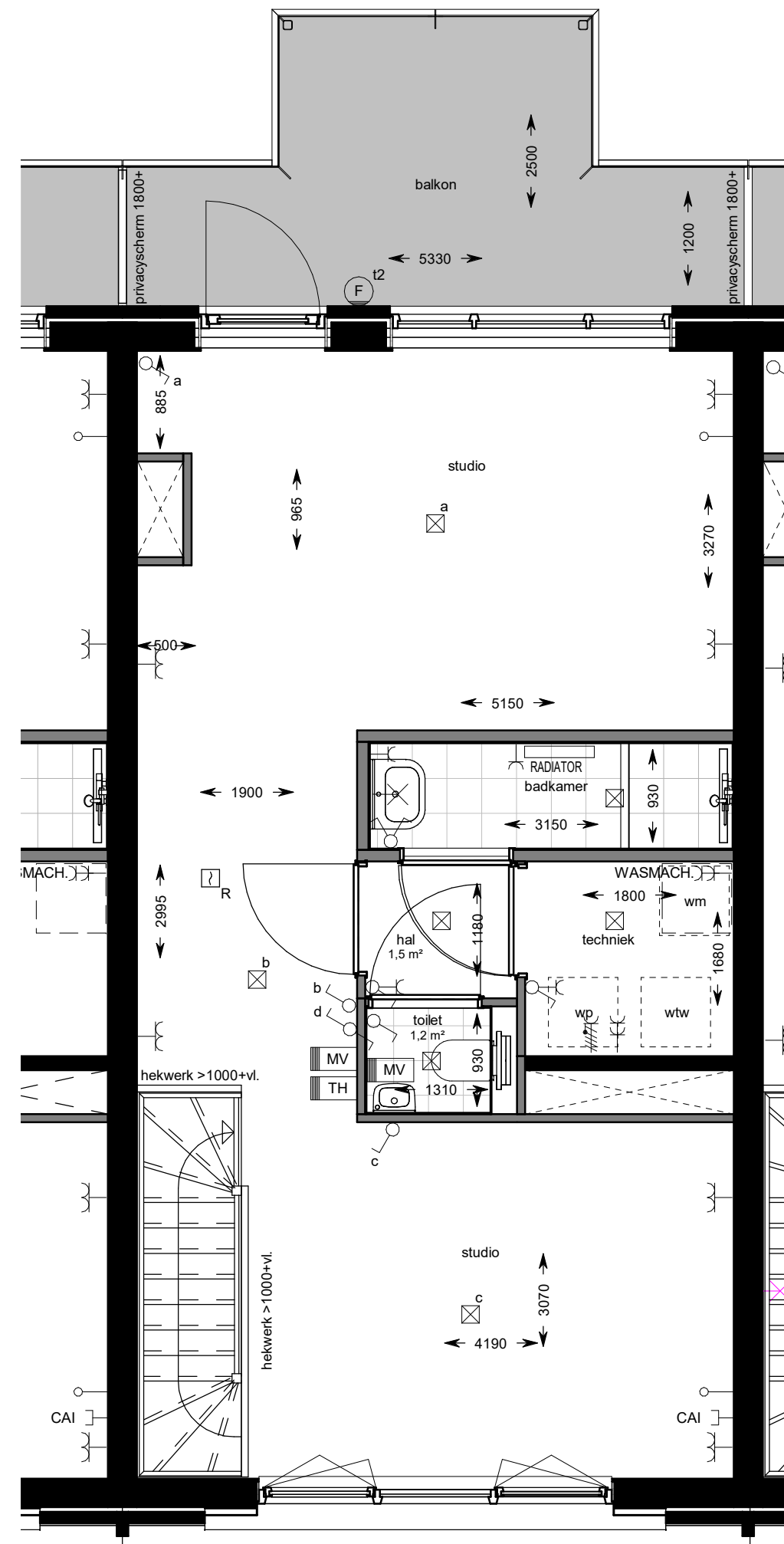
eerste verdieping
