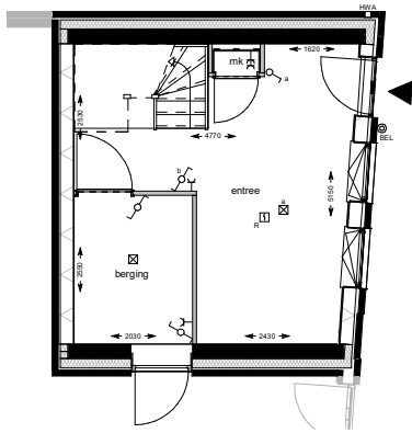
begane grond 1 : 50
