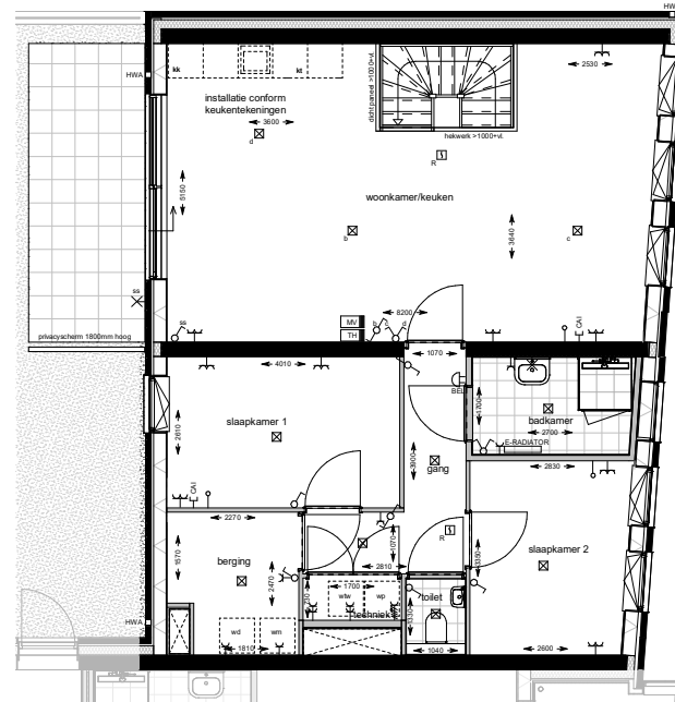
eerste verdieping 1 : 50
