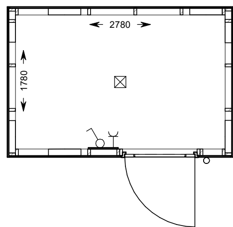
begane grond
