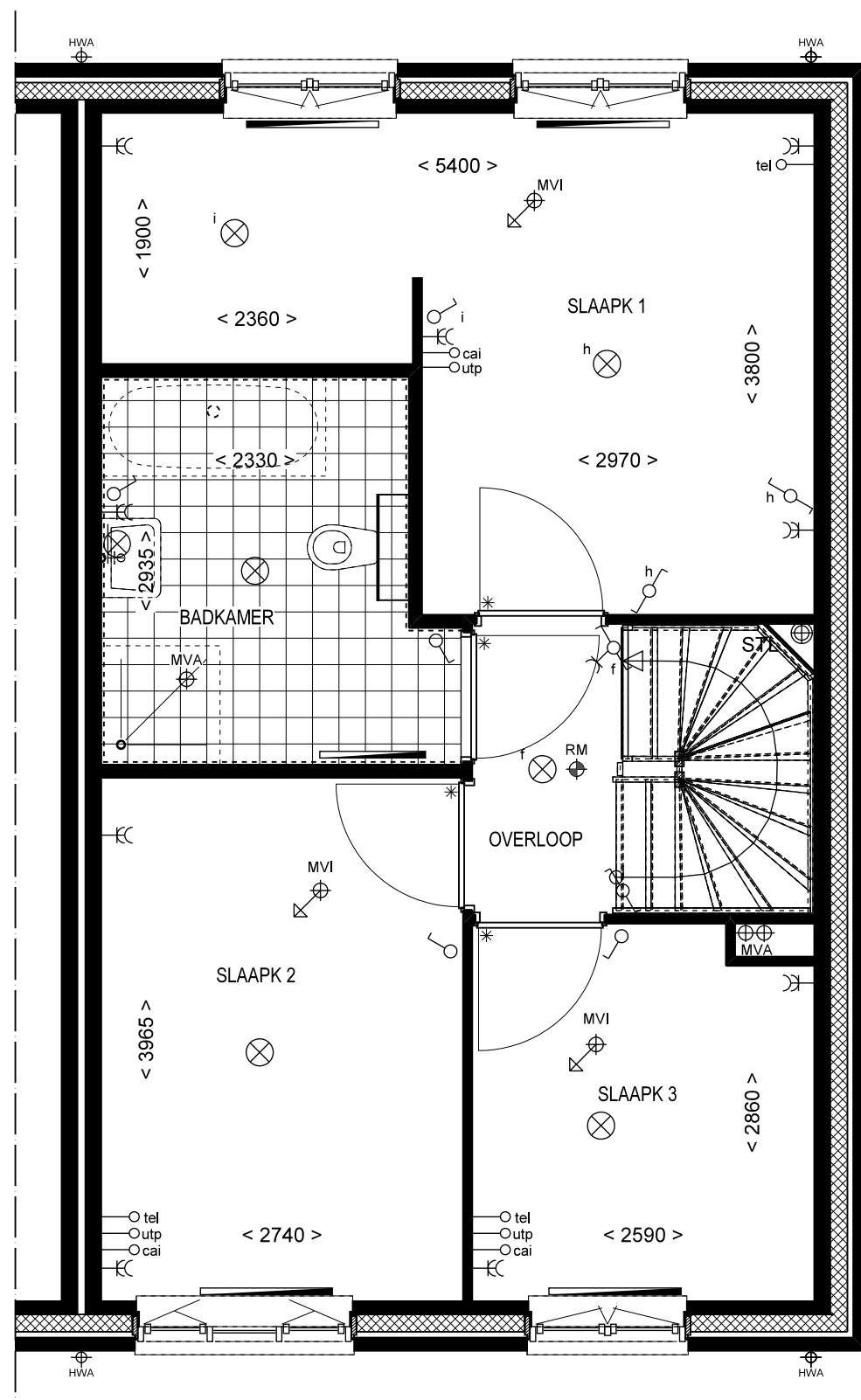
1e VERDIEPING
