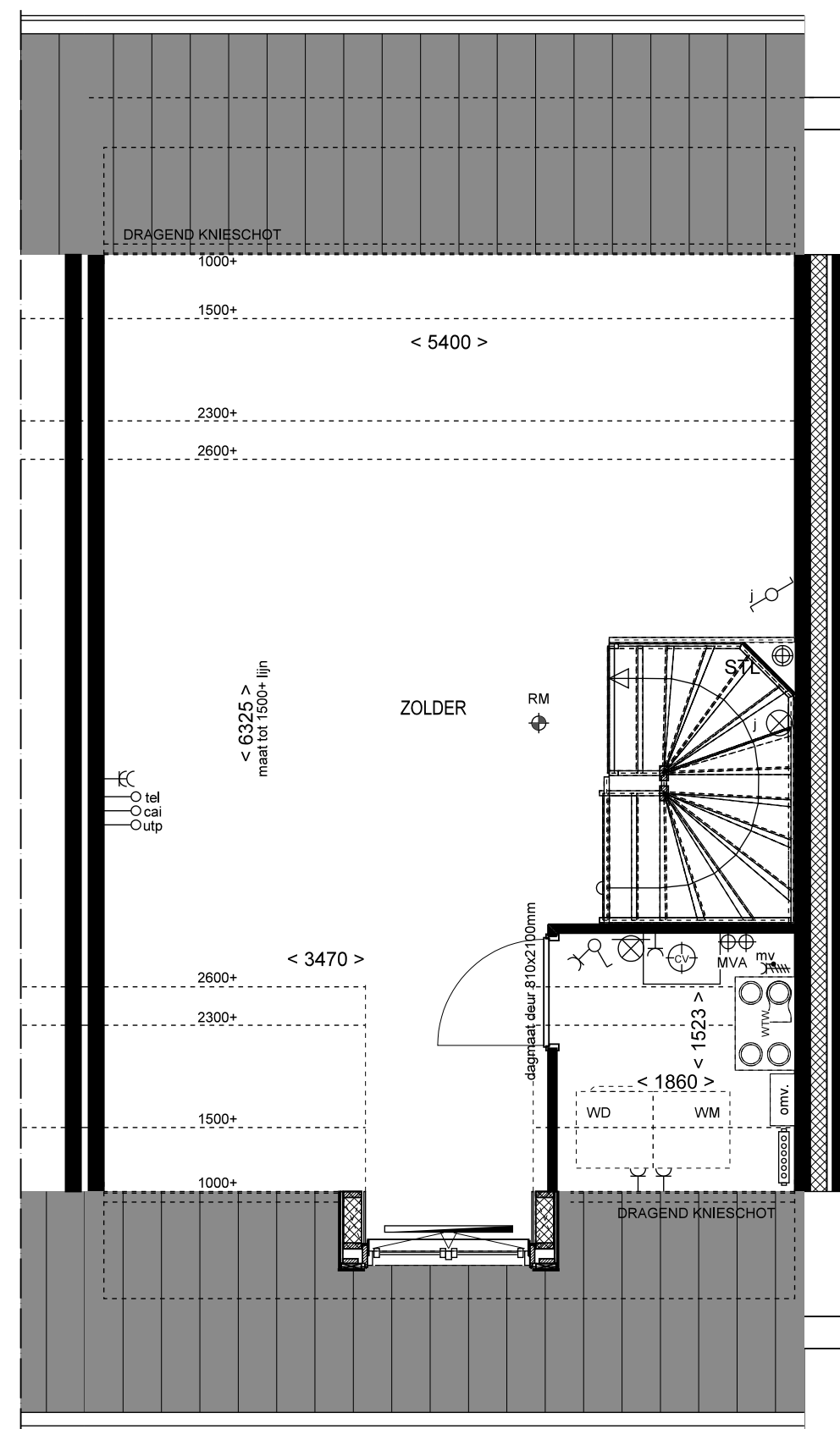
2e VERDIEPING
