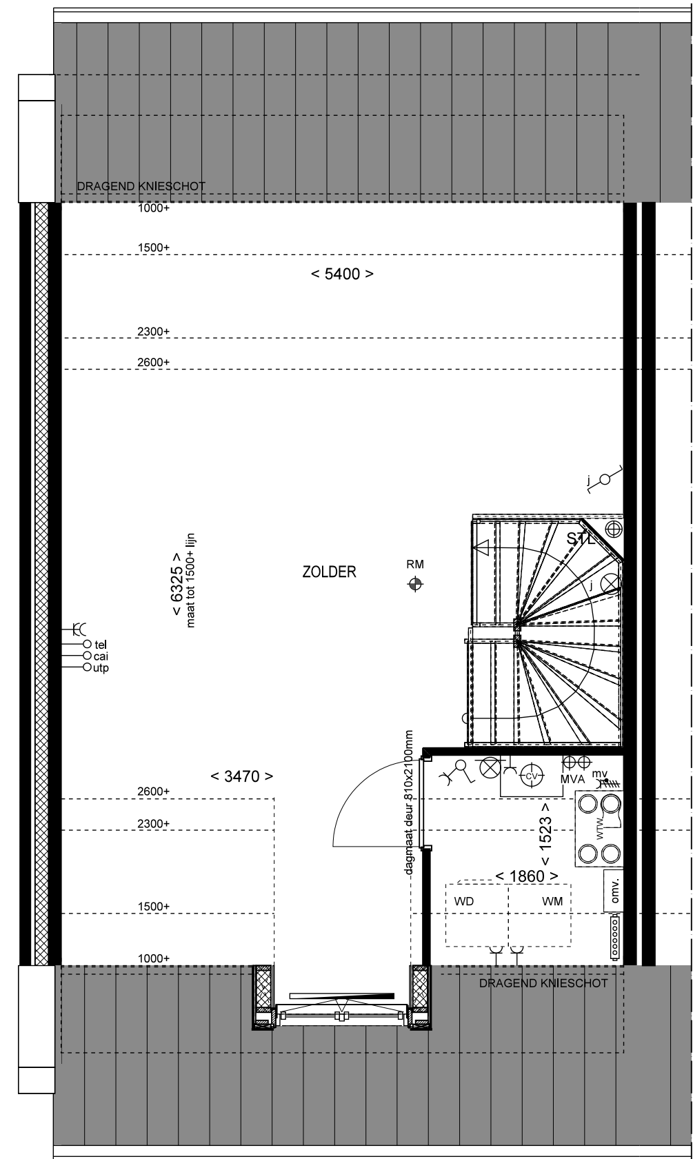
2e VERDIEPING
