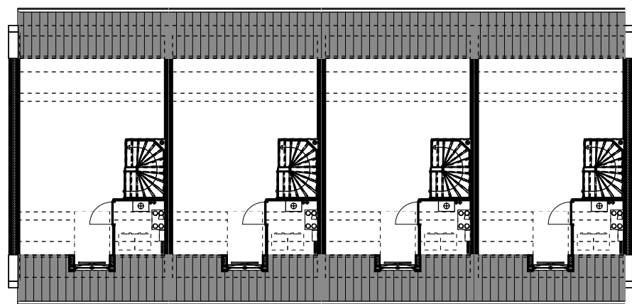
BNR 13 TYPE B1l BNR 12 TYPE B1 BNR 11 TYPE B1 BNR 10 TYPE B1r
