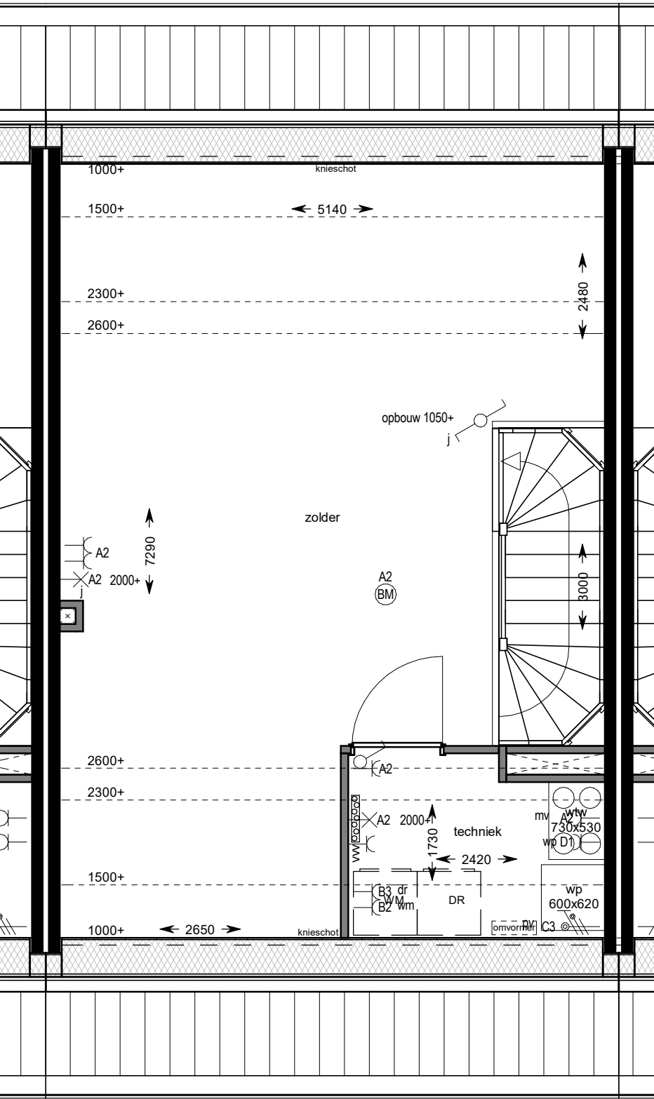
tweede verdieping
