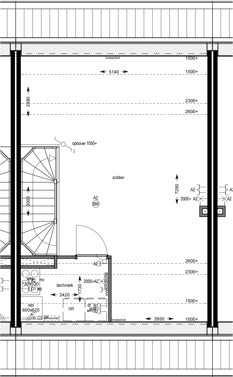
tweede verdieping
