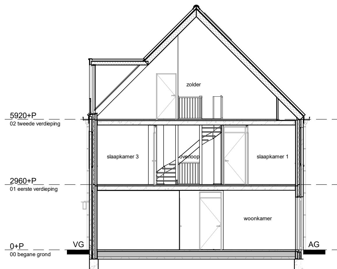
doorsnede
