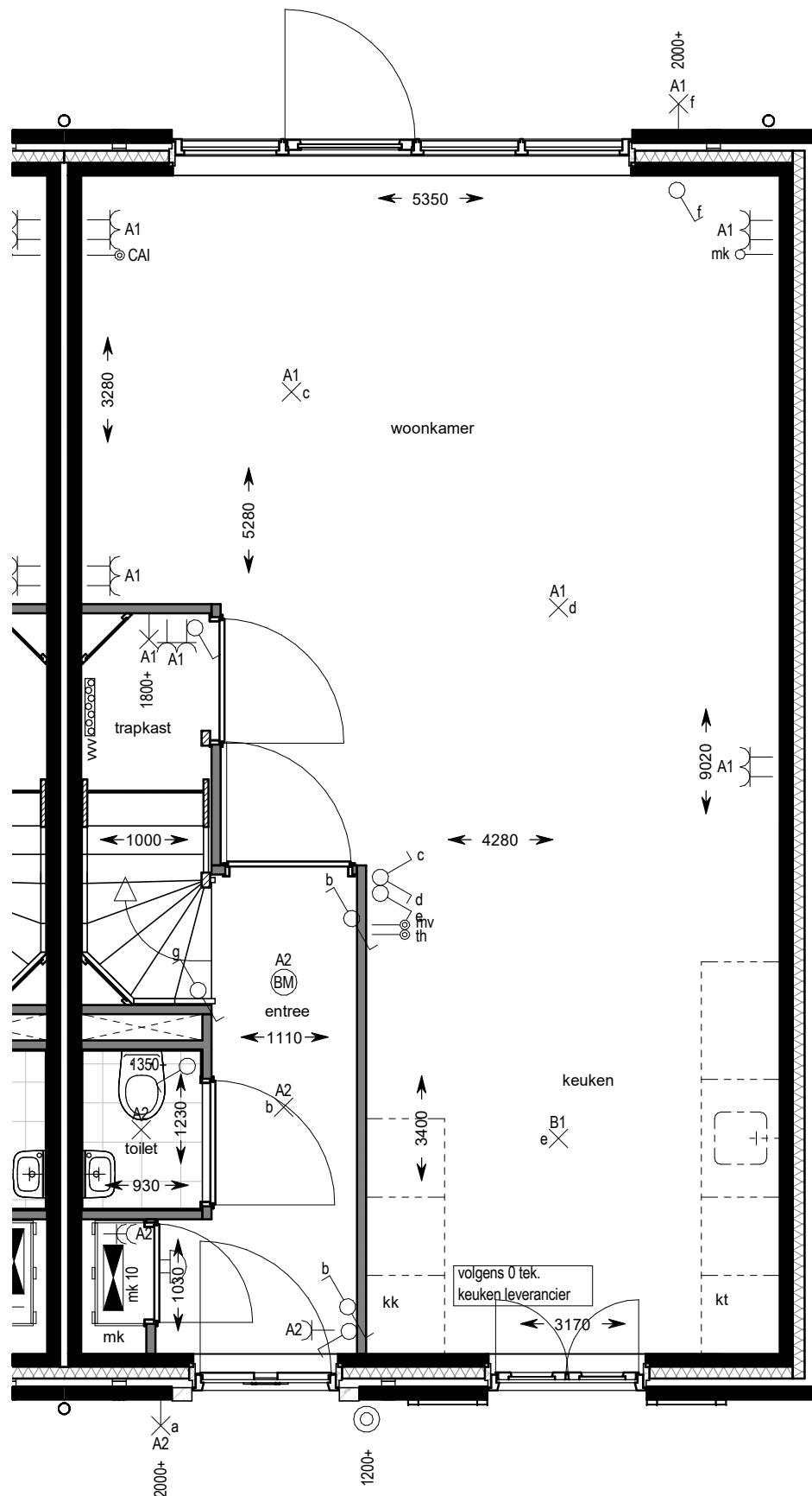
begane grond
