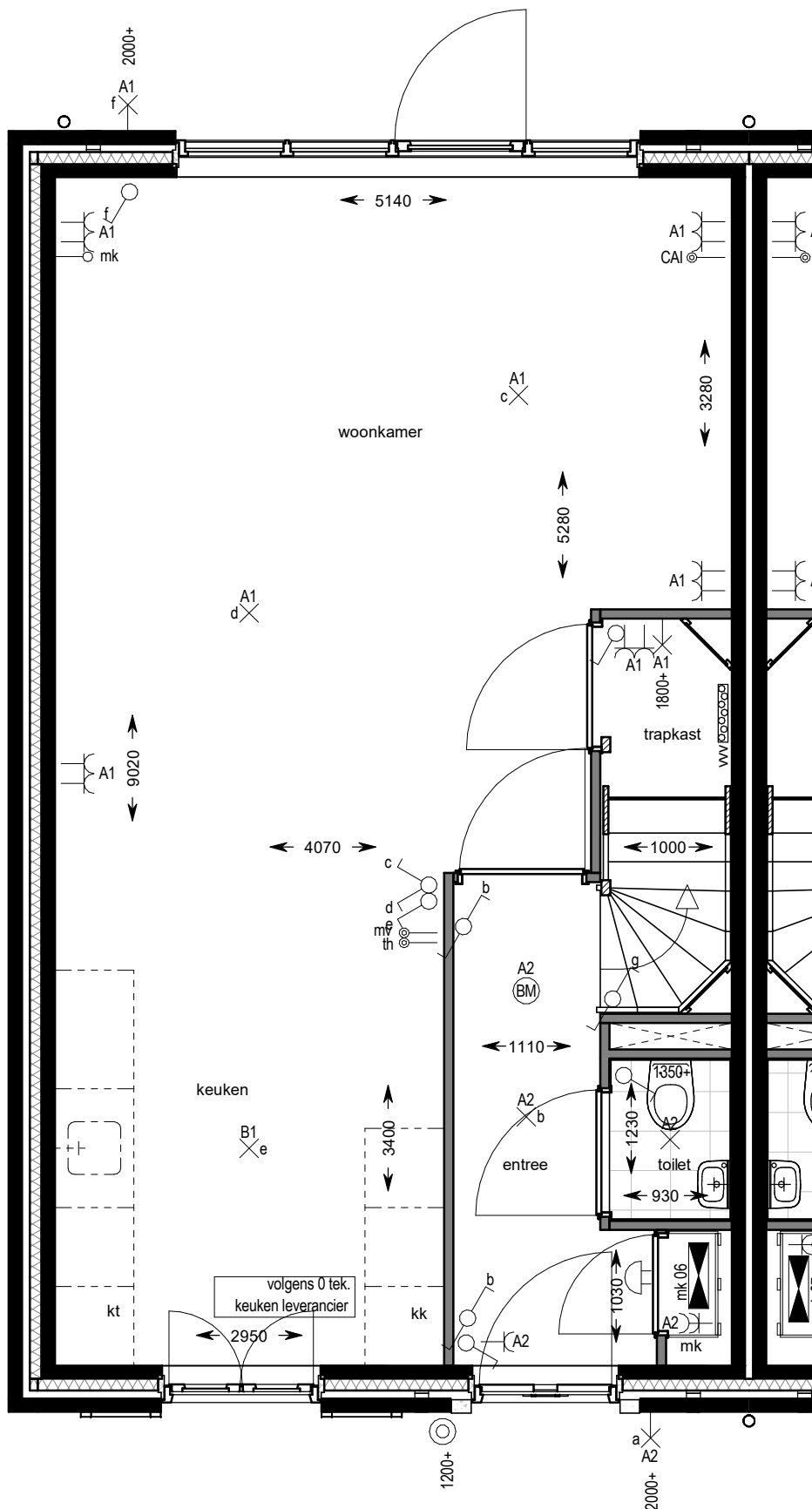
begane grond
