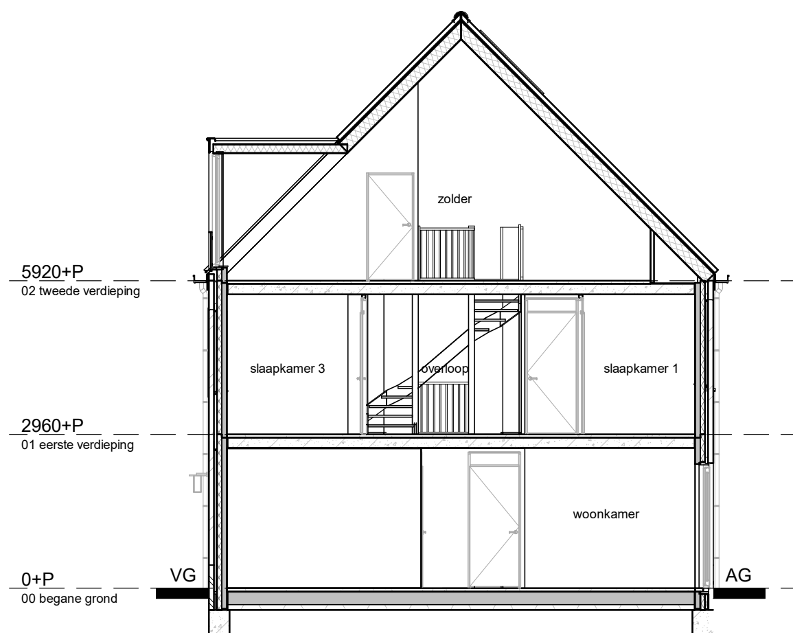
doorsnede
