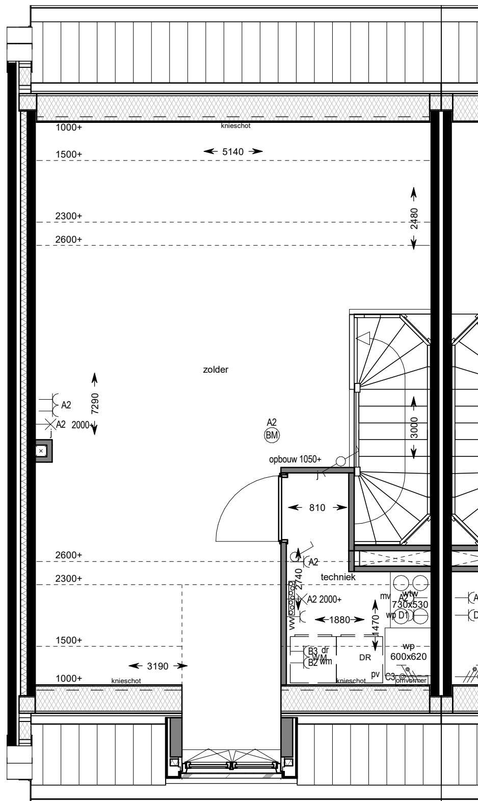
tweede verdieping
