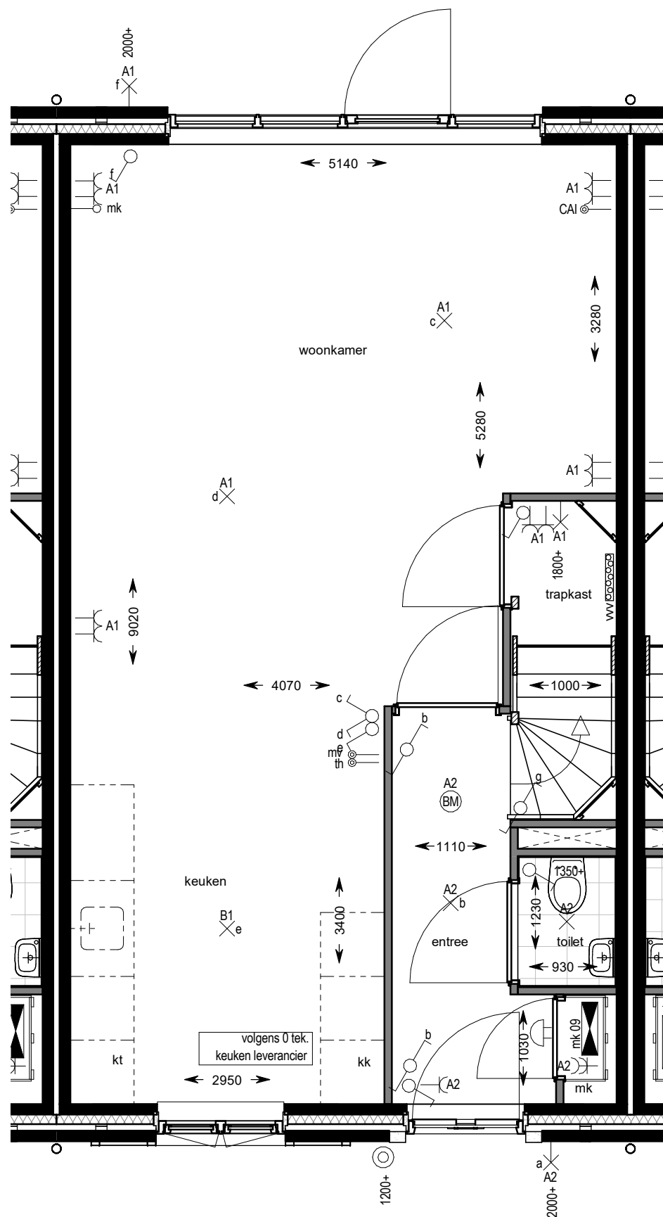
begane grond
