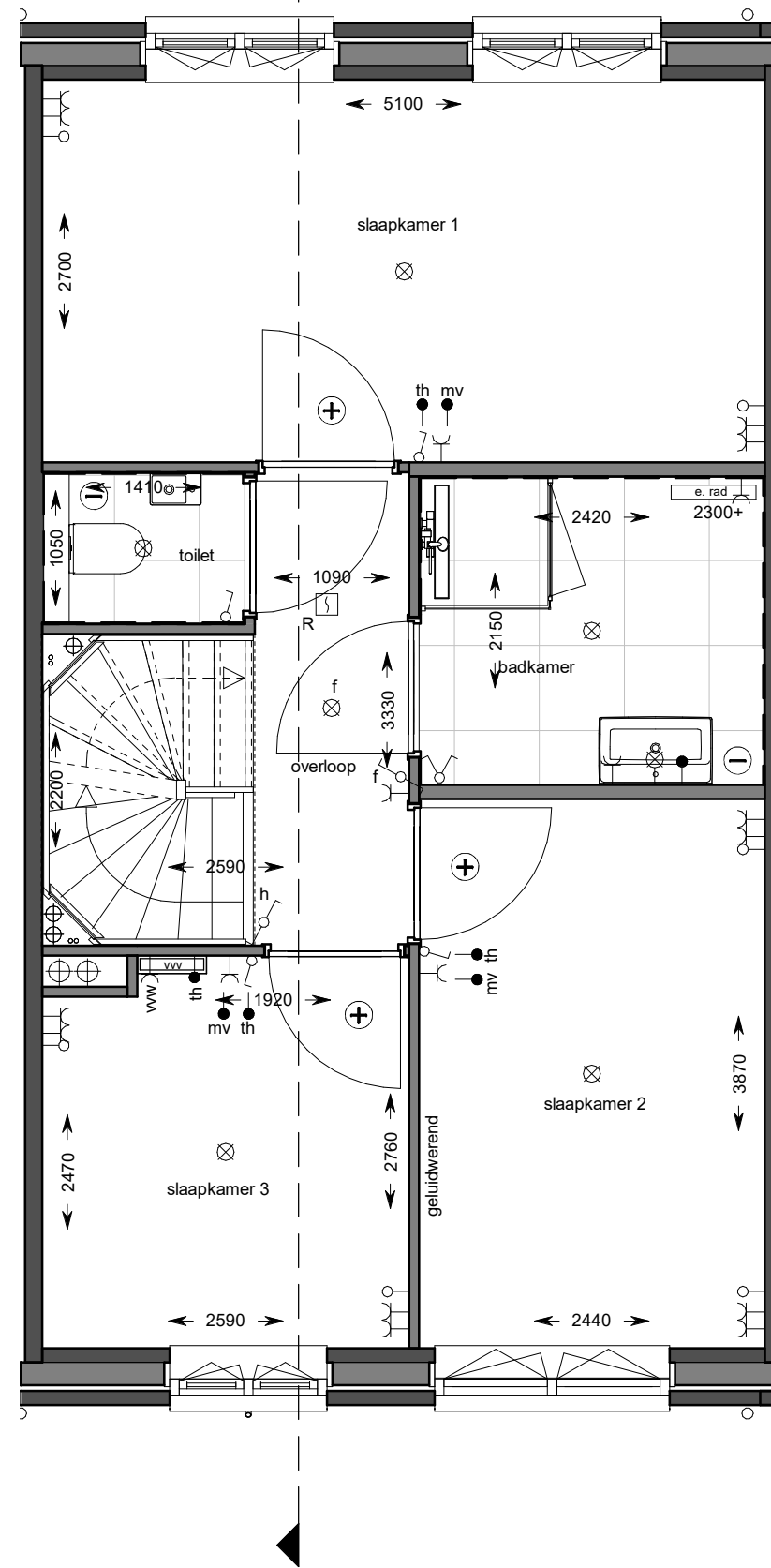
eerste verdieping
