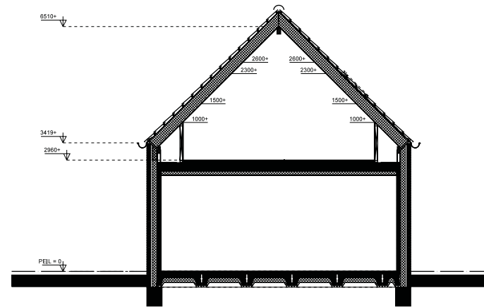
DOORSNEDE
