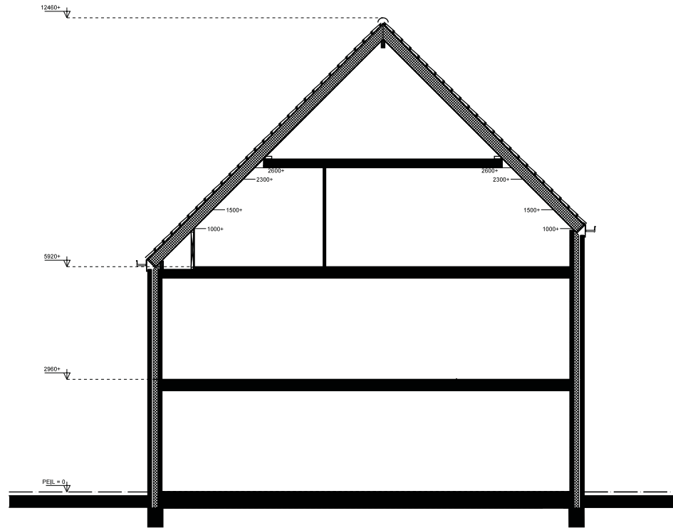
DOORSNEDE type C3
