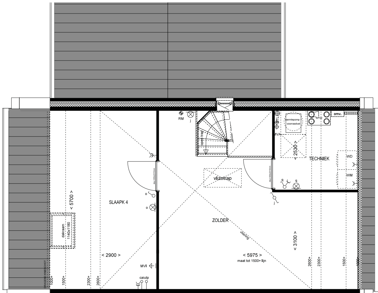
2e VERDIEPING BNR 8 TYPE C3
