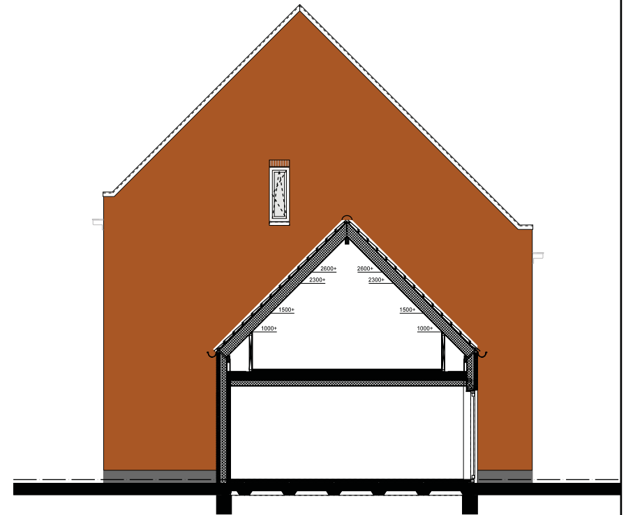
ZIJGEVEL
