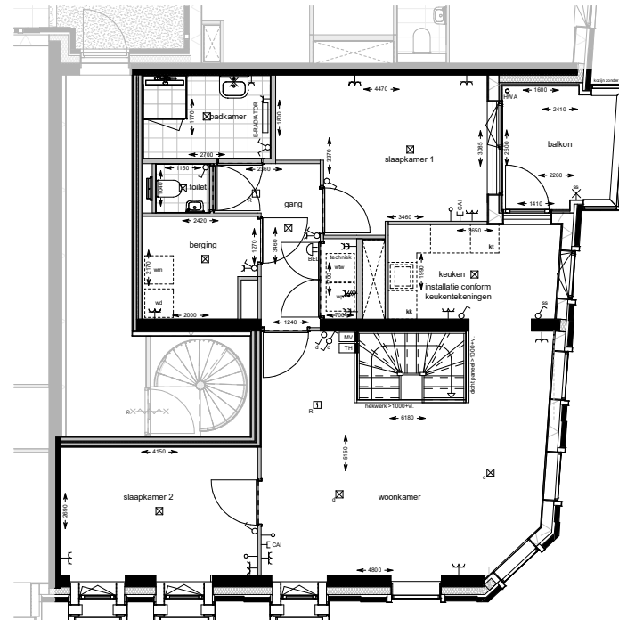
eerste verdieping 1: 50
