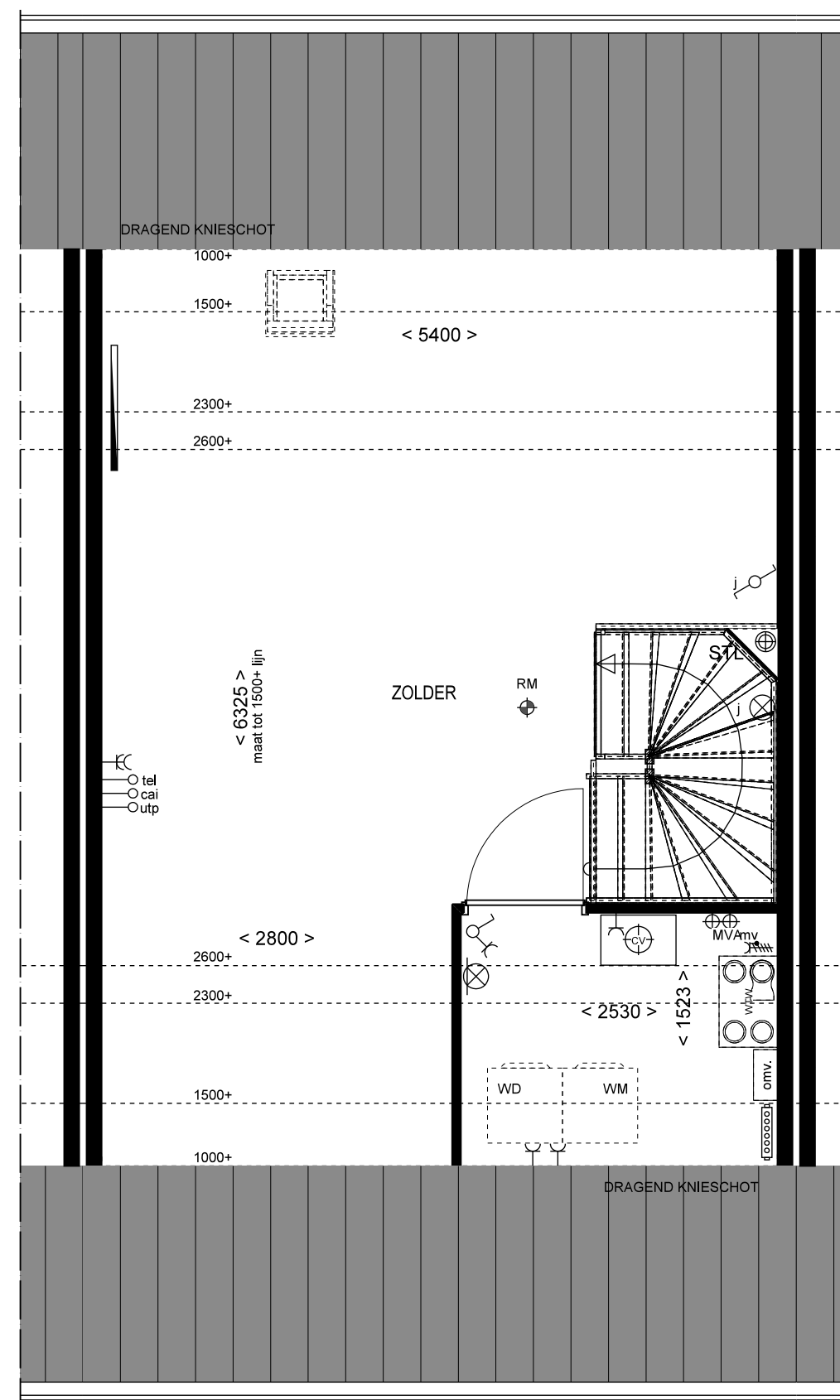
2e VERDIEPING
