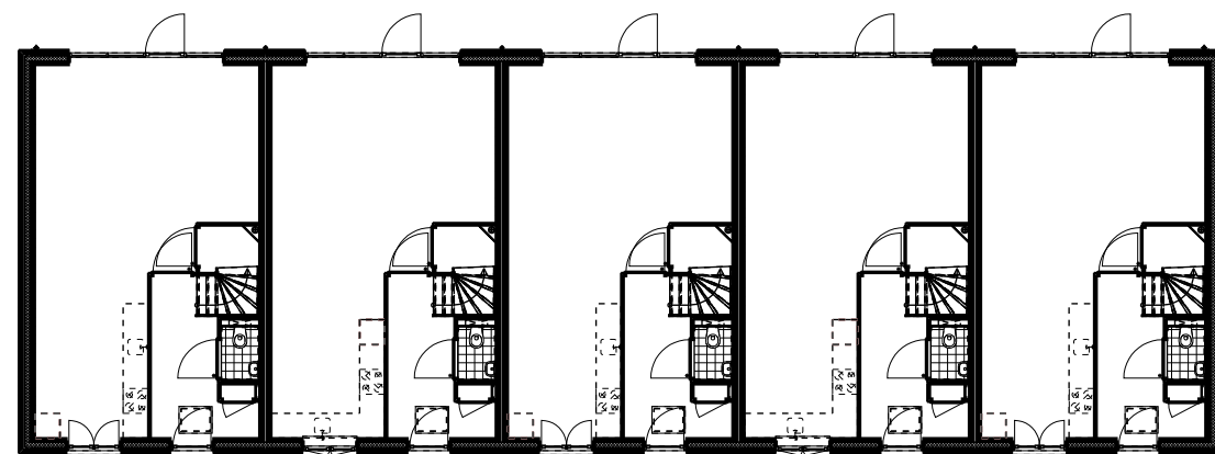
BNR 38 TYPE B2l BNR 37 TYPE B3 BNR 36 TYPE B2 BNR 35 TYPE B3 BNR 34 TYPE B2r
