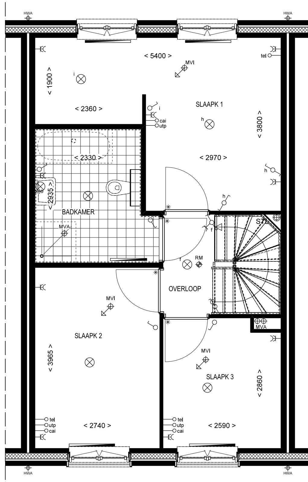
1e VERDIEPING
