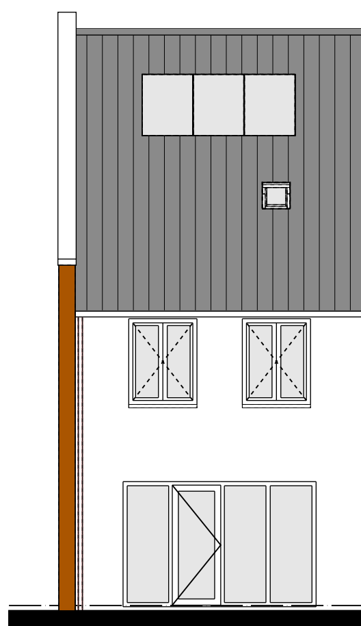
ACHTERGEVEL
