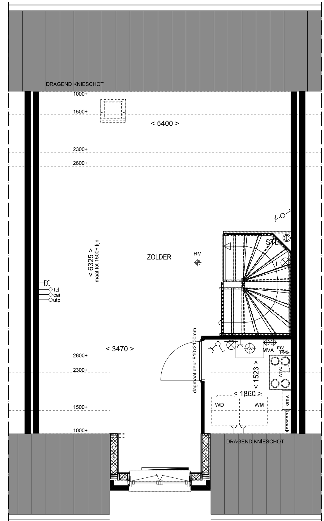
2e VERDIEPING
