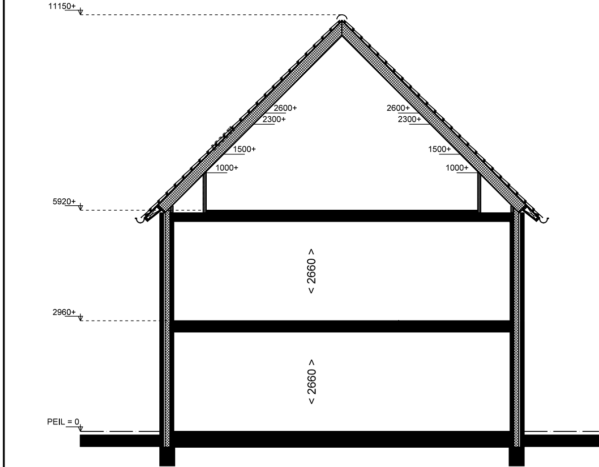
DOORSNEDE
