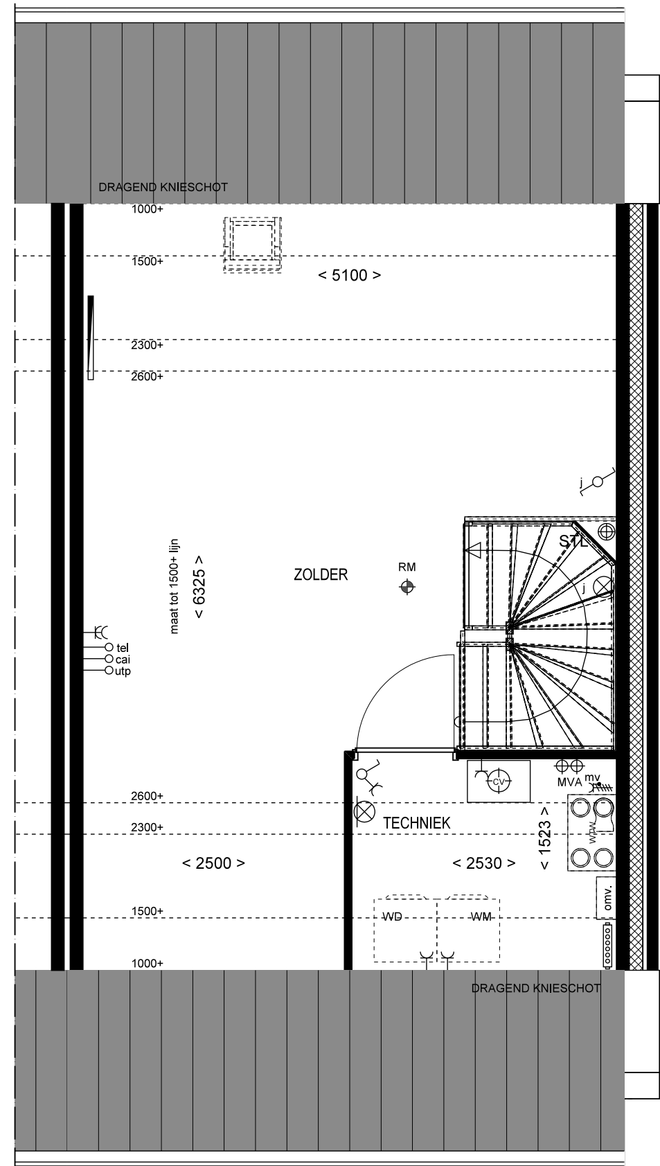
2e VERDIEPING
