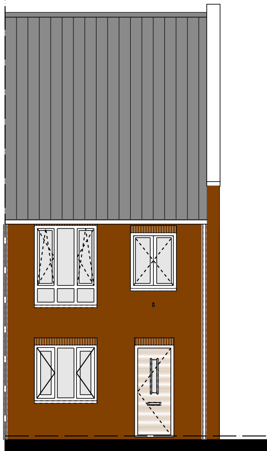
VOORGEVEL
