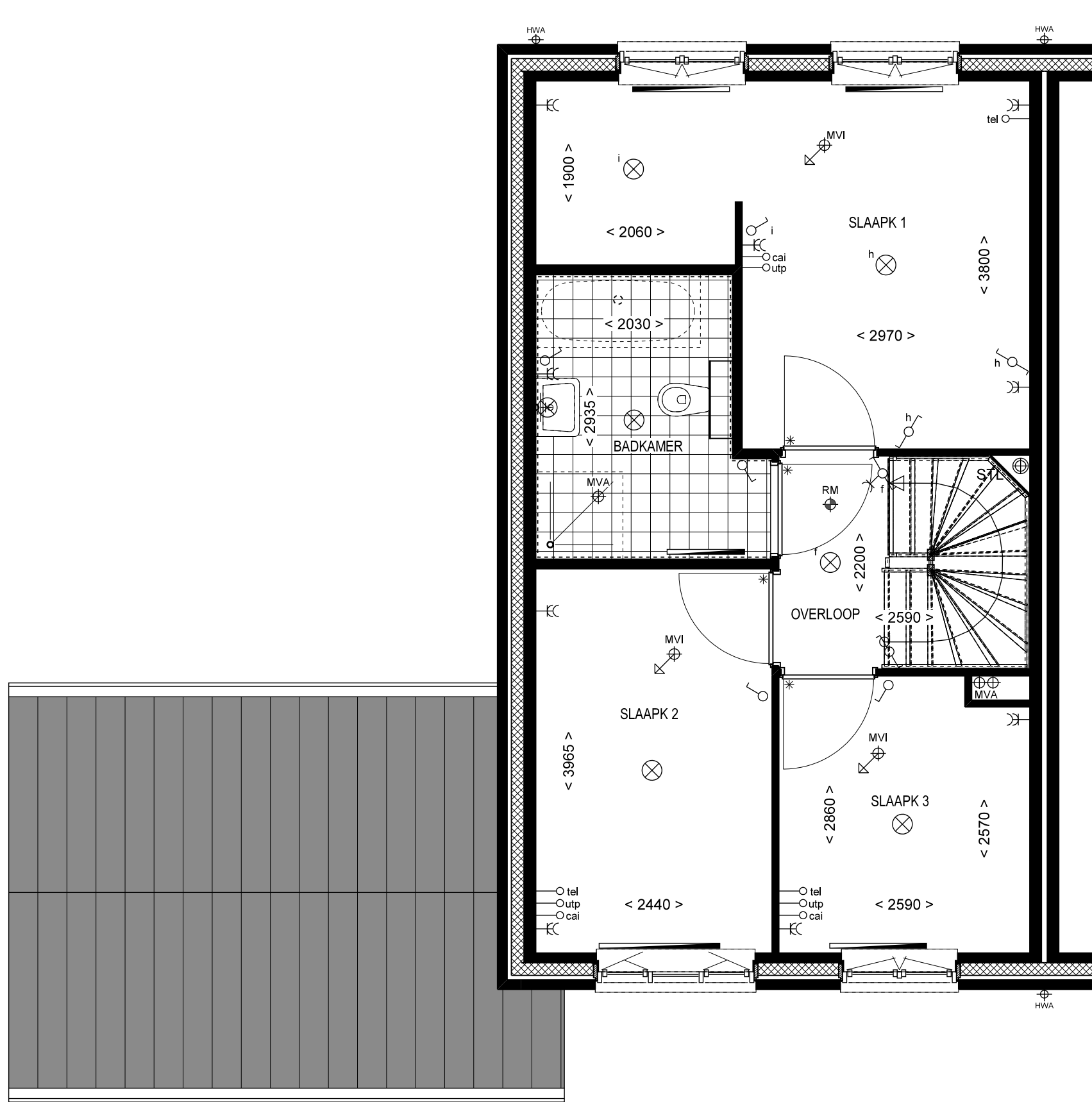
1e VERDIEPING
