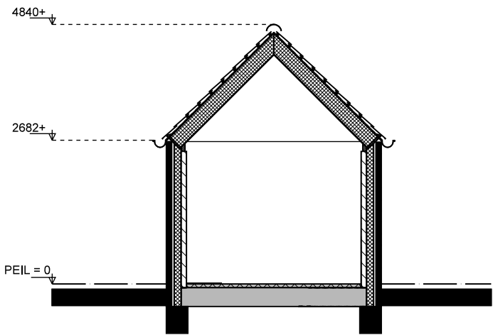
DOORSNEDE
