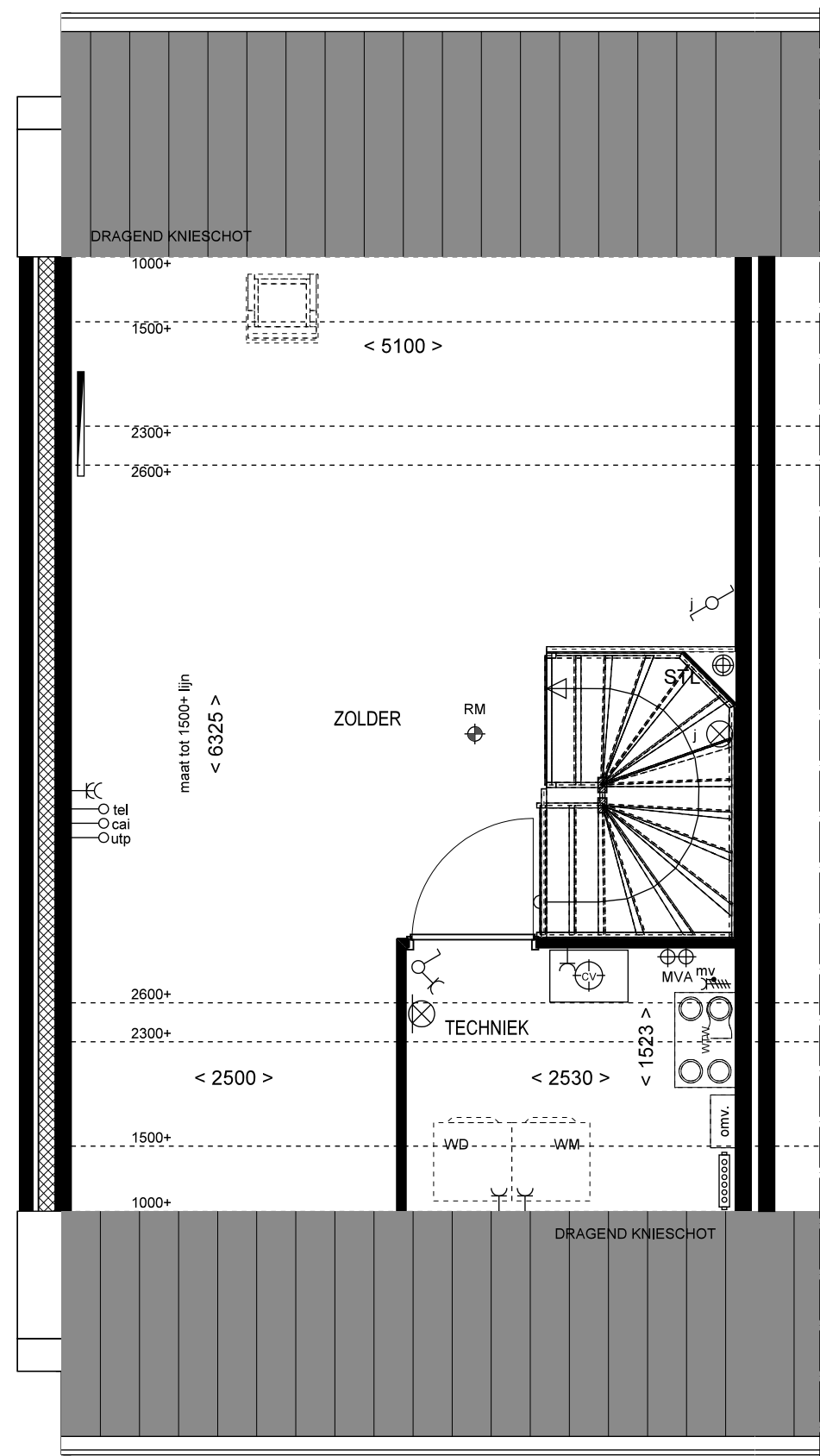
2e VERDIEPING
