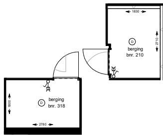
eerste verdieping 1 : 50
