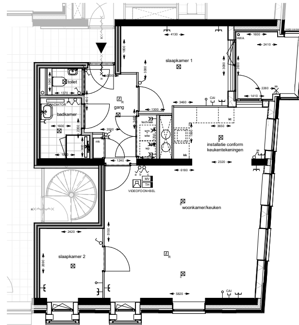
tweede/derde verdieping 1 : 50
