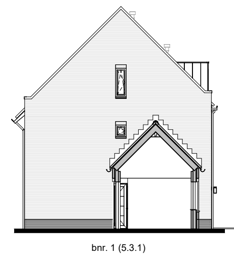
linkergevel
