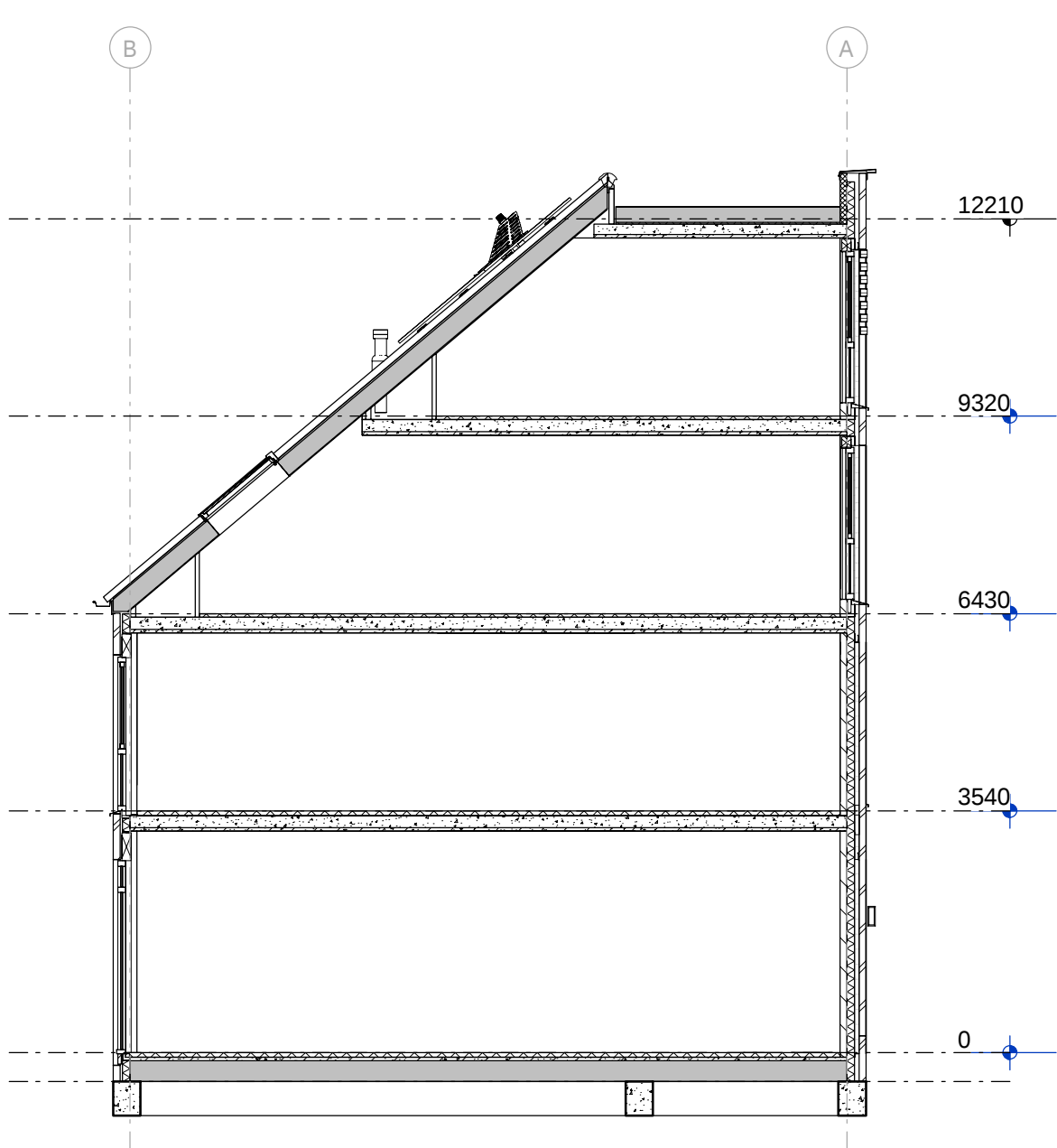
Doorsnede principe
