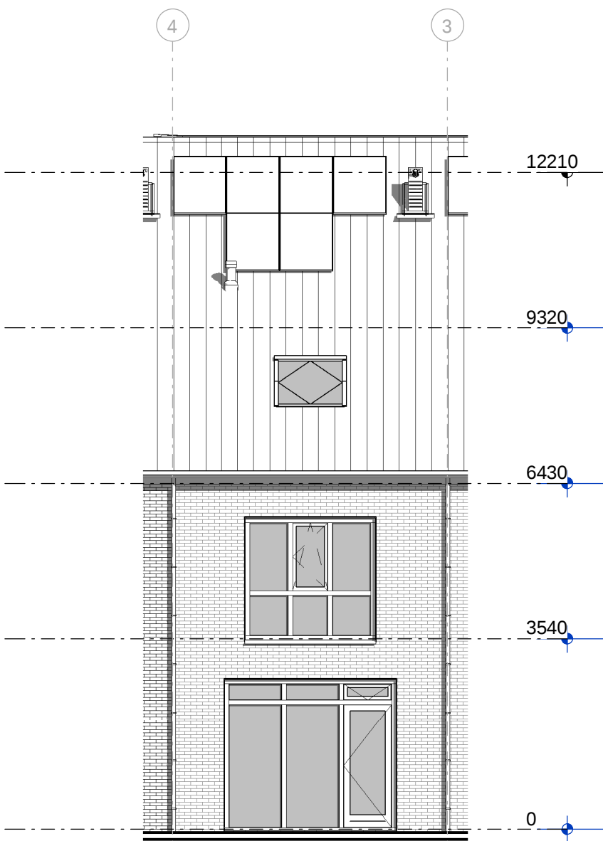
achtergevel
