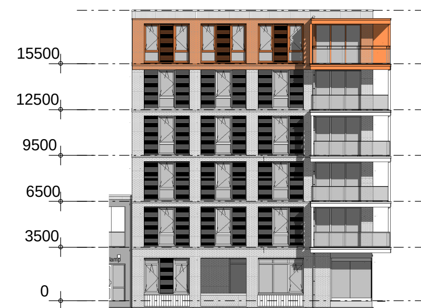
Linker zijgevel
