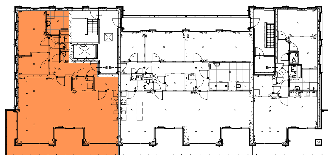
5e Verdieping
