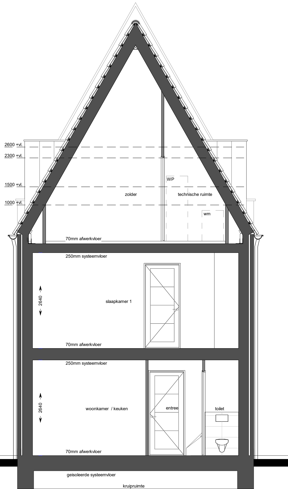
doorsnede woning
