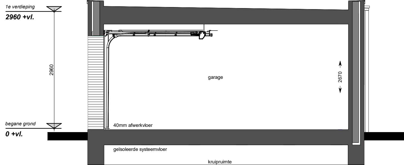
doorsnede garage
