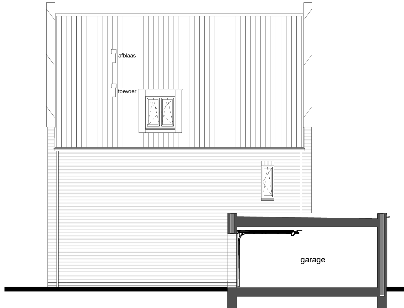
rechtergevel
