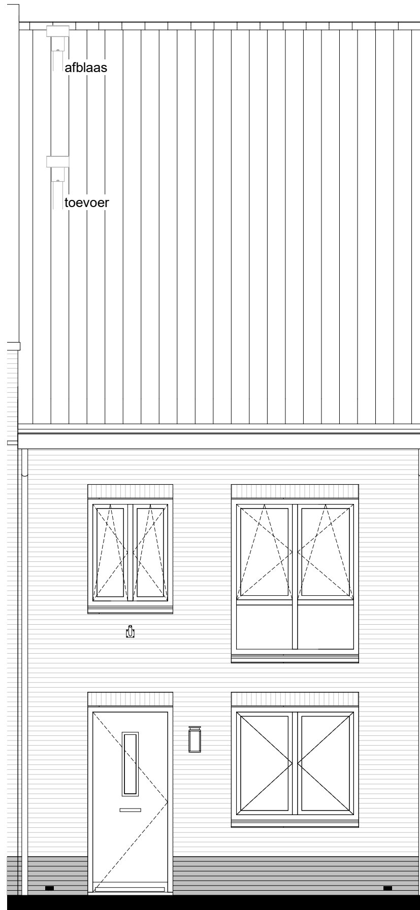
voorgevel
