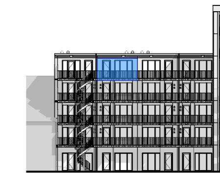
binnengevel (Zuid-Oost)
