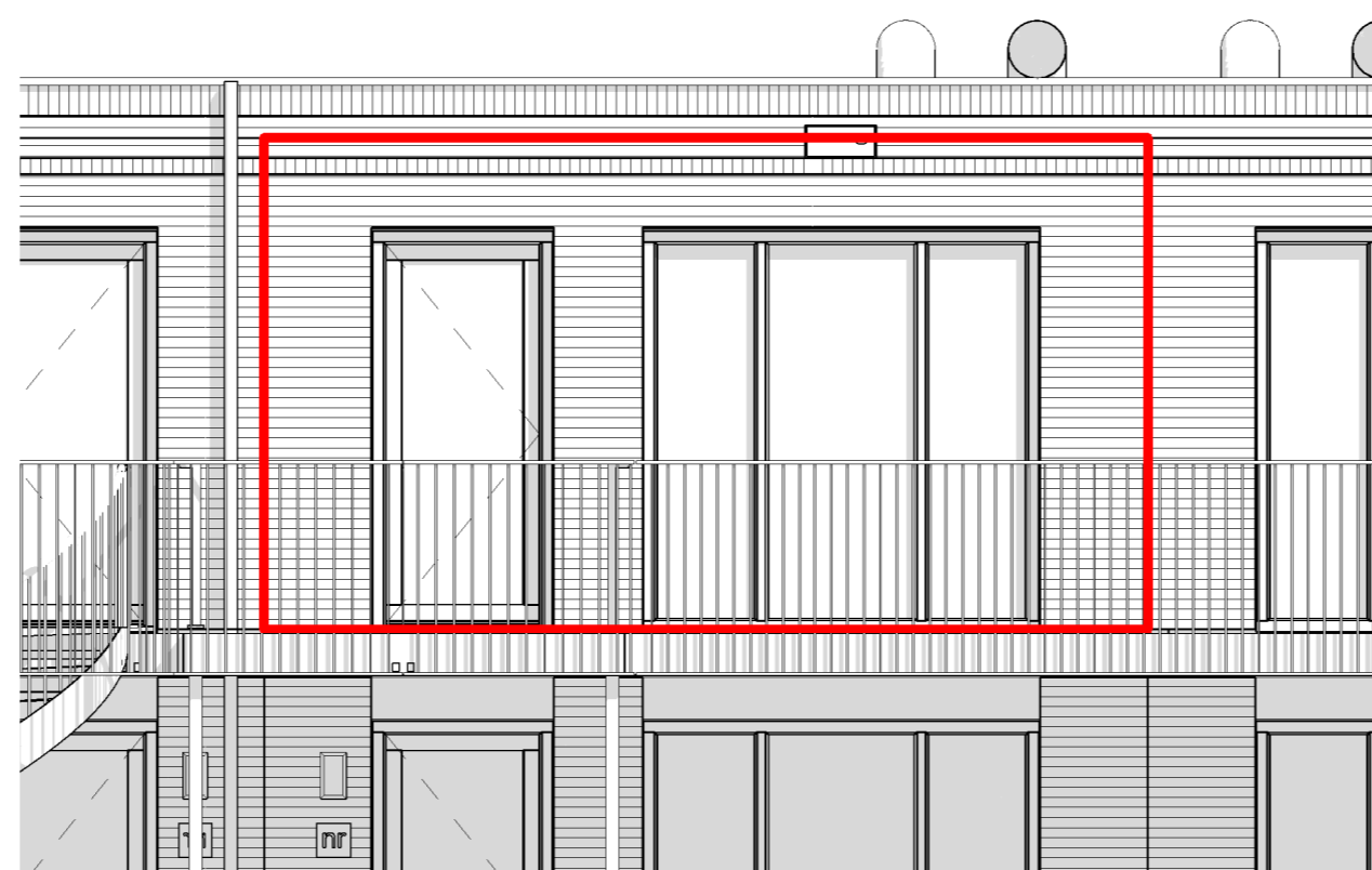
binnengevel (Zuid-Oost)
