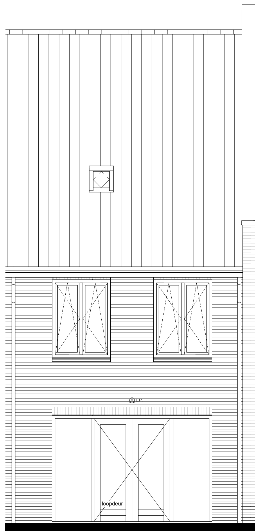
achtergevel
