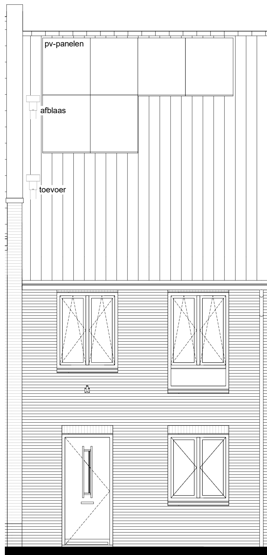
voorgevel
