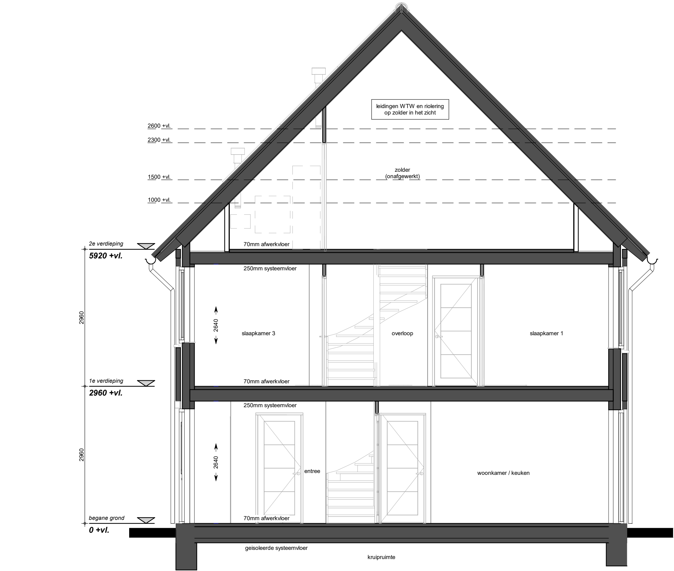
doorsnede
