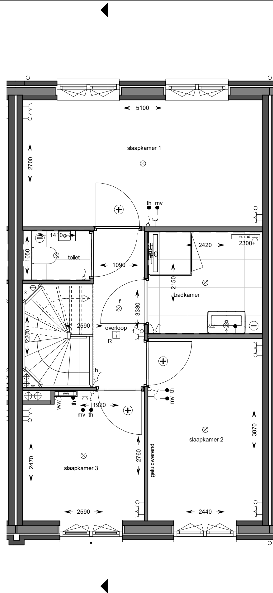
eerste verdieping
