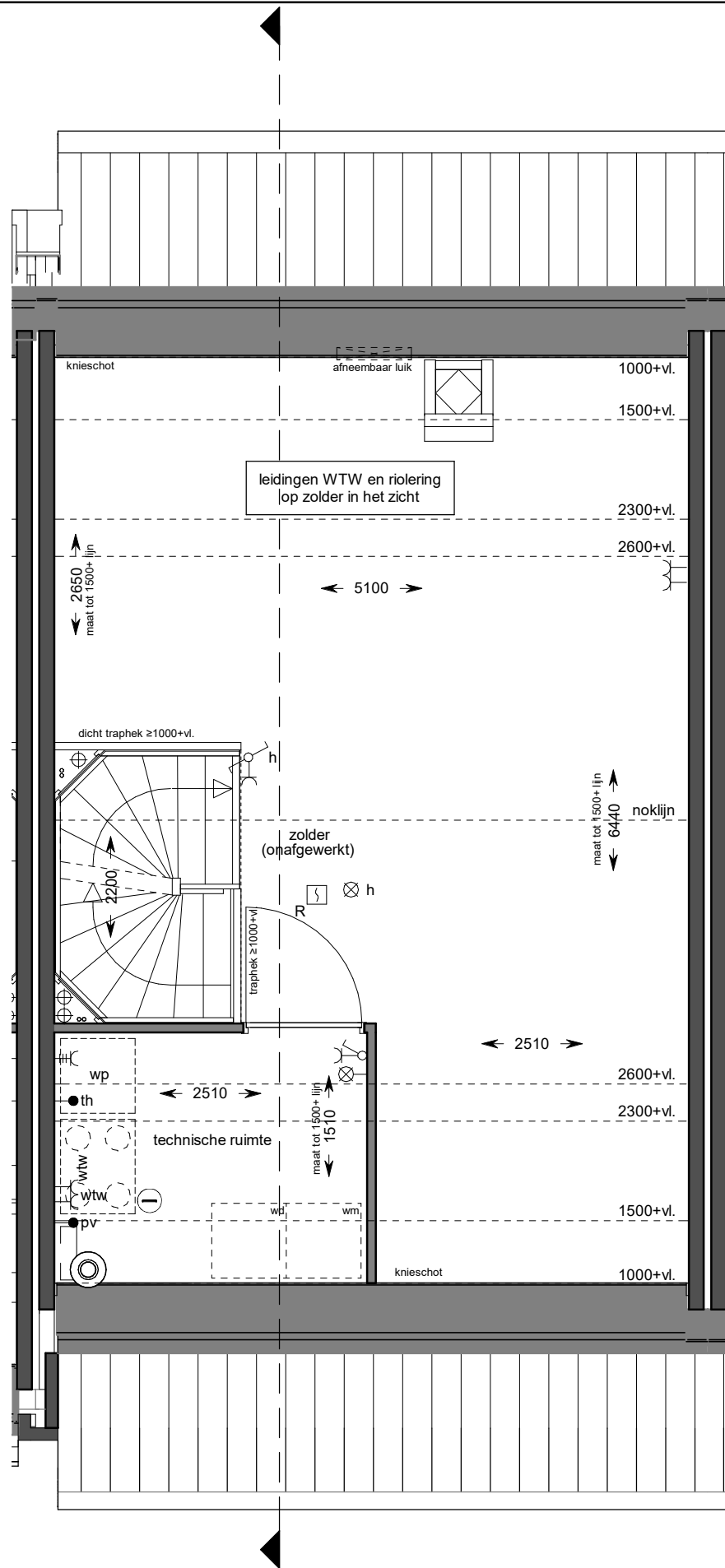
tweede verdieping
