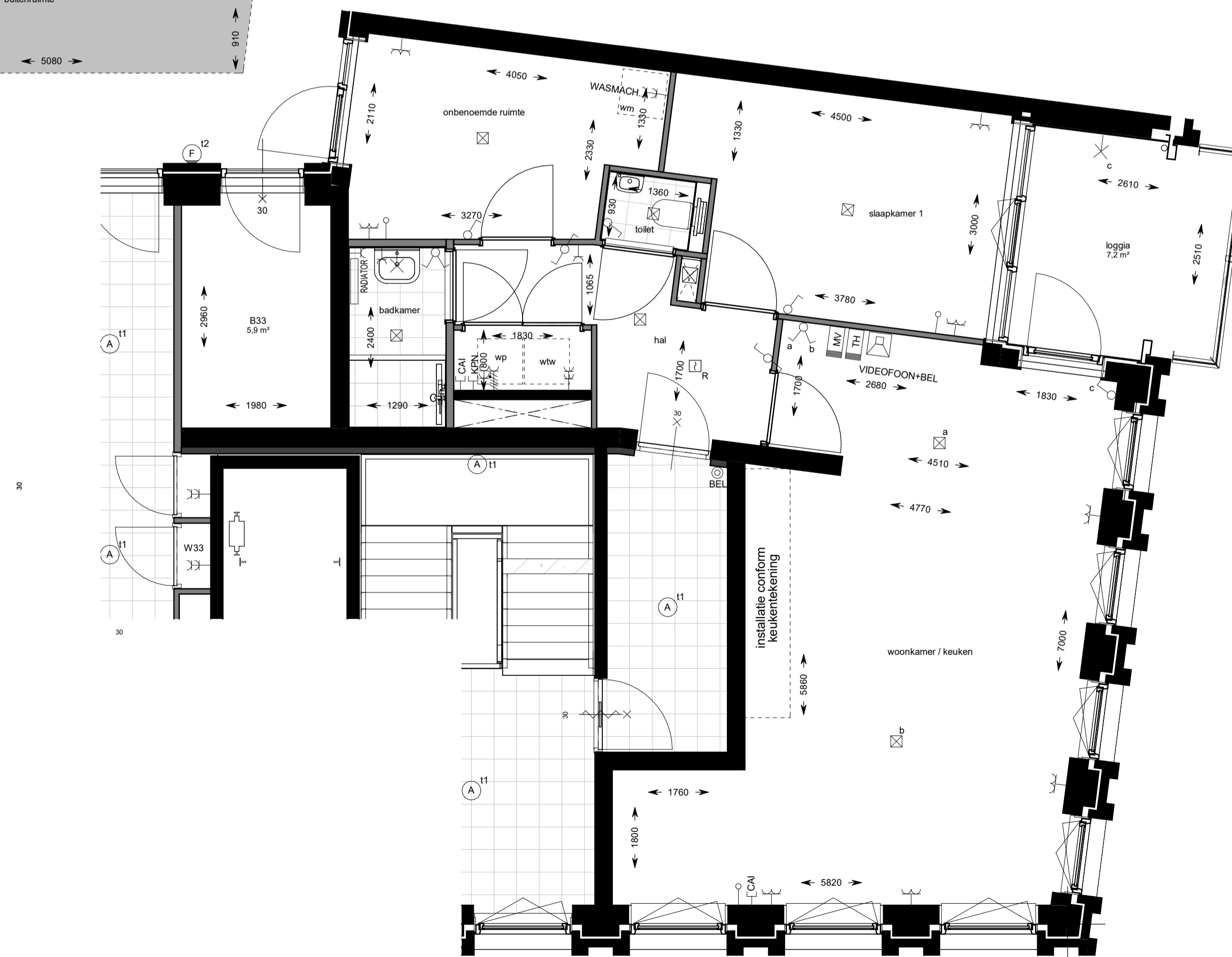
derde verdieping
