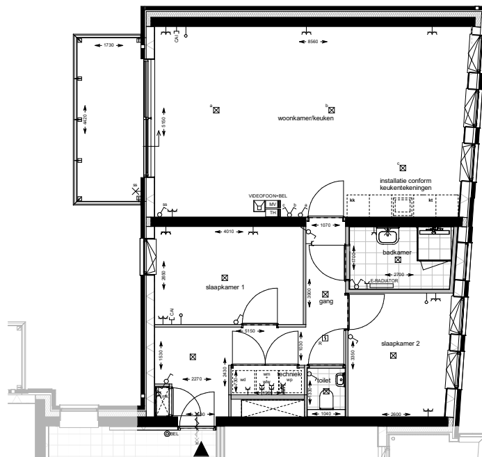
tweede verdieping 1 : 50
