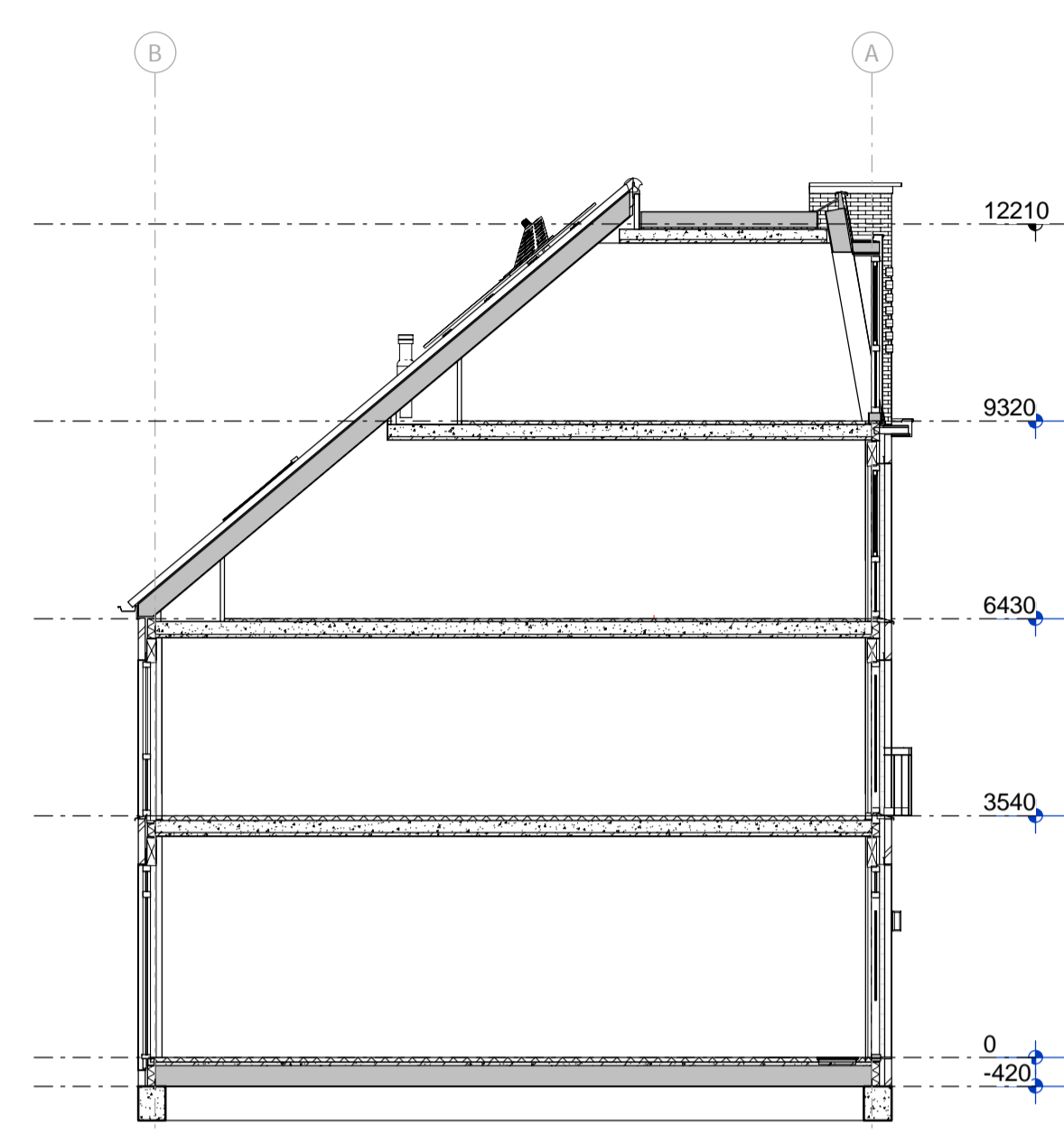
Doorsnede principe
