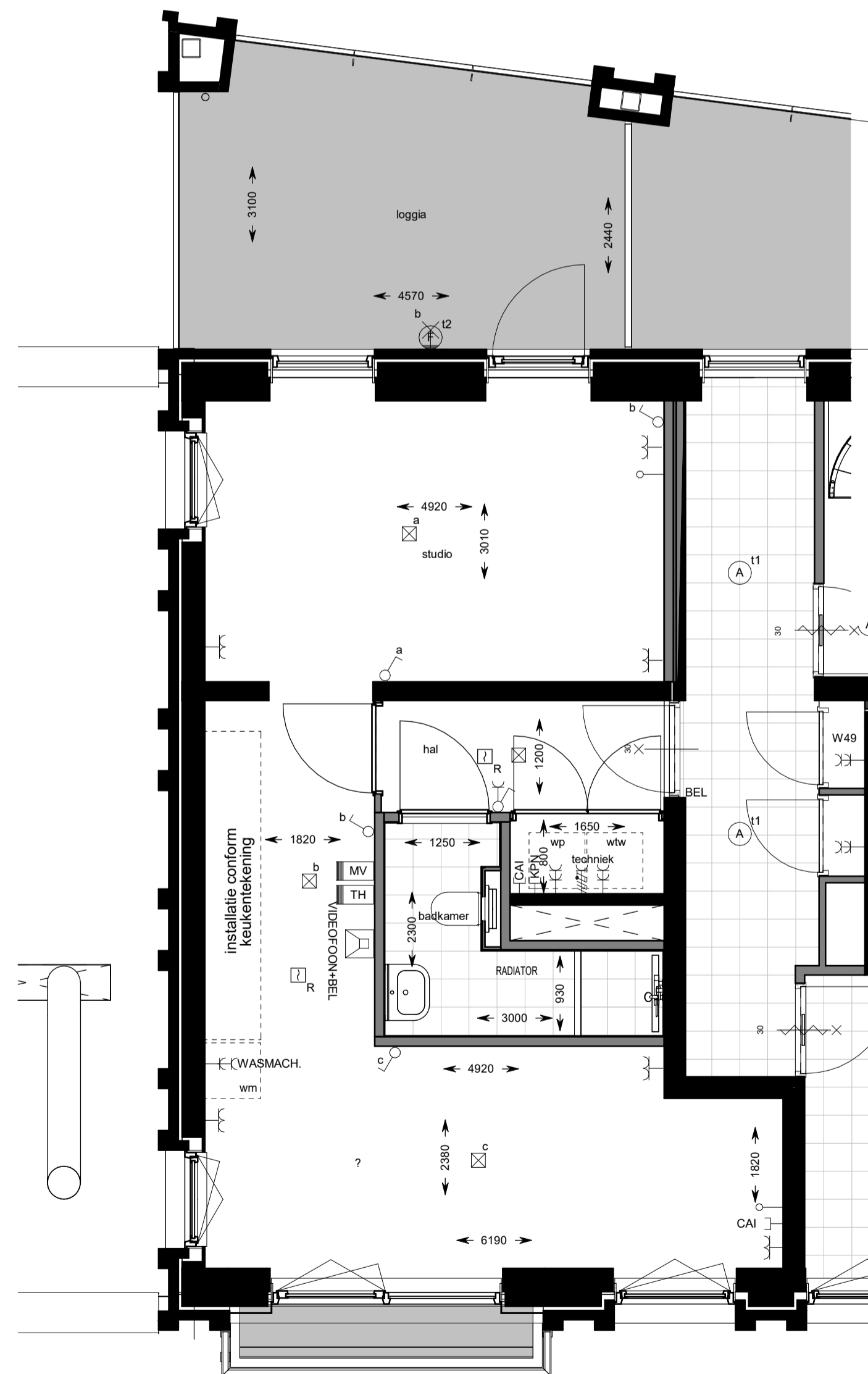
vijfde verdieping
