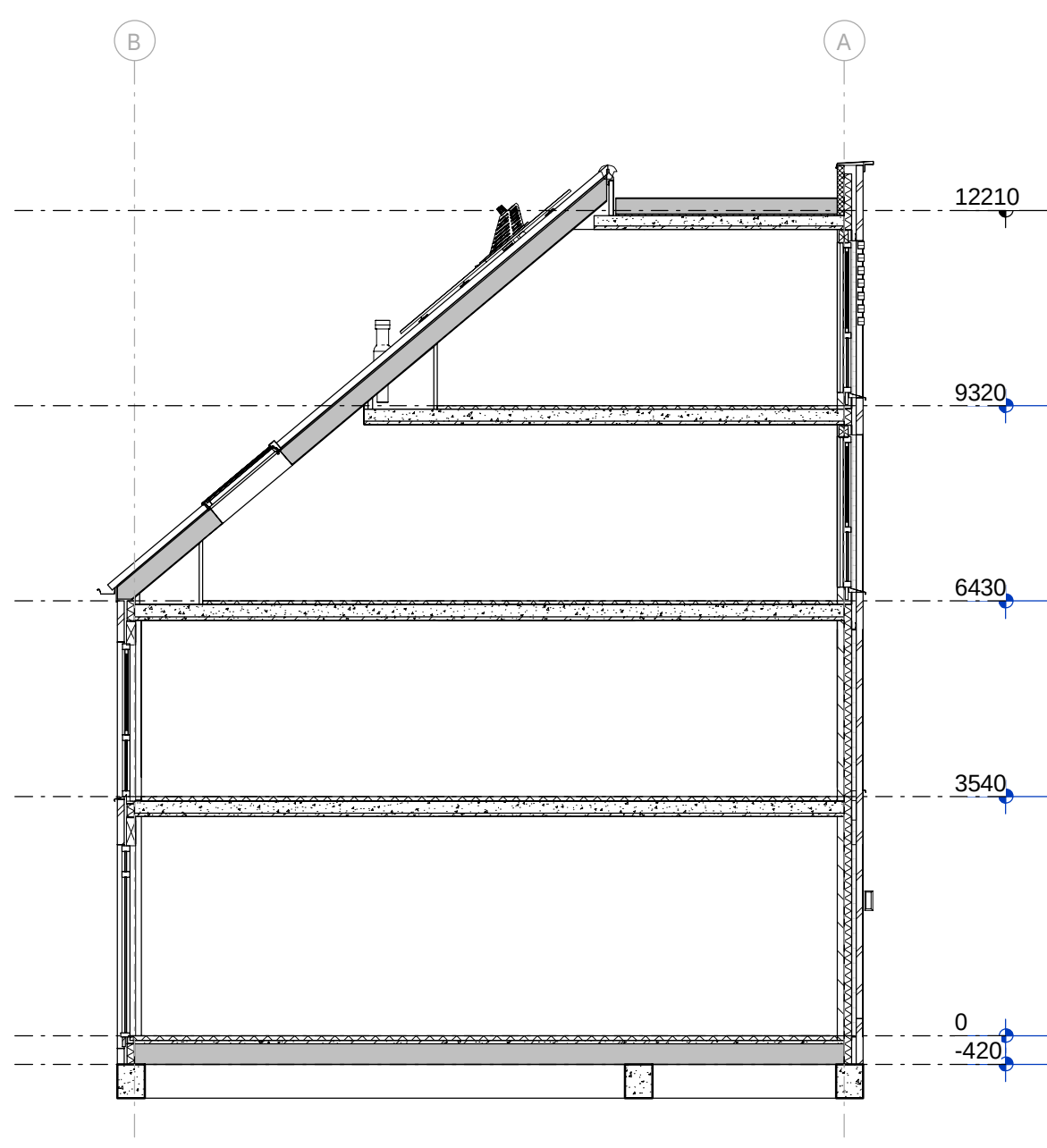
Doorsnede principe
