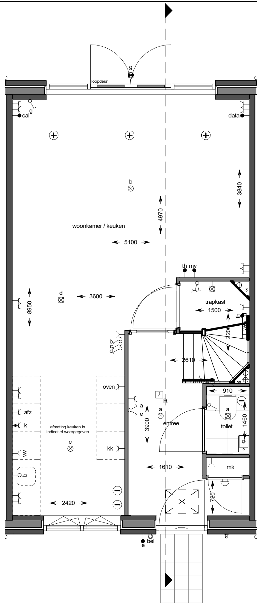
begane grond
