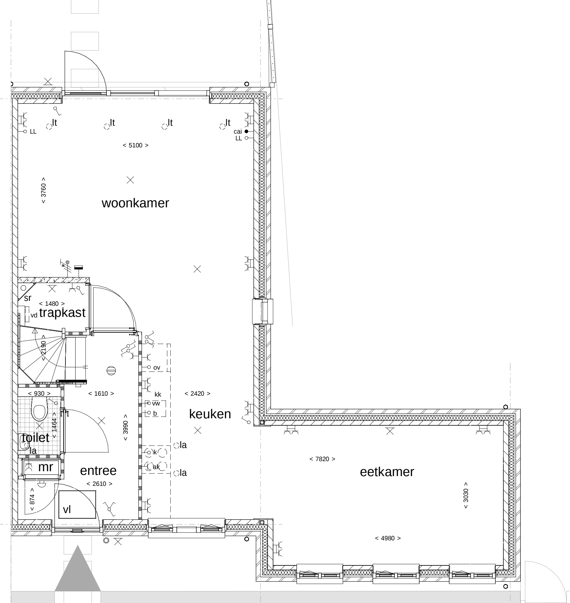
begane grond
