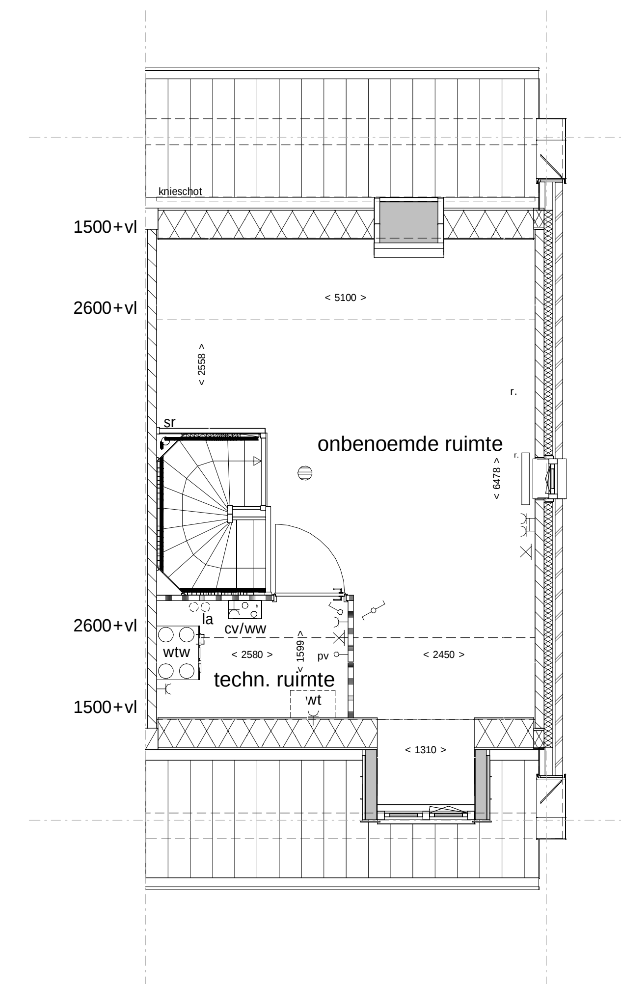
2e verdieping
