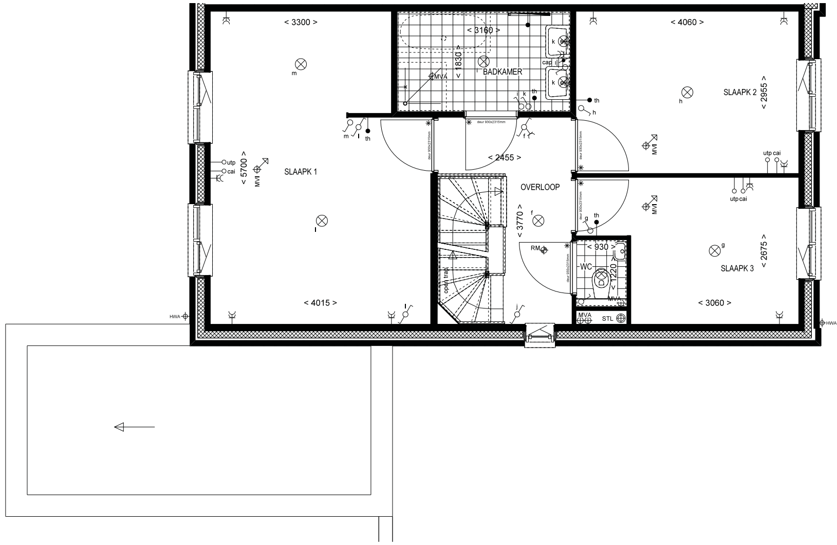
1e VERDIEPING BNR 5 TYPE D1
