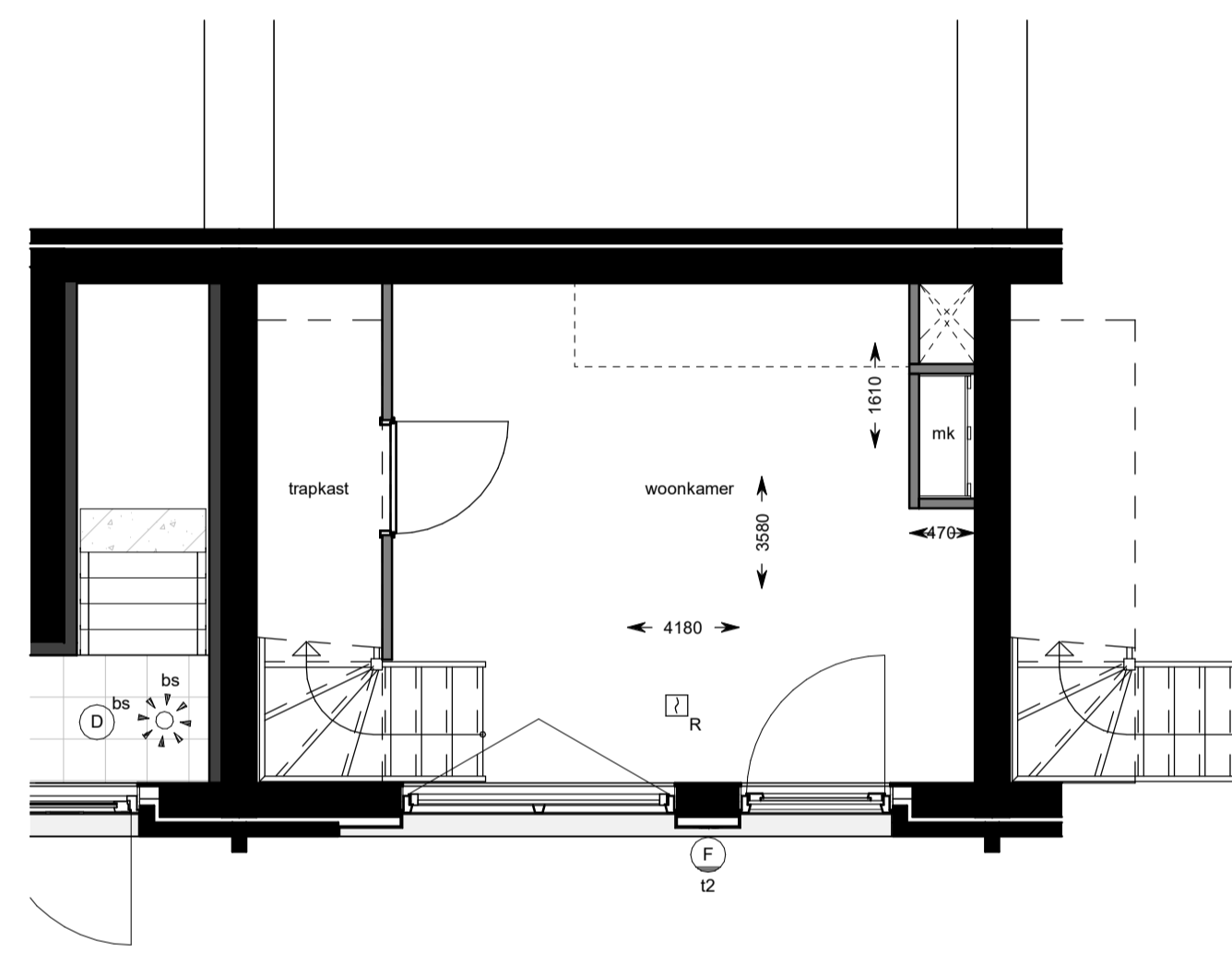
begane grond
