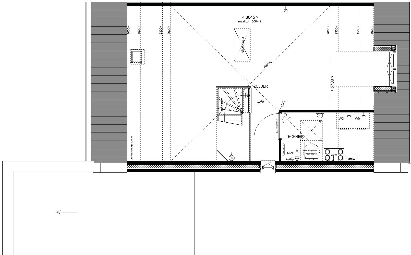
2e VERDIEPING BNR 15 TYPE D2
