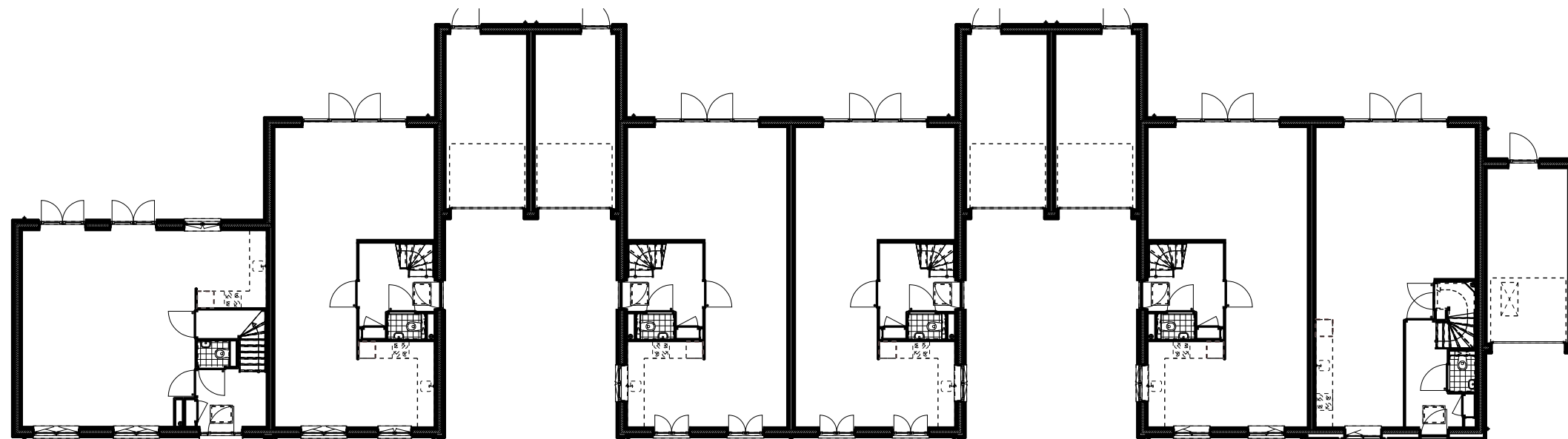
BNR 19 TYPE F1 BNR 18 TYPE D3 BNR 17 TYPE D2 BNR 16 TYPE D2sp BNR 15 TYPE D1 BNR 14 TYPE C1 BEGANEGROND
