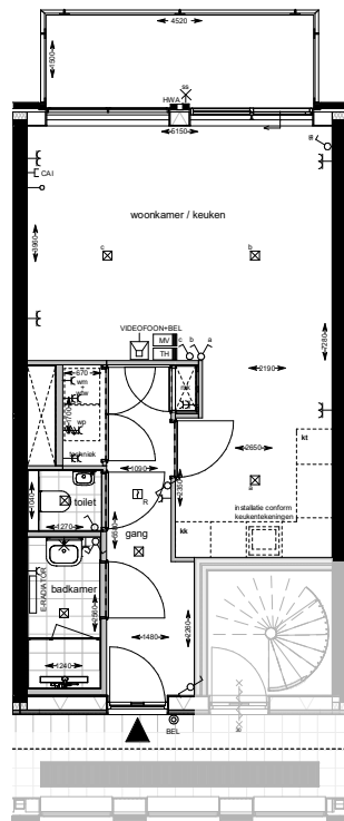
plattegrond 1 : 50
