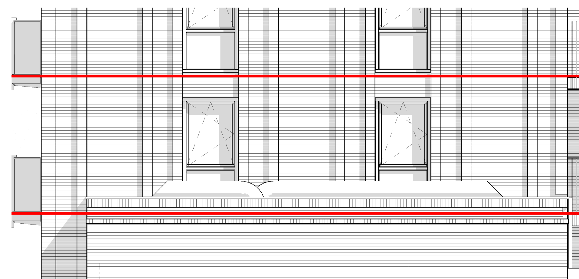
binnengevel (Zuid)
