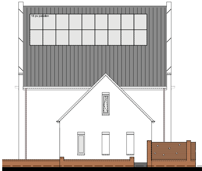
ZIJGEVEL
