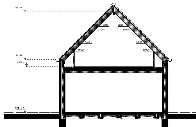
DOORSNEDE
