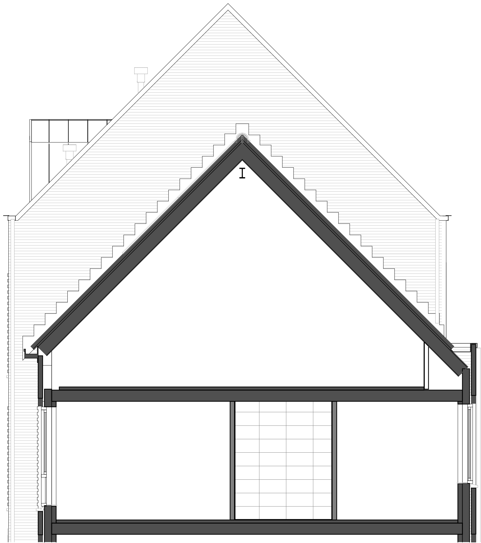
zijgevel
