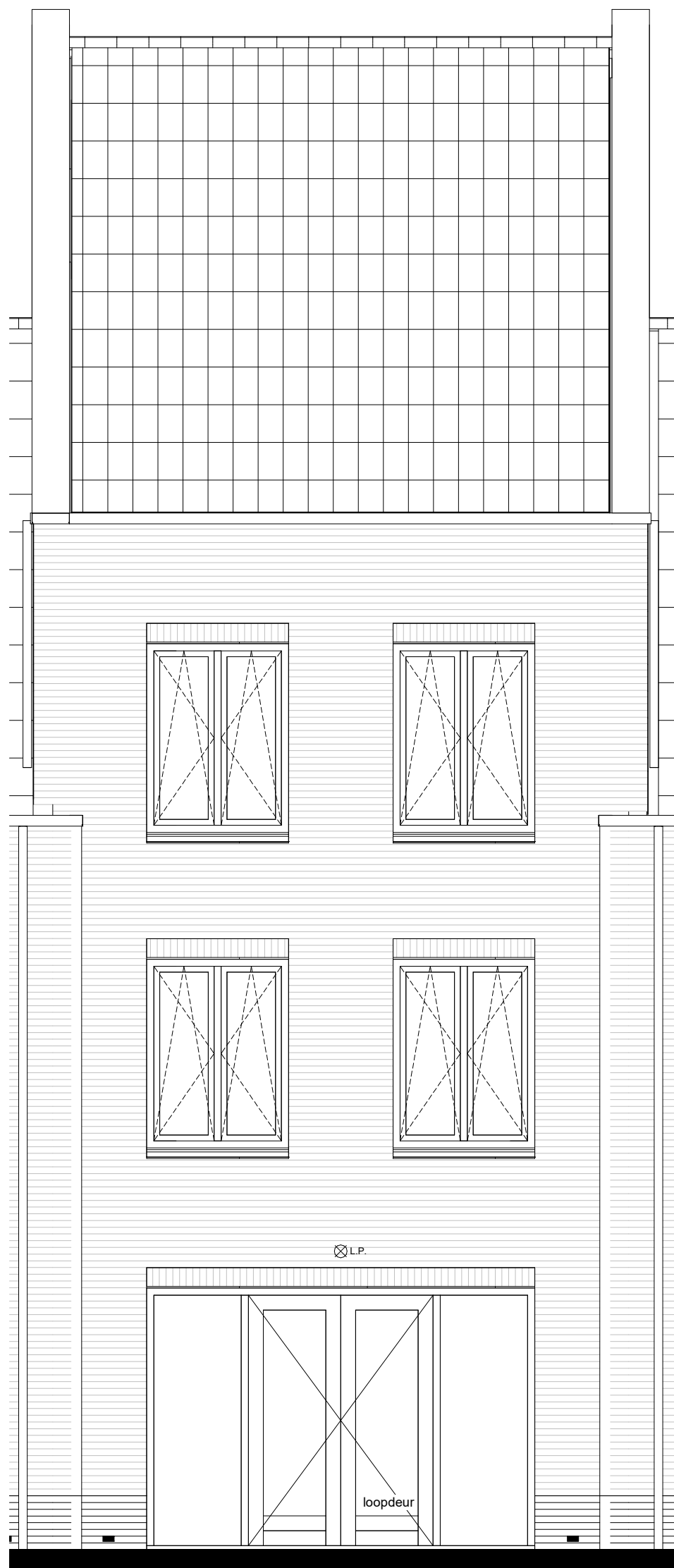
achtergevel
