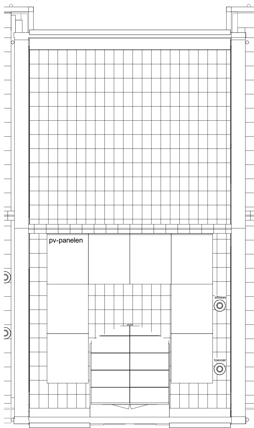
dakaanzicht
