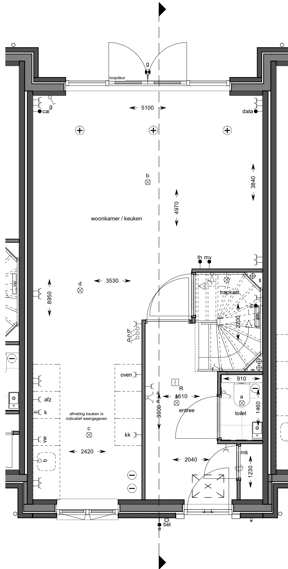
begane grond
