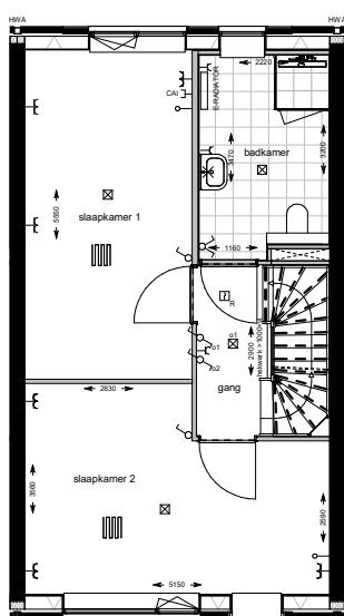
eerste verdieping 1 : 50
