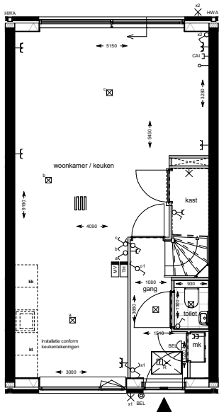
begane grond 1 : 50
