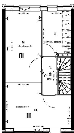
tweede verdieping 1 : 50
