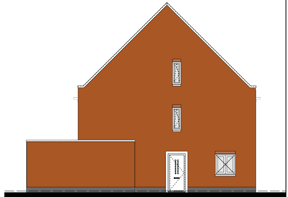
ZIJGEVEL
