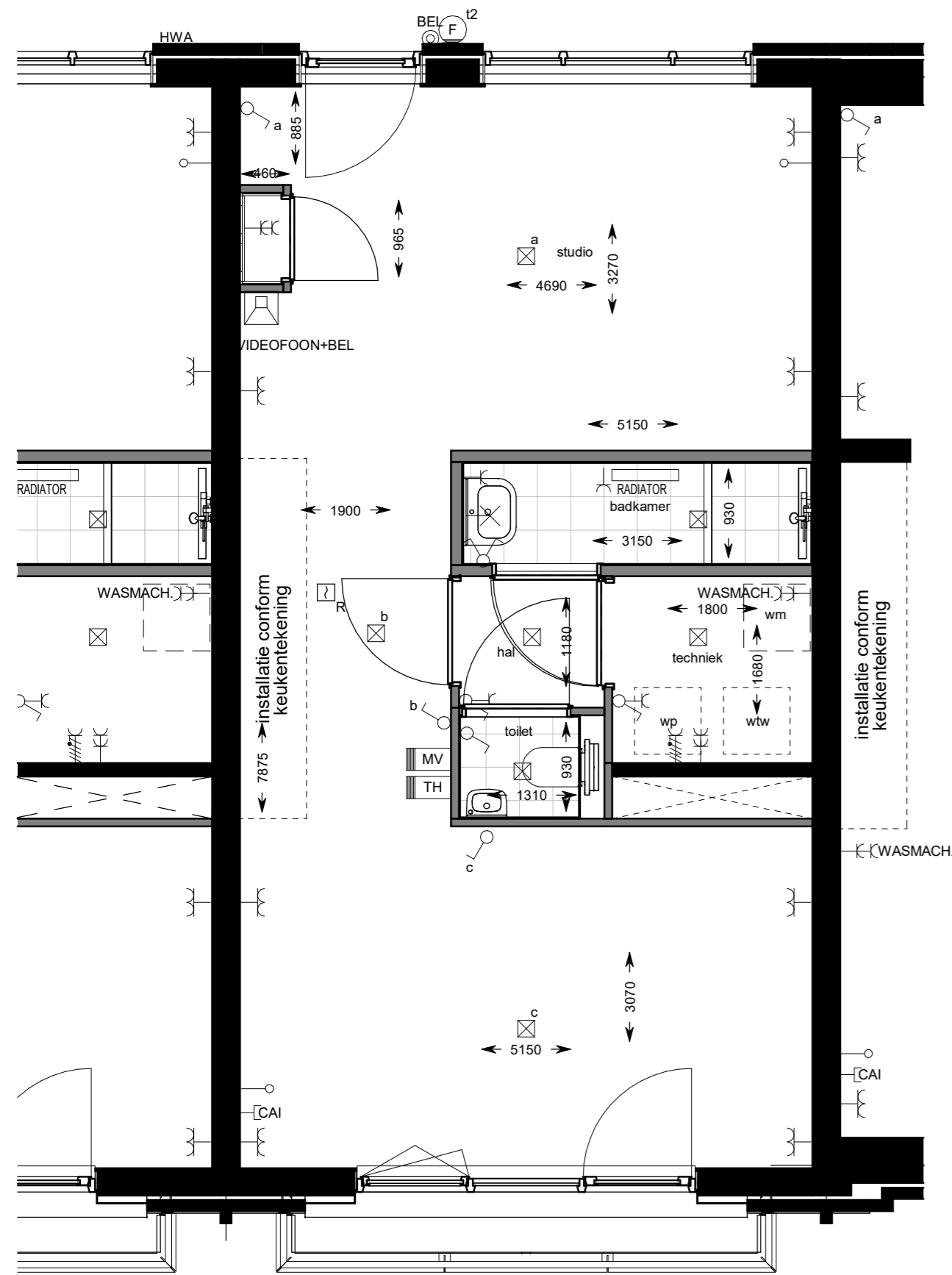
tweede verdieping
