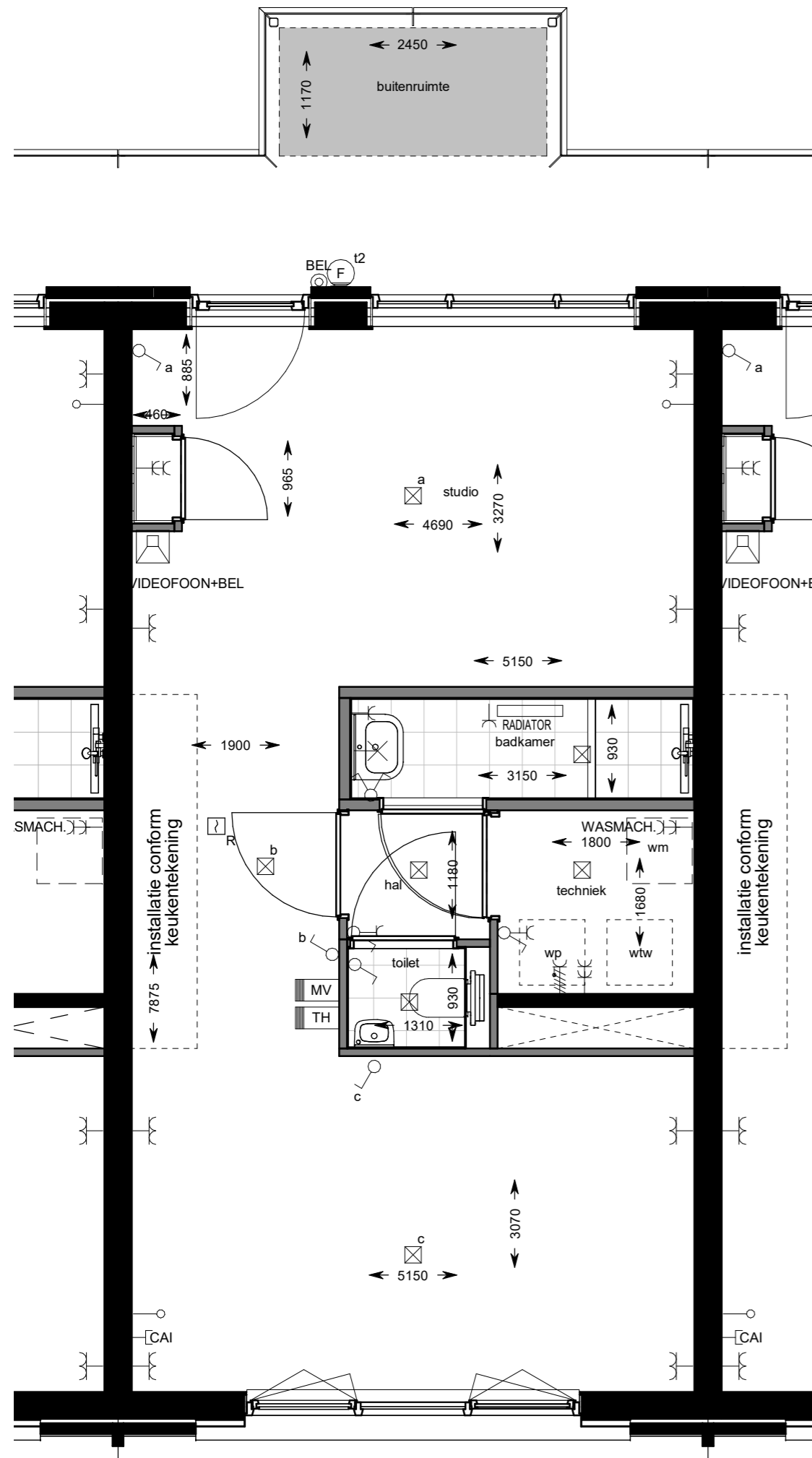
derde verdieping
