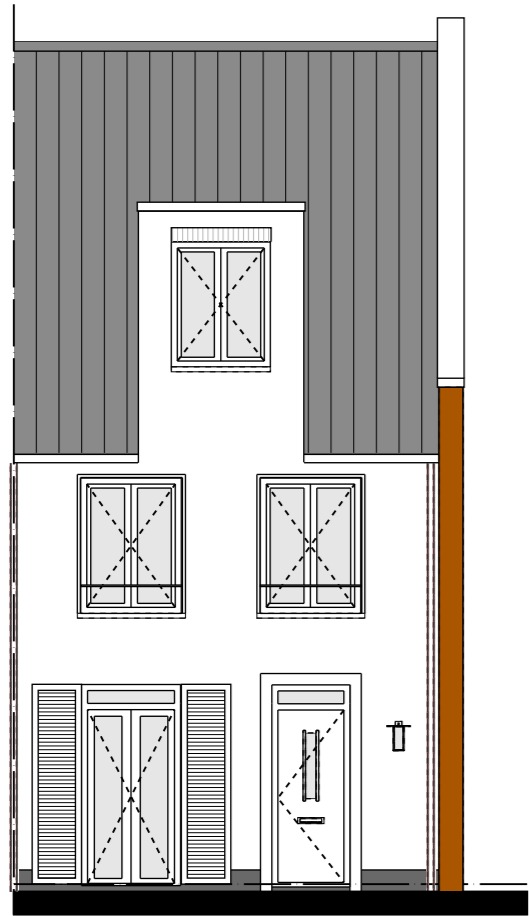
VOORGEVEL
