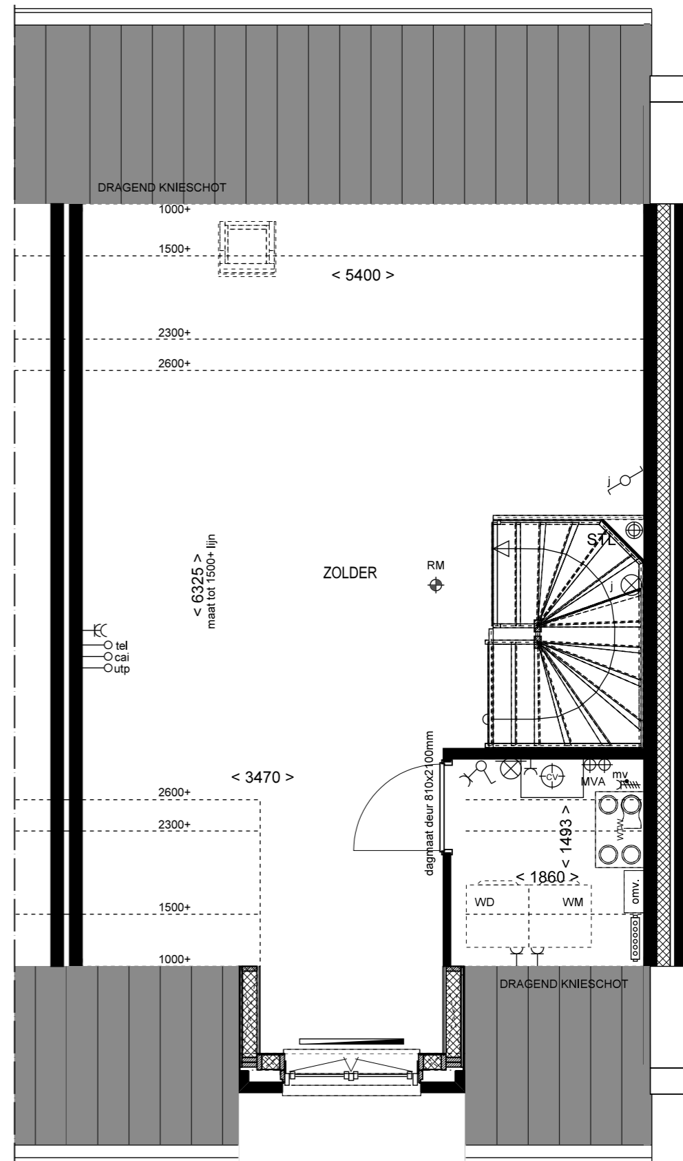
2e VERDIEPING
