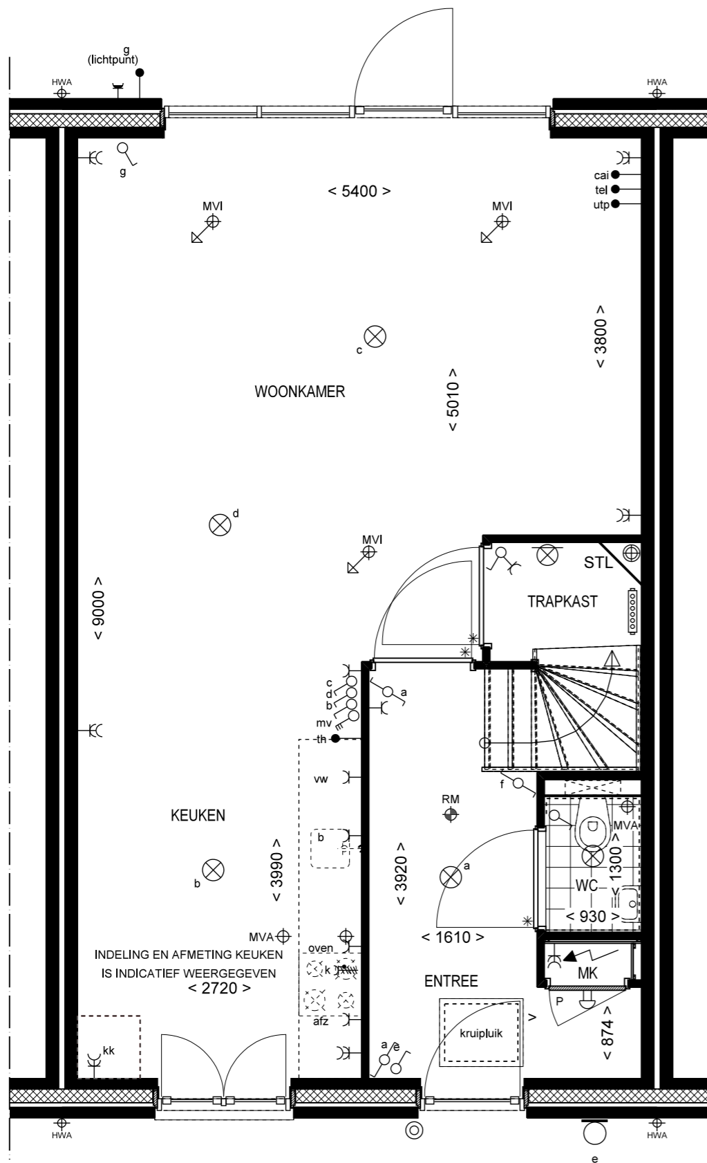
BEGANE GROND
