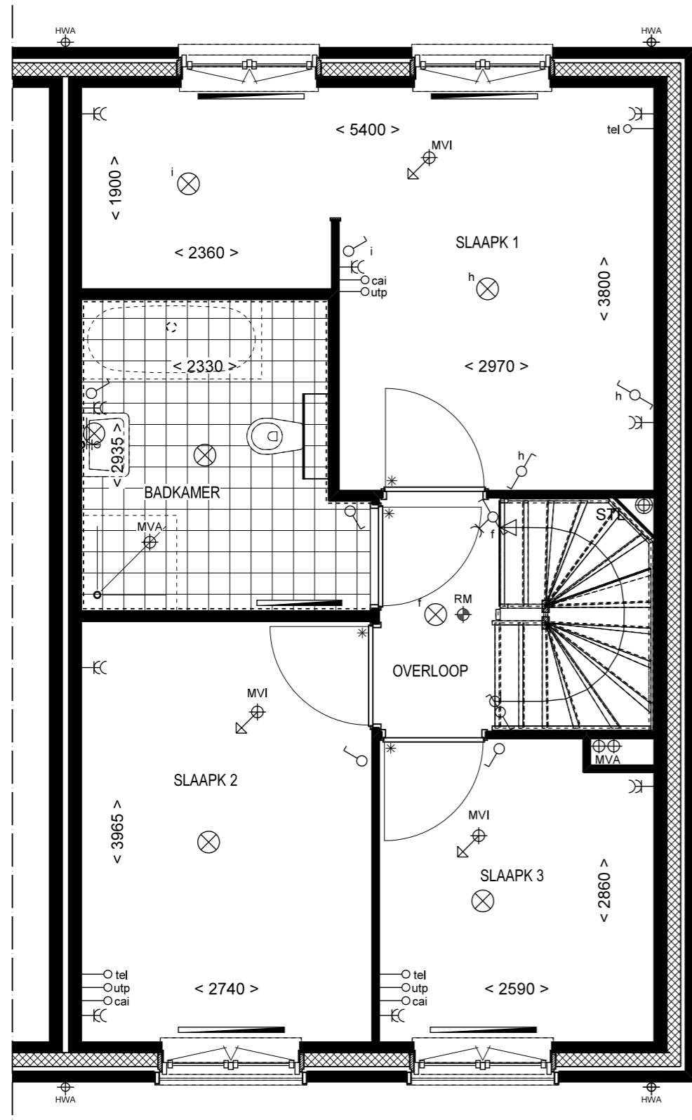
1e VERDIEPING
