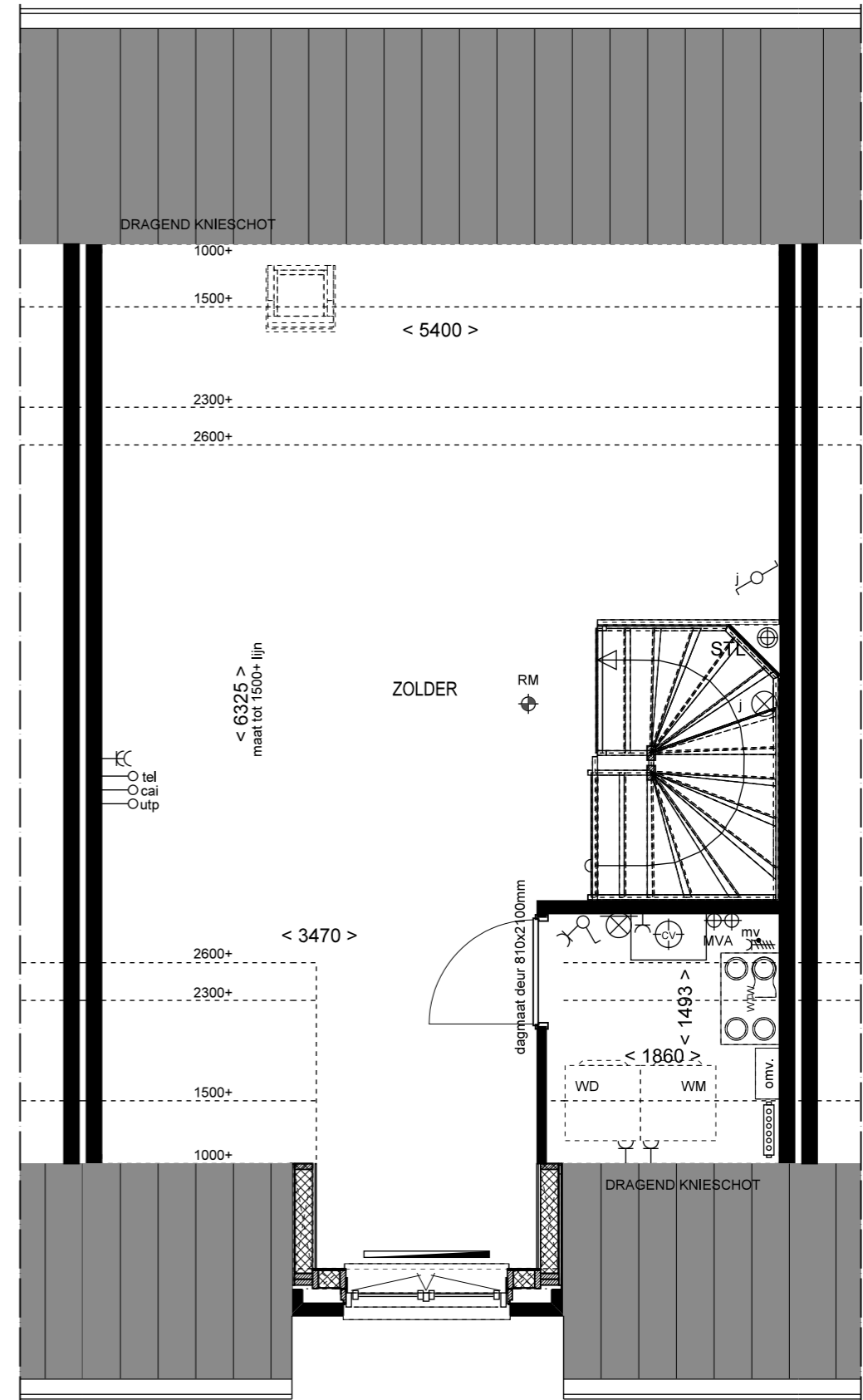
2e VERDIEPING
