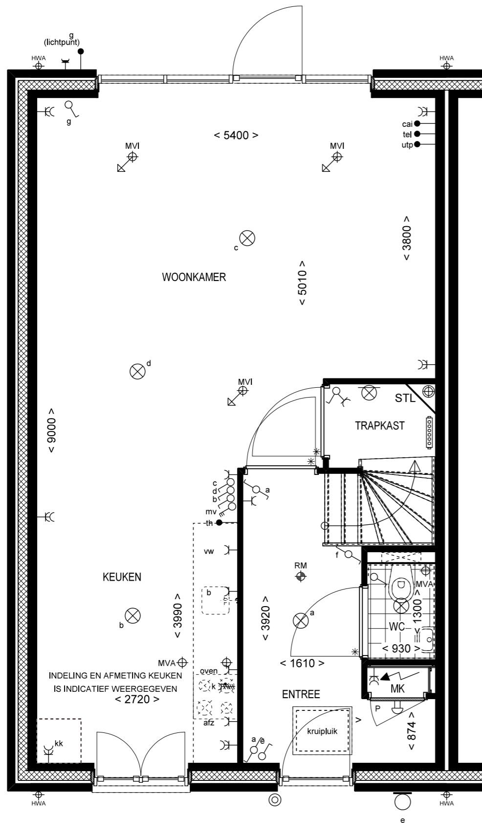
BEGANE GROND
