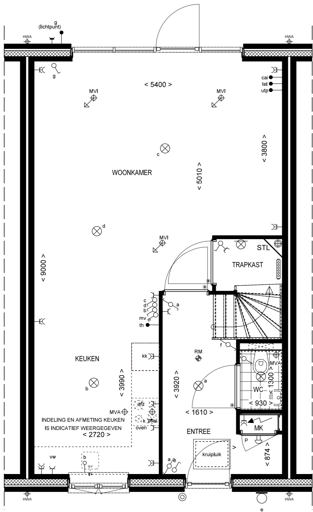
BEGANE GROND
