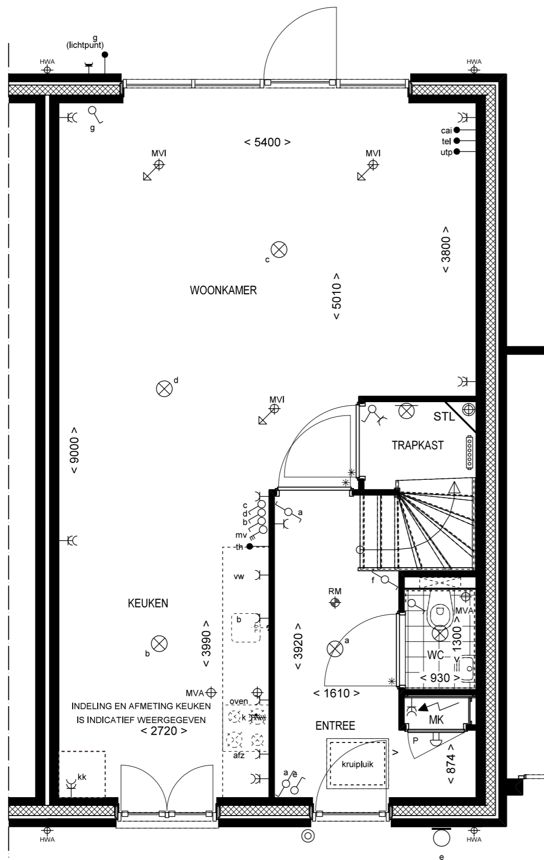
BEGANE GROND
