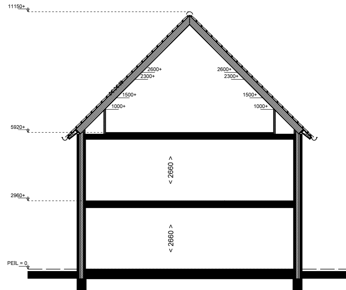
DOORSNEDE
