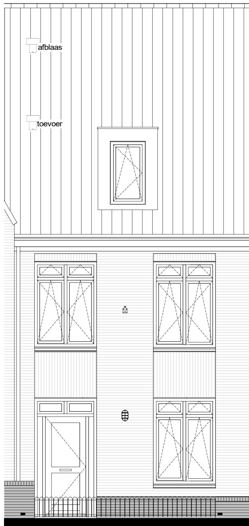
voorgevel
