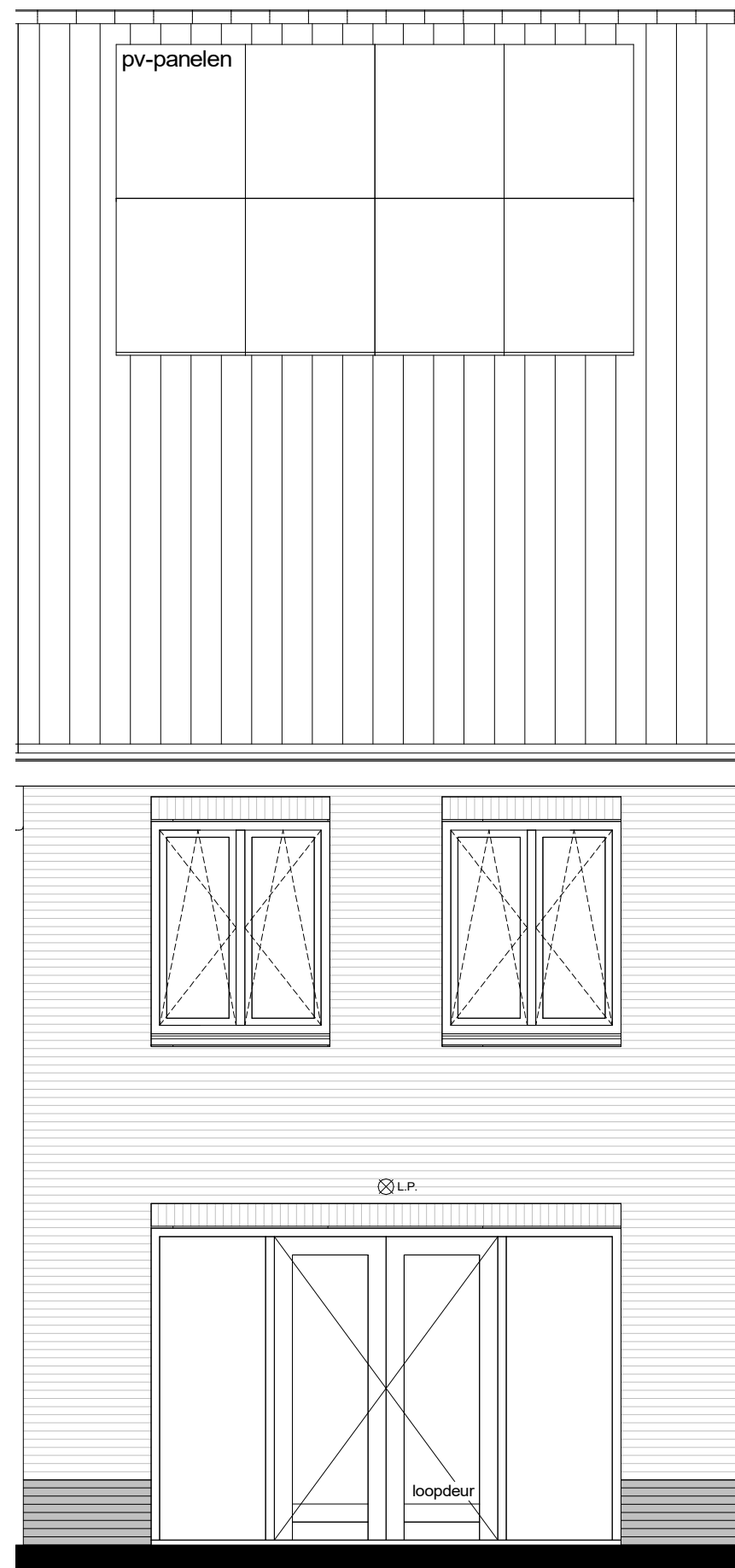
achtergevel
