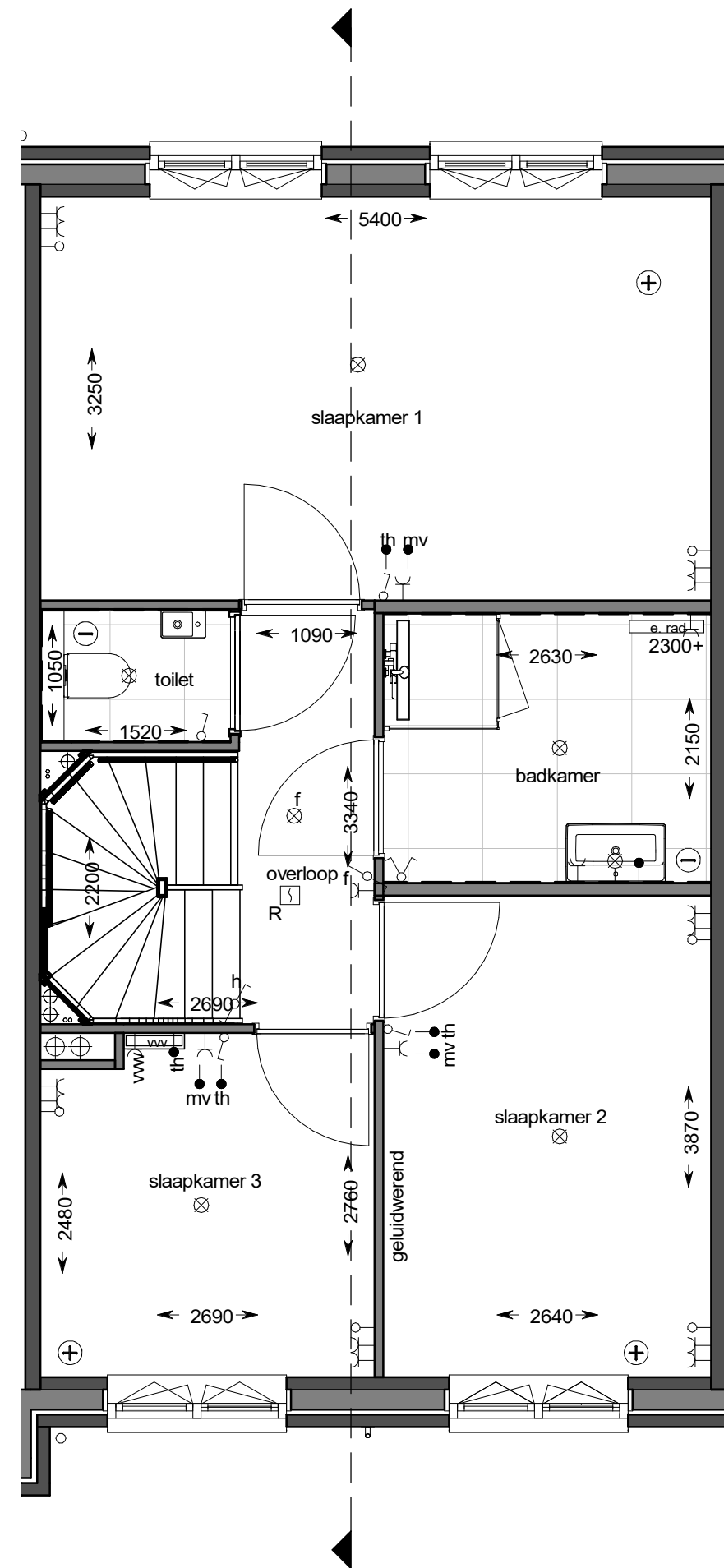
eerste verdieping
