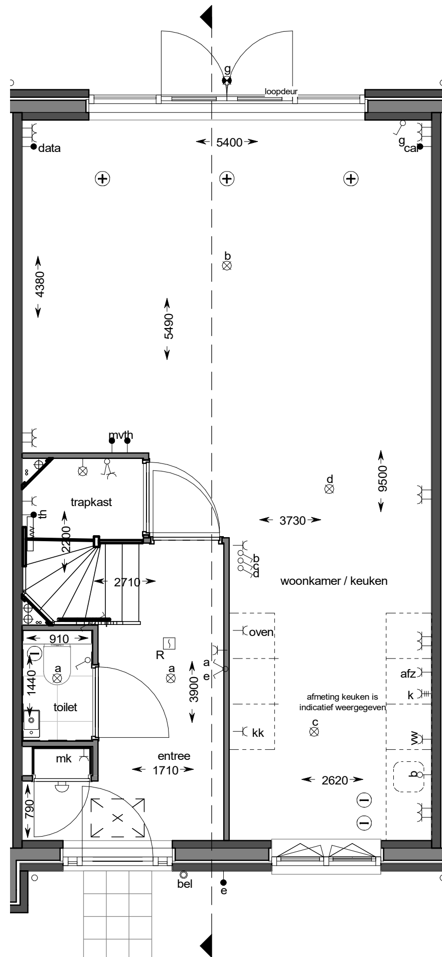
begane grond
