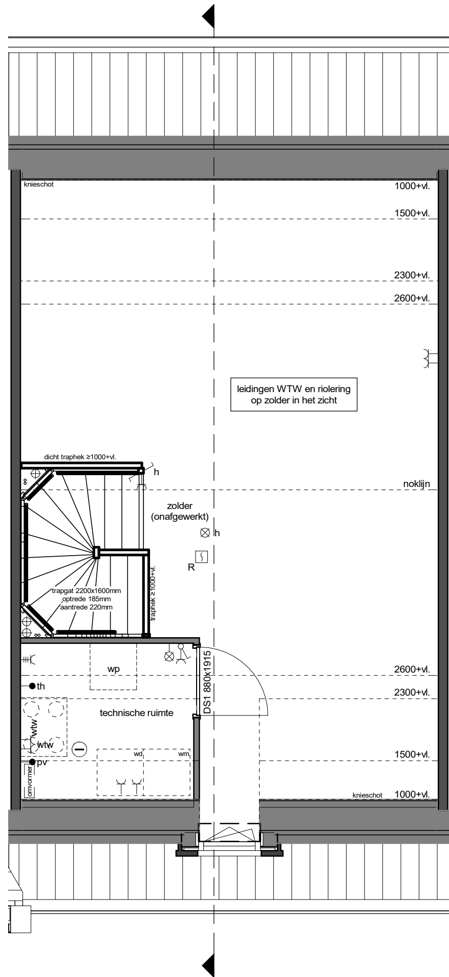
tweede verdieping
