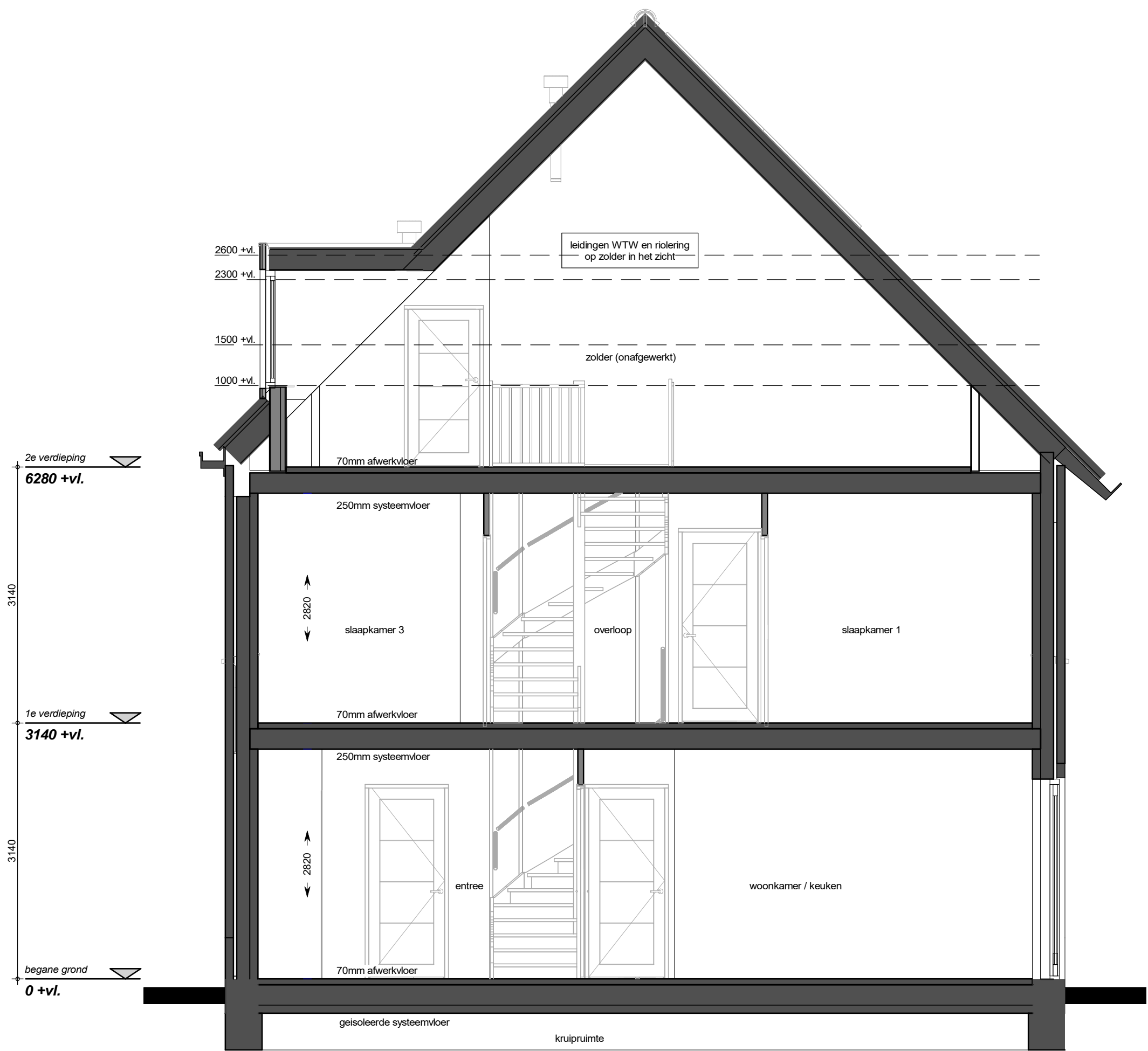
doorsnede
