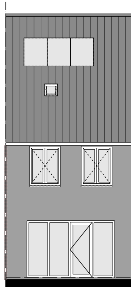
ACHTERGEVEL
