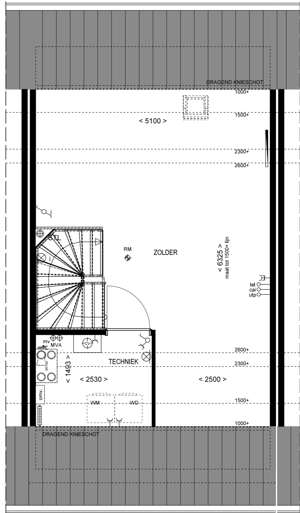
2e VERDIEPING
