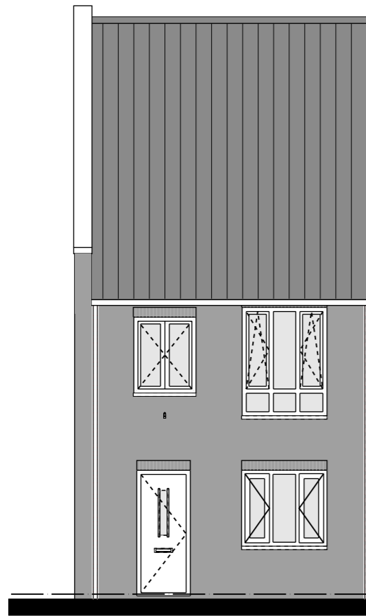
VOORGEVEL
