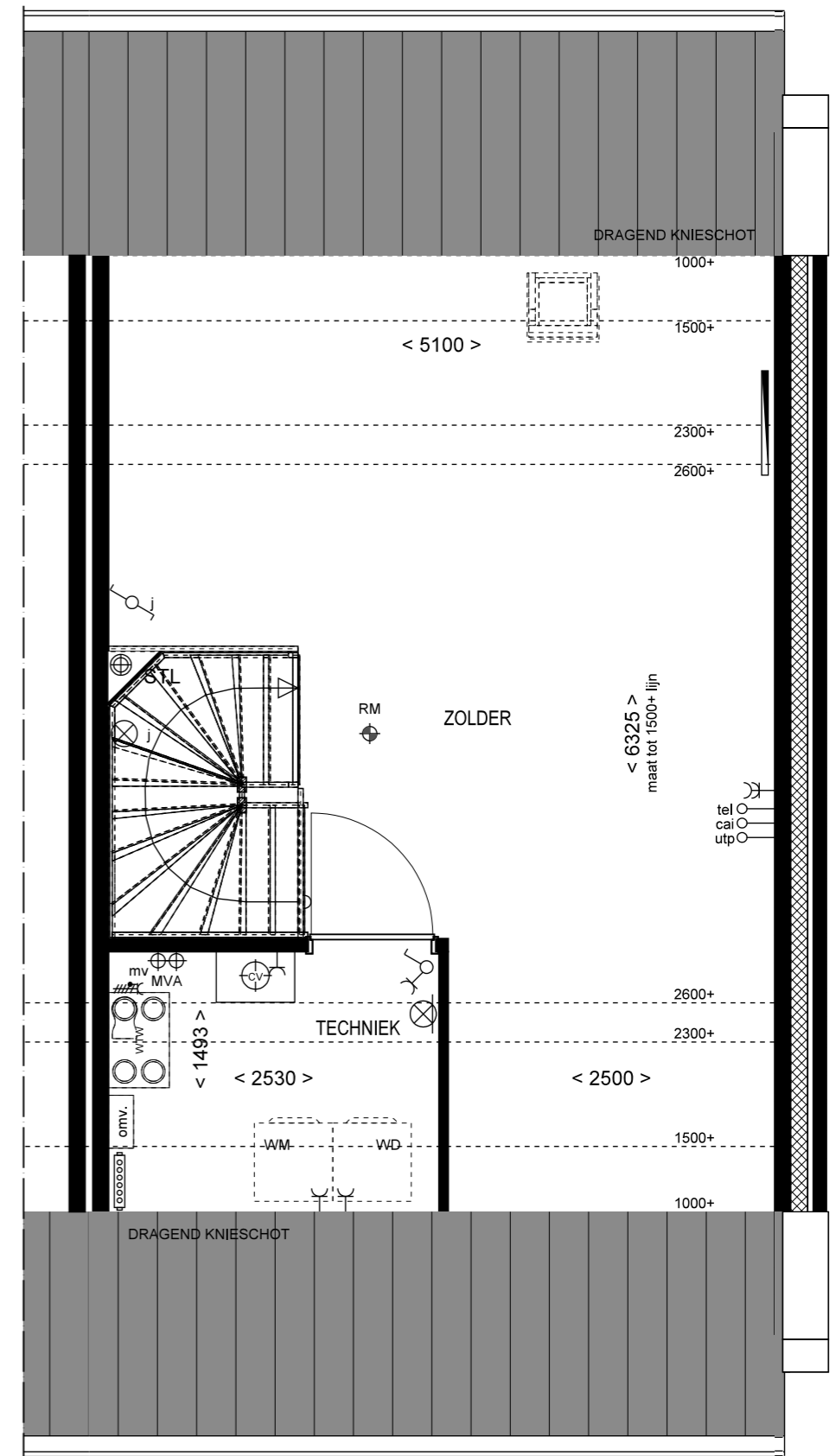
2e VERDIEPING
