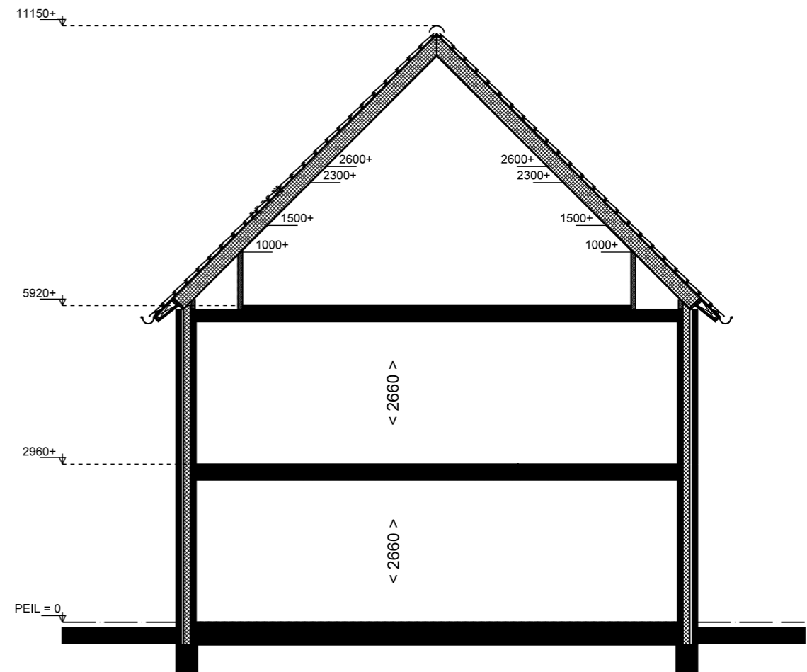
DOORSNEDE
