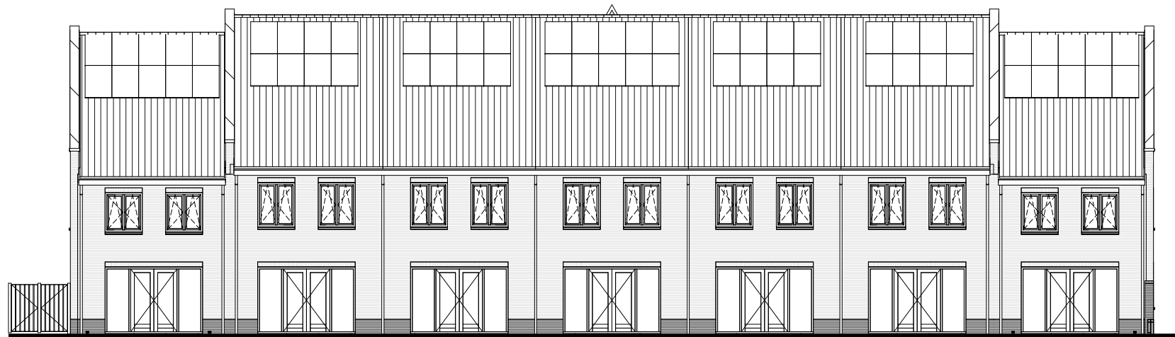
achtergevel
