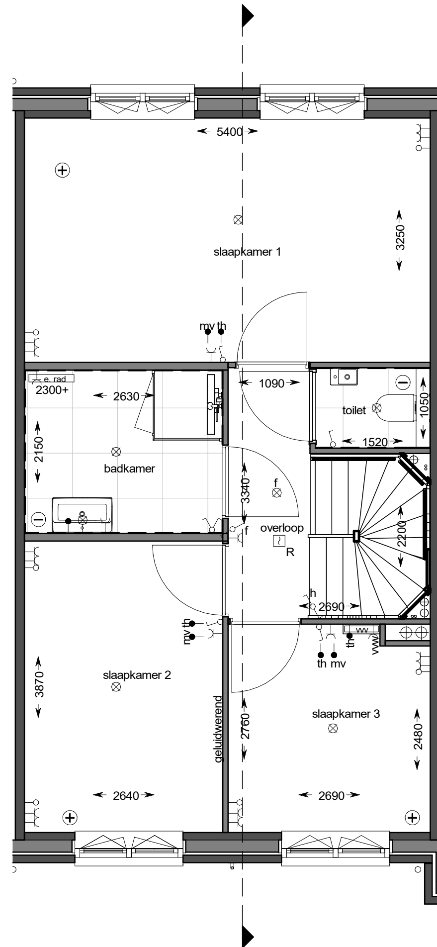
eerste verdieping
