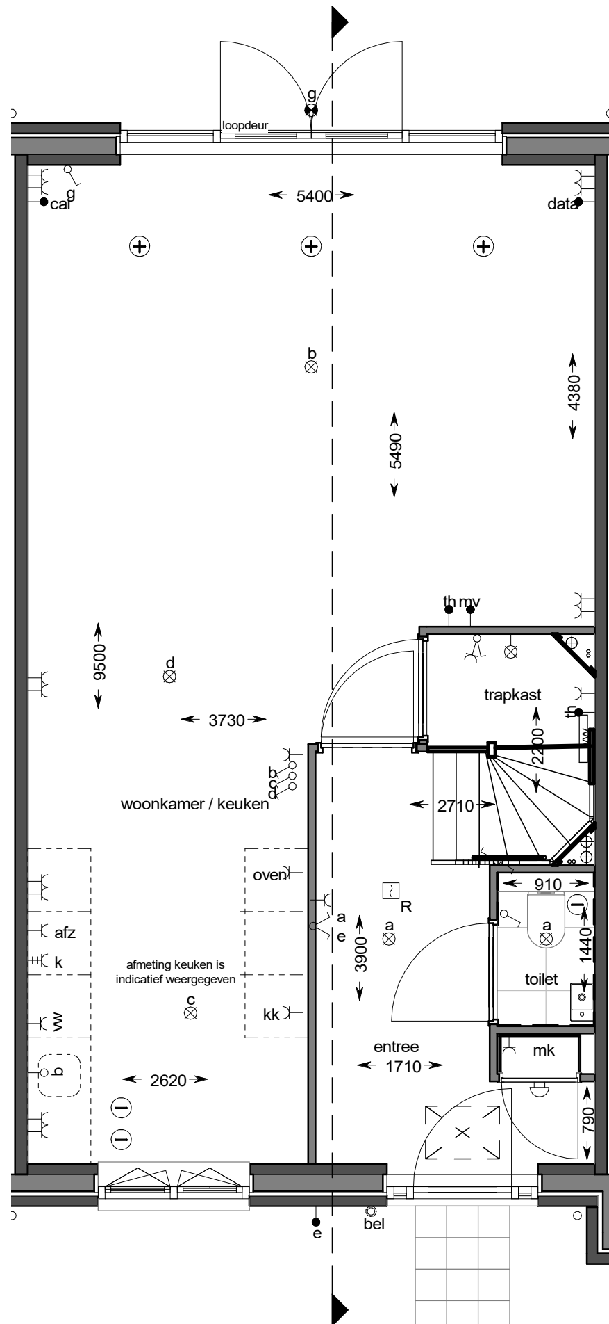
begane grond
